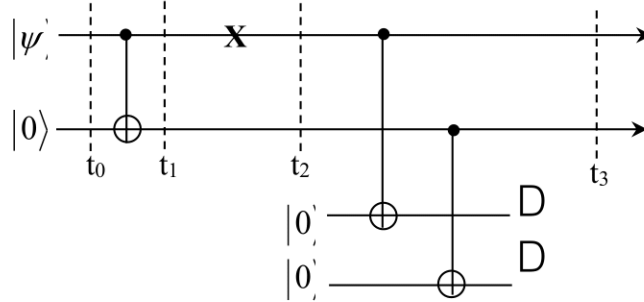
Figure C2 : Circuit quantique du code correcteur à deux qubits. Le symbole D désigne la détection de l'erreur sur qubit 1 par la mesure des deux qubits rajoutés.
