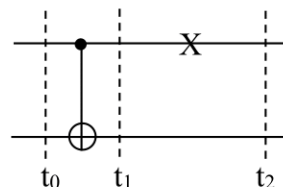
Figure C1 : Circuit quantique du code correcteur à deux qubits.
