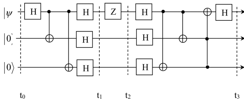
Figure D2 : Circuit du code à trois qubits pour la correction d'une erreur de phase.
