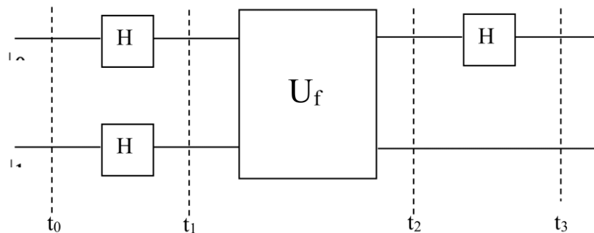
Figure A1 : Circuit quantique de l'algorithme de Deutsch.
