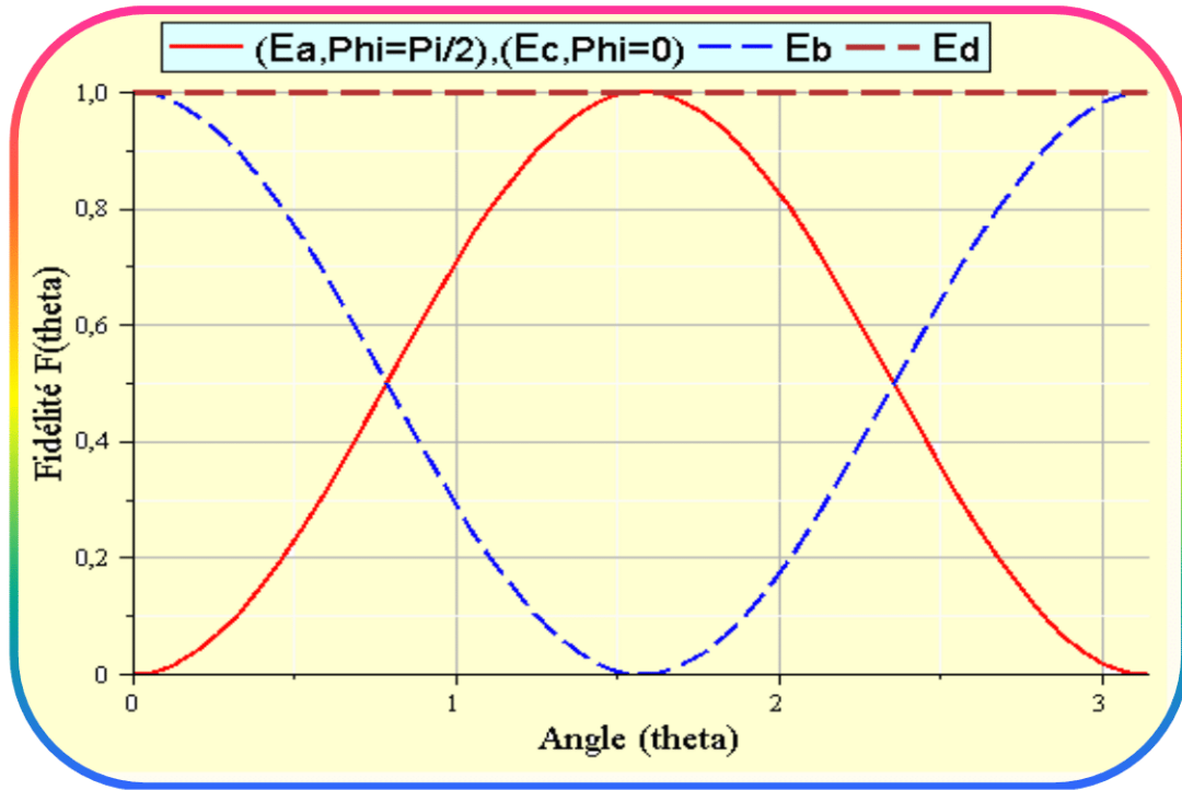
Figure 12 : Fidélité F(\theta, \phi) avec 0 \leq \theta \leq \pi , \phi = \pi/2 pour le groupe d'erreur \varepsilon_a et \phi = 0 pour le groupe d'erreur \varepsilon_c . On note que pour le groupe d'erreur \varepsilon_d la fidélité est égale à 1 pour 0 \leq (\theta, \phi) \leq \pi .
