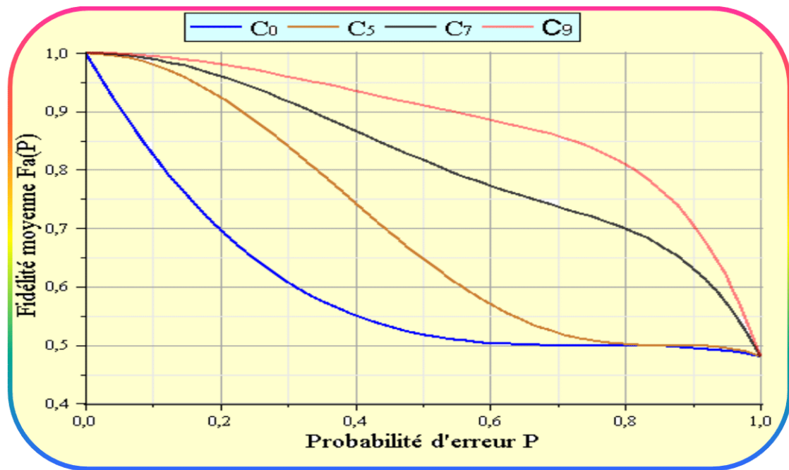
Figure 15 : Evolution de la fidélité moyenne avec la probabilité d'erreur de canal dépolarisant, sans et avec protection par trois codes.
