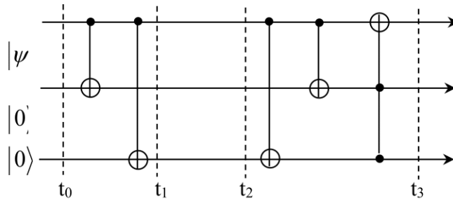
Figure D1: Circuit quantique du code correcteur à trois qubits.
