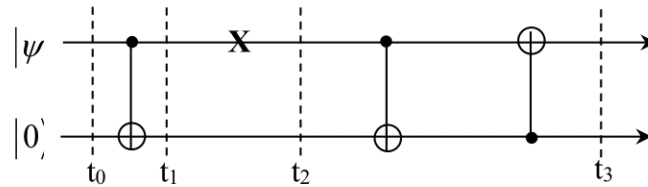
Figure C4 : Circuit quantique du code correcteur à deux qubits.
