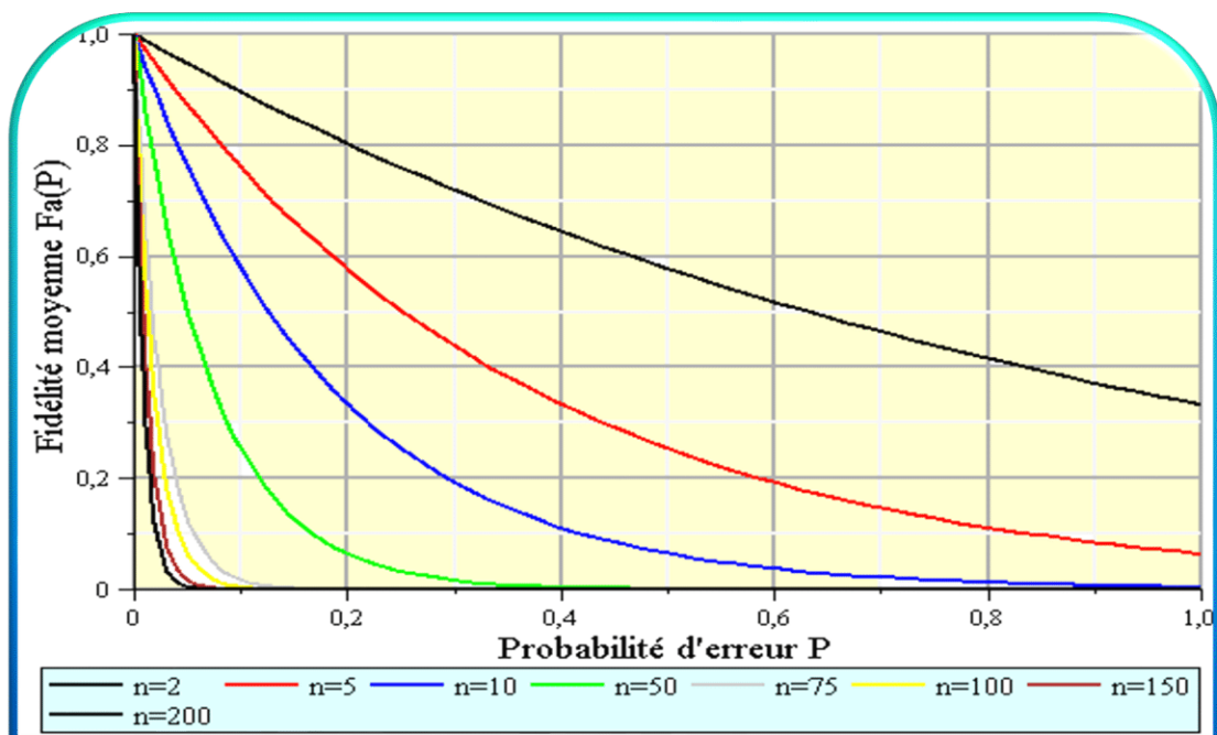
Figure 10 : Evolution de la fidélité en fonction de la probabilité P qu'une erreur affecte deux qubits durant la transmission pour différentes valeurs du nombre total n de qubits portant l'information utile.
