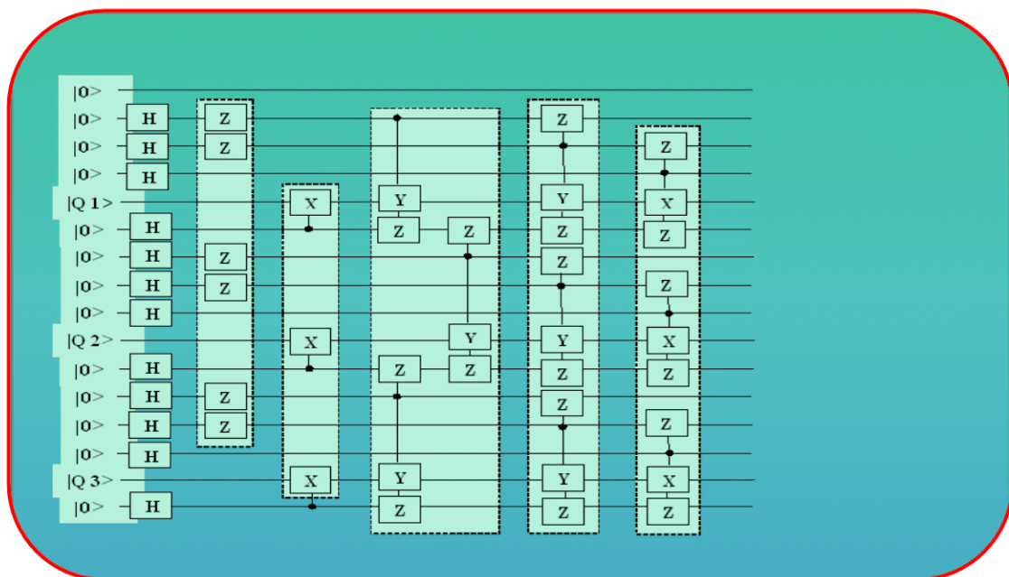
Figure 9 : Circuit de codage d'un code convolutif à cinq qubits [7].
