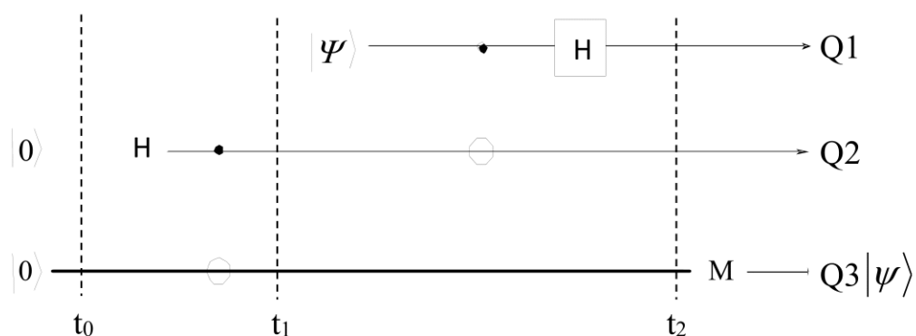
Figure 7 : Circuit de la téléportation. Alice possède les qubits (Q1,Q2) aux états initiaux |0\rangle et |\Psi\rangle puis finaux |0\rangle ou |1\rangle et Bob le qubit Q3 sur lequel il applique la porte M pour accéder à l'état |\Psi\rangle .
