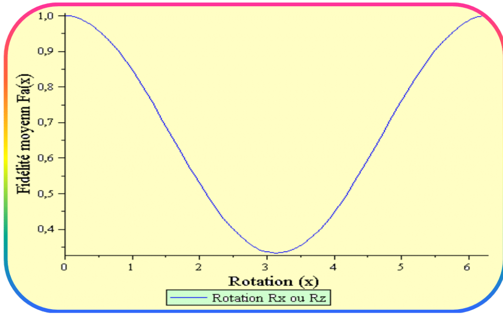
Figure 13 : Evolution de la fidélité moyenne F_a(x) en fonction de la valeur x de la rotation R_x(x) ou R_z(x) sur l'un des qubits 1, 2 ou 3.
