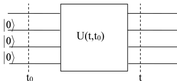
Figure 5 : Schéma général du calcul quantique.
