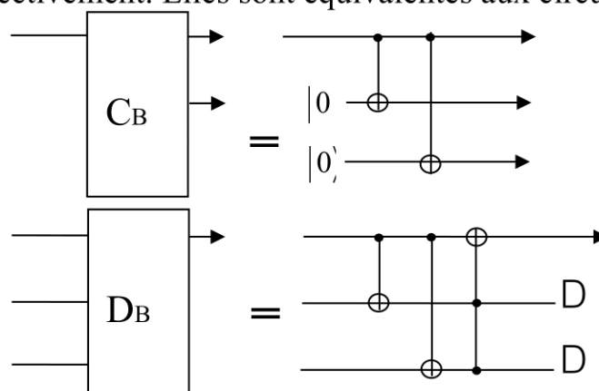
Figure E2 : Boîtes de codage ( C_B ) et décodage ( D_B ).
