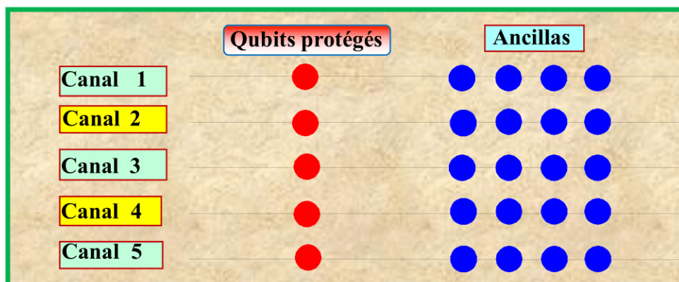
Figure 14 : Protection par le code à cinq qubits.
