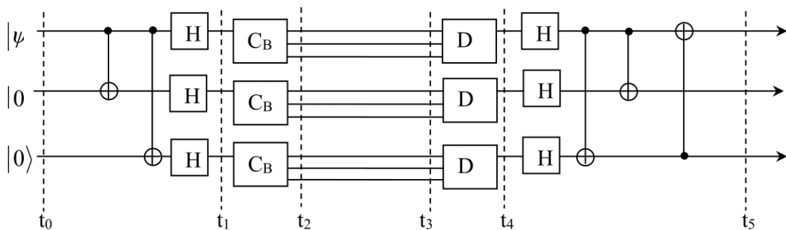
Figure E1 : Circuit de codage et décodage du code de Shor à neuf qubits.
