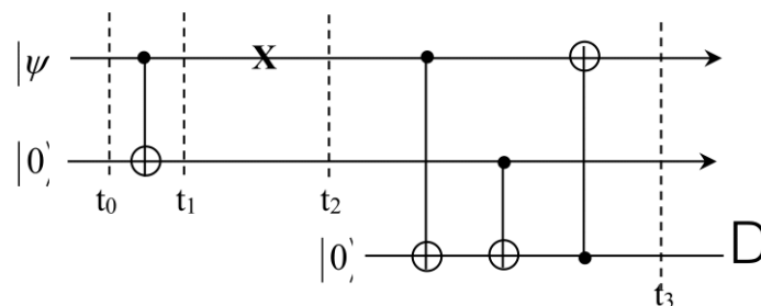
Figure C3 : Circuit quantique du code correcteur à deux qubits.
