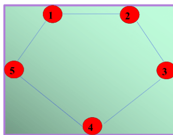
Figure 11 : Etat de graphe à cinq qubits |G\rangle .
