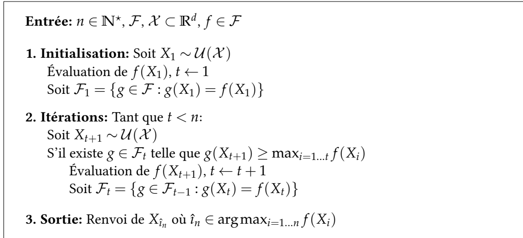
Figure V.1: Optimisation d'une fonction inconnue f appartenant à la classe \mathcal{F}
