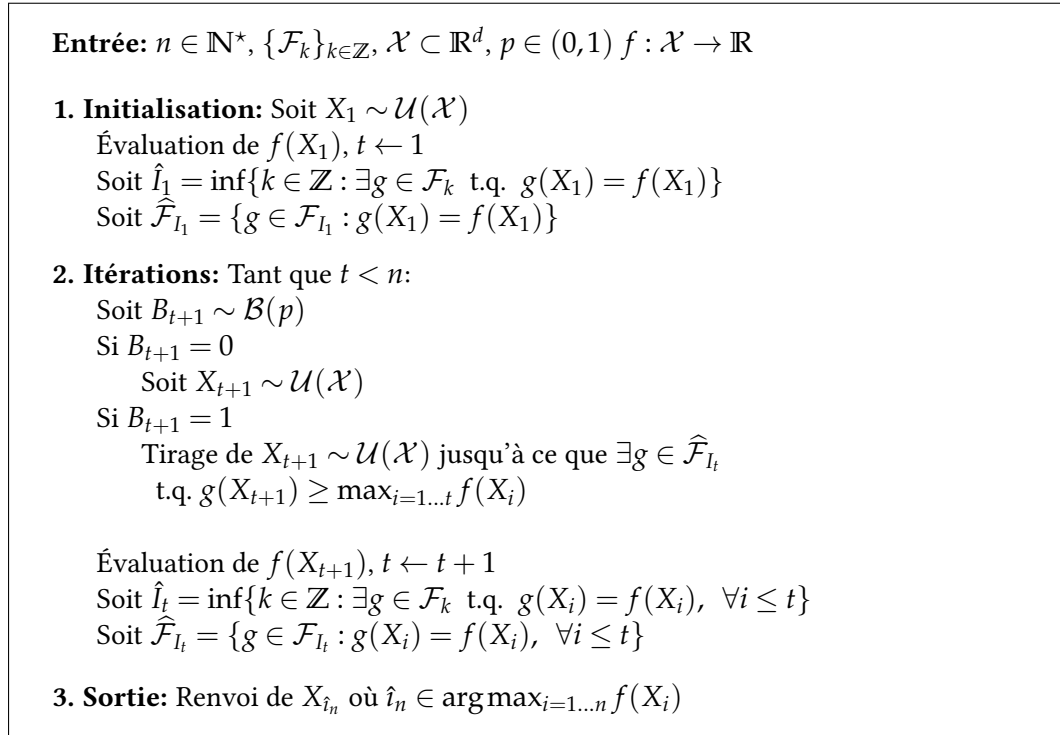
Figure V.2: Algorithme adaptatif sur une séquence \{\mathcal{F}_k\}_{k \in \mathbb{Z}} avec un paramètre p \in (0,1)
