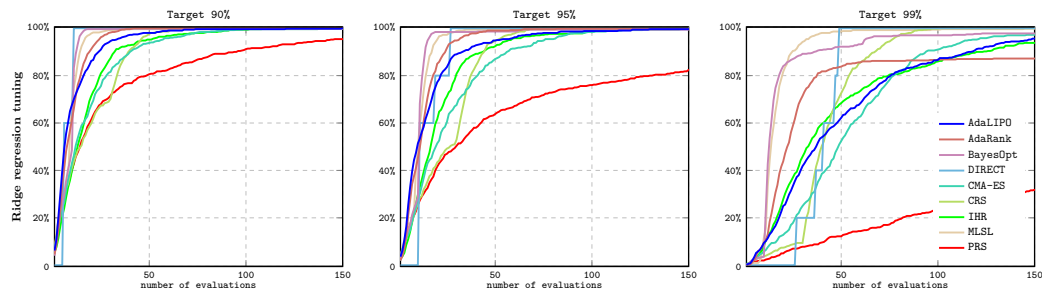
Figure V.3: Proportion du nombre d'expériences qui ont atteint les cibles 90%, 95% et 99% en fonction du nombre d'évaluations sur chacune des séries de problèmes.
