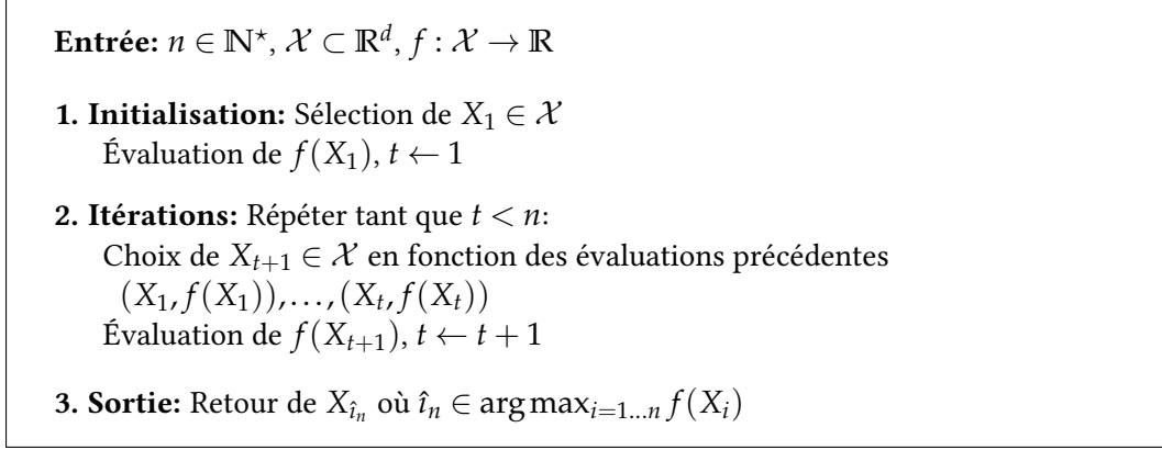
Figure II.1: Squelette d'une procédure d'optimisation séquentielle
