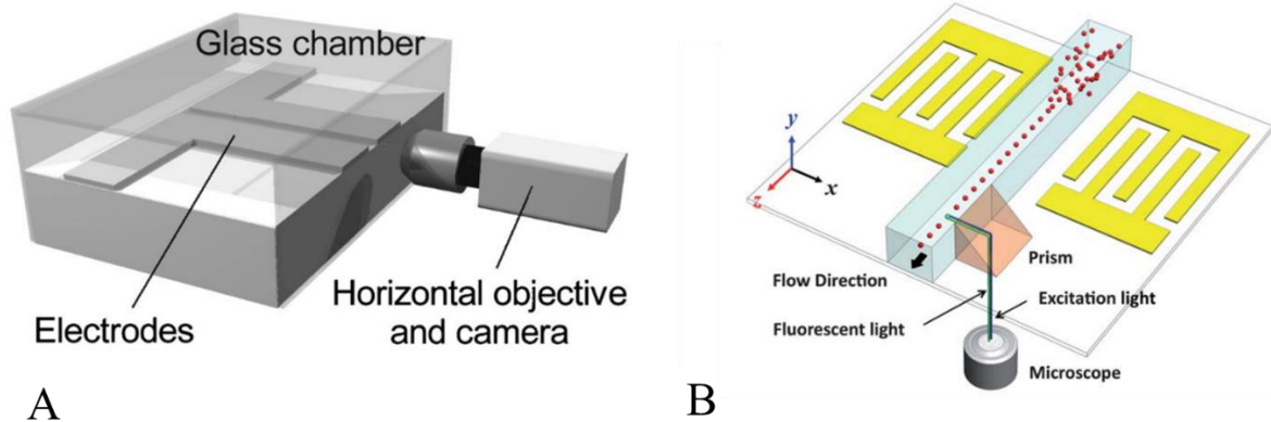
Figure 4-5 : Deux systèmes permettant une observation de côté d'une cellule fluïdique. A repose sur l'observation directe grâce à un objectif de microscope [103]. B propose d'utiliser un prisme [67] pour imager le côté d'un canal fluïdique.
