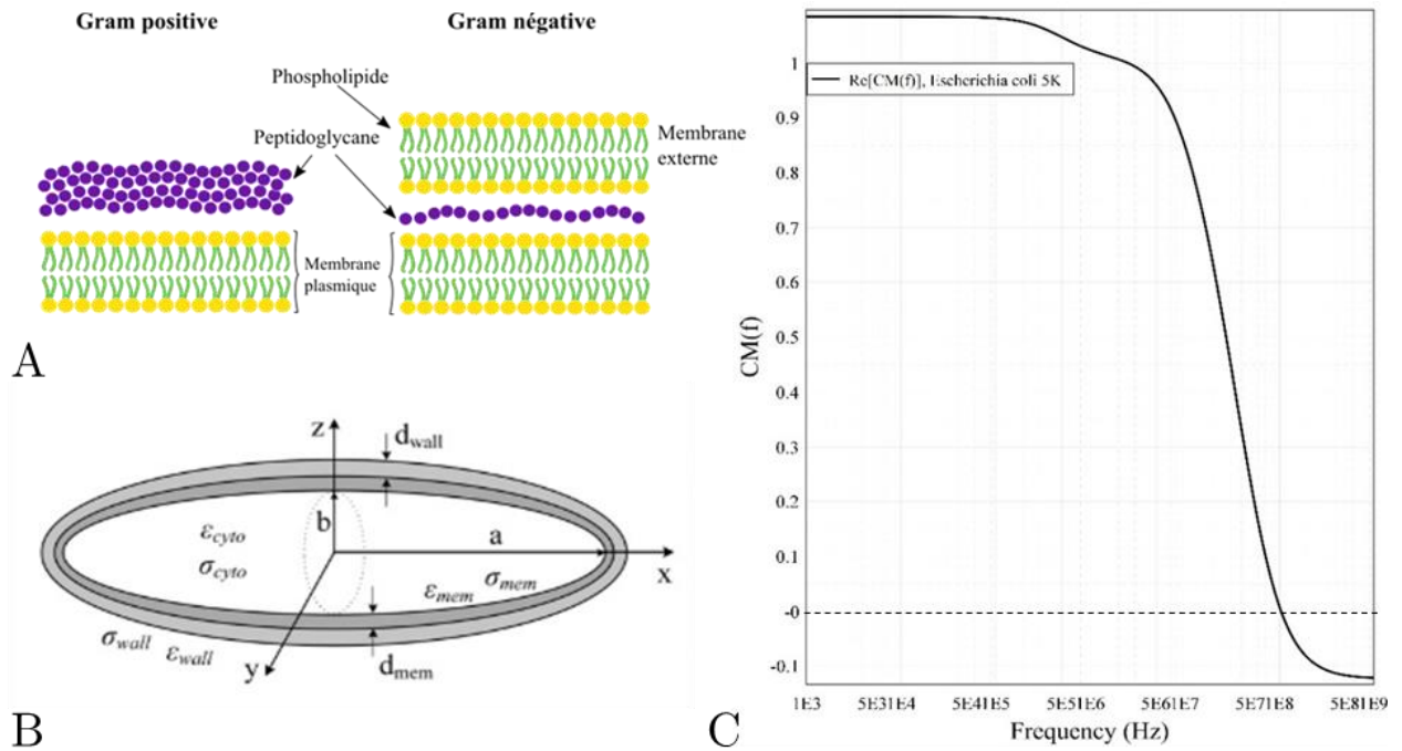
Figure 3-2A: Schéma de la membrane d'une bactérie de type Gram négatif ou Gram positif. B : Structure de la membrane retenue pour les simulations [132]. C : facteur de Clausius-Mossotti en fonction de la fréquence, calculé avec le logiciel MyDEP pour une bactérie de type e.coli et une conductivité de 6,6 \cdot 10^{-6} \text{ S/m} .
