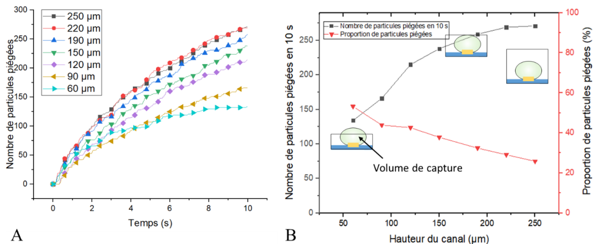
Figure 3-13A : Nombre de particules piégées sur l'électrode centrale pour différentes hauteurs du canal en fonction du temps. B : Nombre et pourcentage de particules piégées sur l'électrode centrale en 10 secondes, en fonction de la hauteur du canal.
