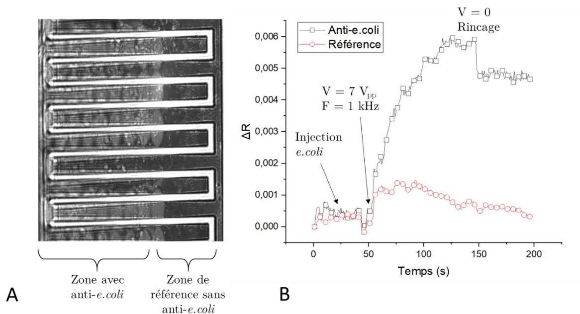
Figure 5-10A : Image SPR TM des électrodes avec la partie gauche fonctionnalisée avec des anticorps anti e.coli . B: Signal SPR mesuré sur une électrode fonctionnalisée avec des anticorps anti e.coli (en noir) et sur une électrode non fonctionnalisée (en rouge).
