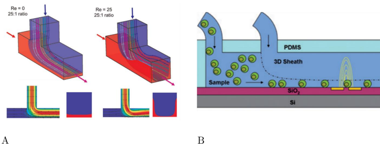
Figure 2-7A : Dépendance au nombre de Reynolds sur l'interface entre deux types de fluides [55]. B : Détection par impédancemétrie de cellules pré-concentrées par concentration hydrodynamique [56].
