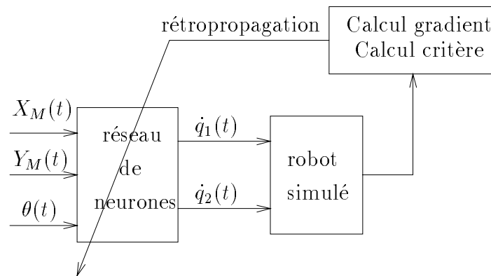
Fig. 7.2: Apprentissage Hors-ligne
