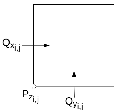
FIGURE 2.2 – Placement et indigage des composantes P_z , Q_x et Q_y dans une cellule de Yee.
