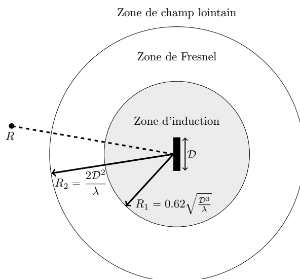
FIGURE 1.1 – Régions de champ diffracté par une antenne de dimension principale égale à \mathcal{D} .
