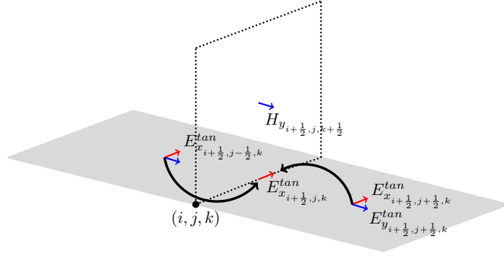
FIGURE 4.7 – Interpolation de E_x tangent pour la mise à jour de H_y . La composante E_x^{tan} placée au centre de la facette a une contribution de 0.5 pour les deux composantes H_y situées sur les faces orthogonales à la paroi dans la cellule de Yee.
