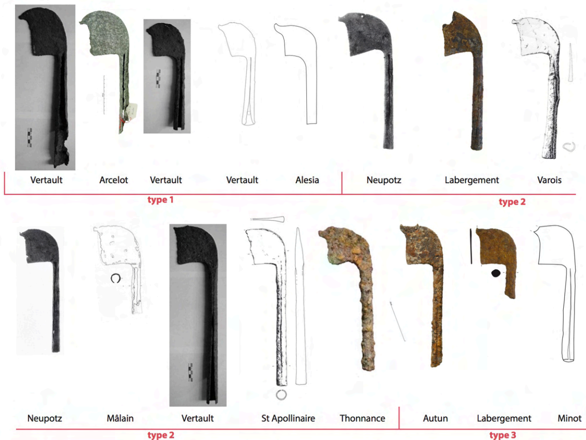
Figure 150. Typologie des serpes à excroissance (poster inédit N. Tisserand & B. Fort).
