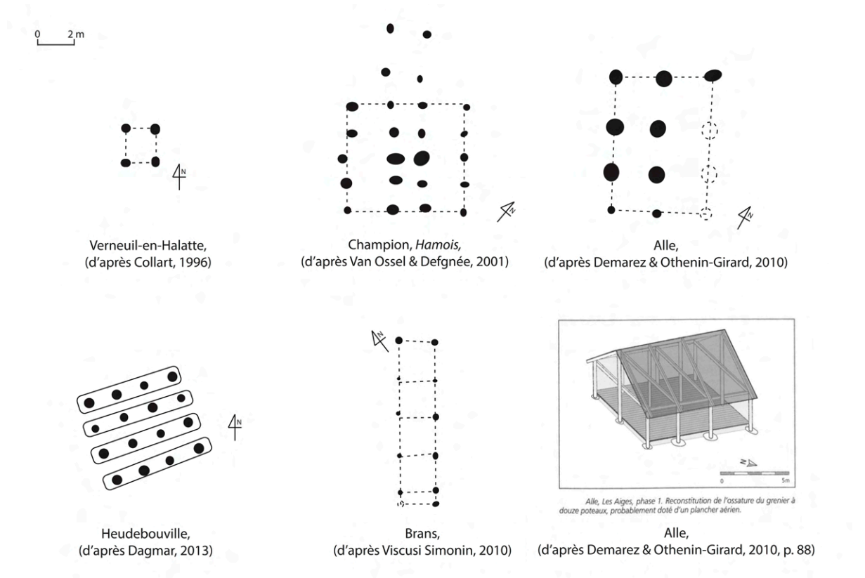
Figure 37. Exemples de greniers sur poteaux du catalogue. Grenier aérien et greniers sur plateforme basse.
