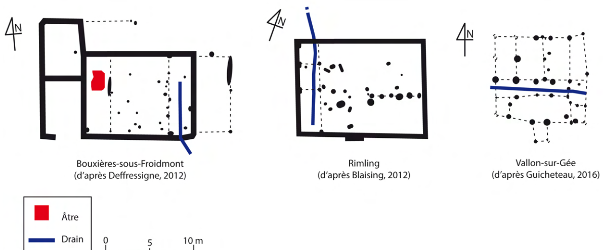
Figure 27. Exemples de bâtiments rectangulaires avec espace de stabulation et drain d'évacuation.
