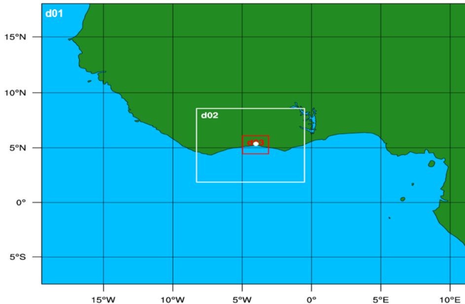
Figure 6.3 : Trois domaines WRF-Chem utilisés dans cette étude. Le point blanc plein montre le centre des domaines situé Abidjan.
