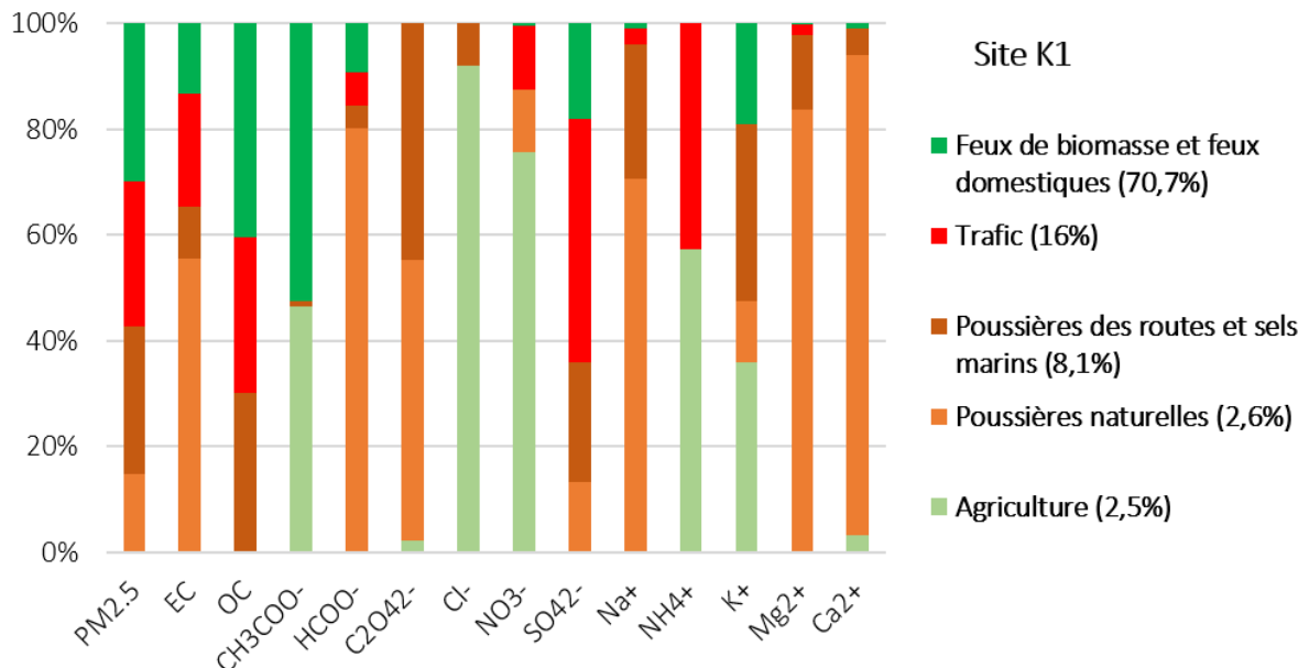
Figure 3.13 : Contribution des sources aux masses des différentes espèces analysées, avec entre parenthèses dans la légende le pourcentage de contribution moyen de la source à la masse des aérosols PM 2.5 du site K1.
