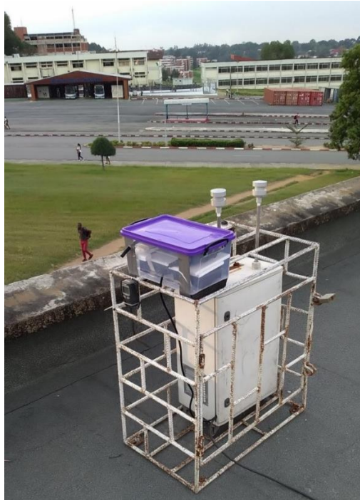
Figure 2.4 : Image des équipements installés sur le site A1, situé à l'Université Félix Houphouët-Boigny (Cocody).
