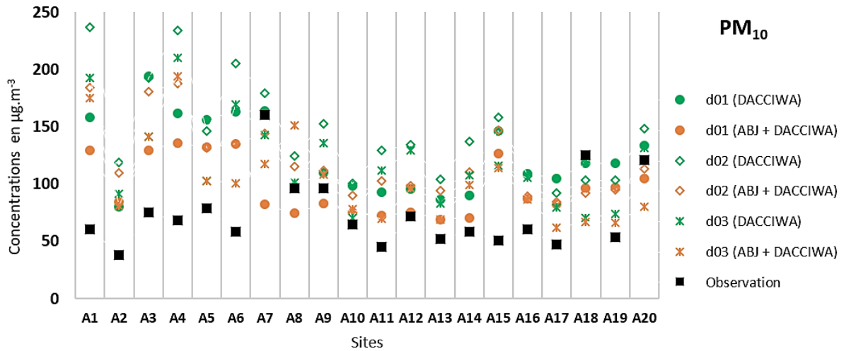
Figure 6.4 : Comparaison des concentrations moyennes des PM_{10} simulées par WRF-Chem pour chacun de domaine (d01, d02 et d03) et pour chacune des simulation (DACCIWA et ABJ + DACCIWA) avec les valeurs obtenues pendant la campagne intensive d'Abidjan.
