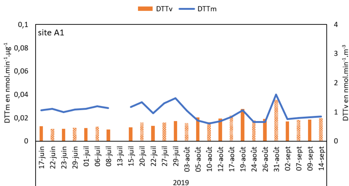
Figure 4.9 : Activités oxydantes journalières (DTTm et DTTv) moyennes des aérosols PM_{2.5} , collectés sur le site A1, avec le DTTm (ligne bleue) et le DTTv (barres orange) pendant la CSH, où les barres sans motifs représentent les jours ouvrables et les barres avec les motifs pointillés représentent les jours de week-end.
