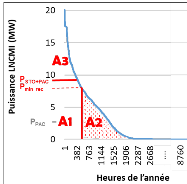
Figure IV.6 : Monotone des consommations électriques des aimants du LNCMI, avec A_1+A_2+A_3 la chaleur fatale théorique, A_1+A_3 la chaleur fatale disponible et A_1 la chaleur fatale récupérable. Source : auteur.
