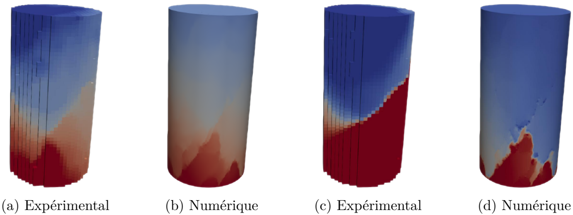
Fig. 21 – Issu de [Stamati, 2020] : Champs de déplacement expérimentaux et numériques pour la compression triaxiale à 5MPa à deux niveaux de chargement : (a) et (b) avant rupture et (c) et (d) après rupture.
