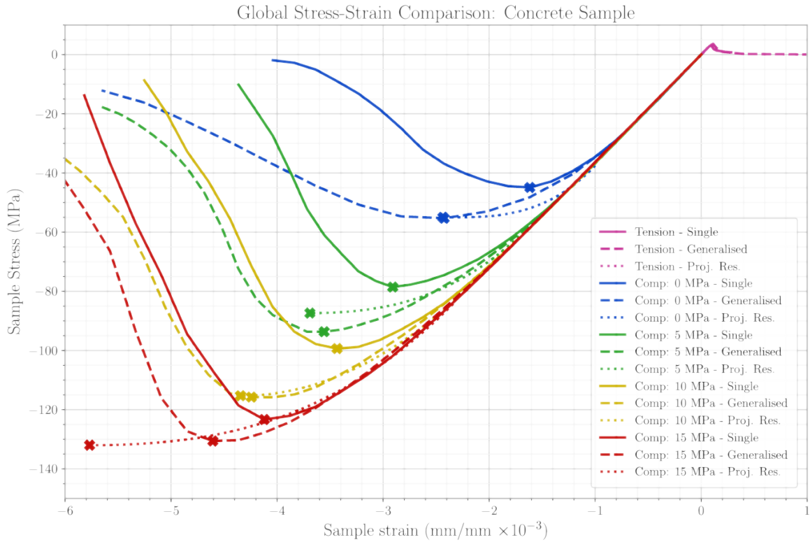
Fig. 20 – Issu de [Ortega Laborin, 2021] : comparaison des comportements macroscopiques entre les résultats expérimentaux (pointillés), modèle en mode I (tirets), modèle généralisé (traits pleins).
