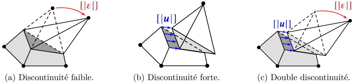
Fig. 11 – Issu de [Sun et al., 2021a] : Représentation des discontinuités faibles et fortes dans le cas d'un glissement de fissure en mode II.
