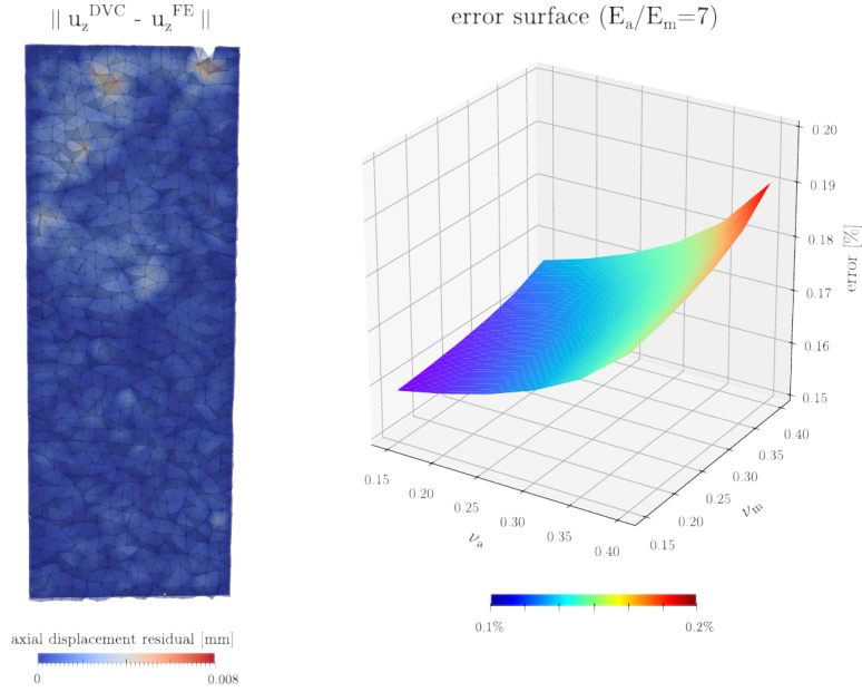
Fig. 29 – Issu de [Stamati, 2020] : couplage faible entre calculs E-FEM et corrélation d’image globale.
