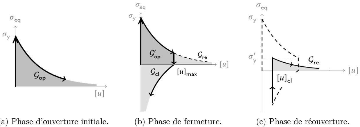
Fig. 9 – Issu de [Sun et al., 2021b] : Loi de traction/séparation définie par les critères \Phi_{op} et \Phi_{cl} , régissant le comportement à l'interface des discontinuités fortes et définissant les lois d'ouverture et de fermeture des fissures.
