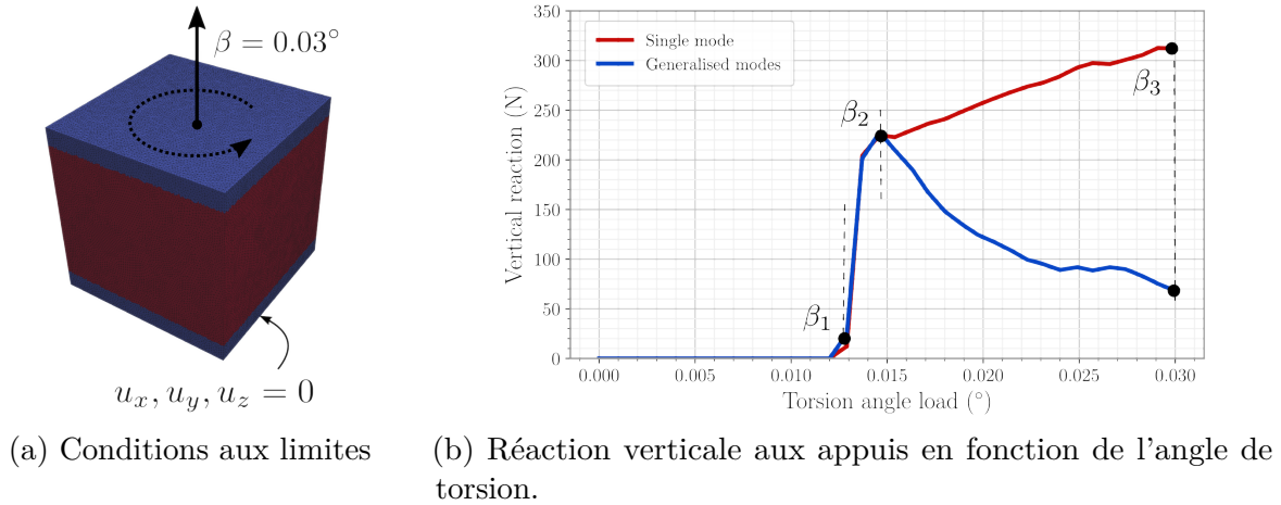
Fig. 14 – Issu de [Ortega Laborin et al., 2021c] : Généralisation du modèle E-FEM et résolution des problématiques de couplage des contraintes.
