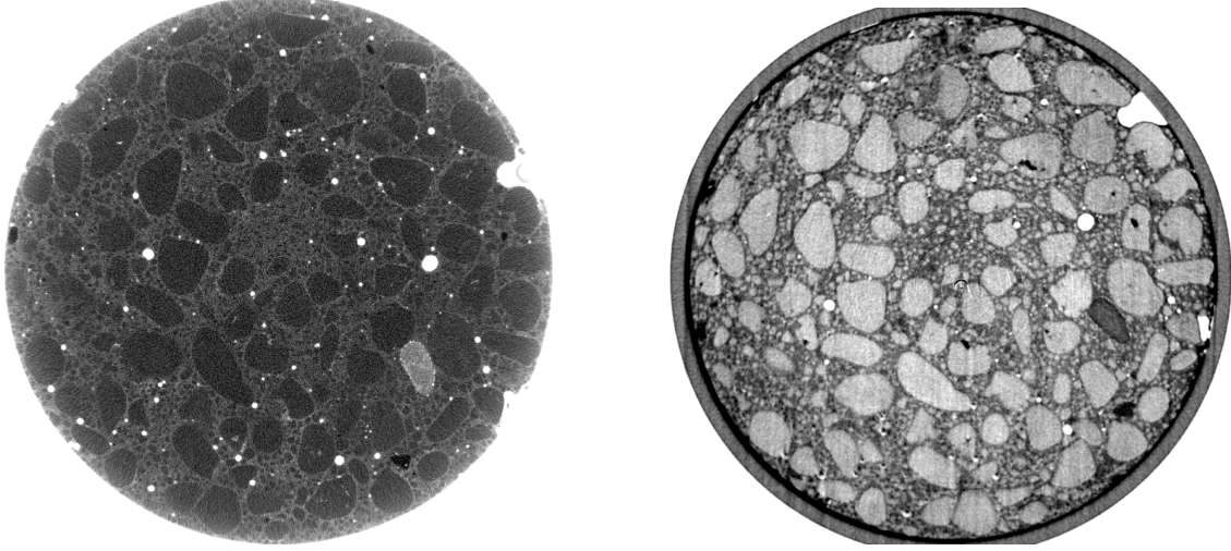
(a) f_x(\mathbf{x}) : champ d'atténuation des rayons X. (b) f_n(\mathbf{x}) : champ d'atténuation des neutrons.
