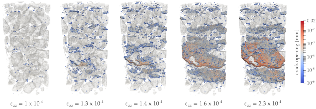
Fig. 6 – Issu de [Stamati, 2020] : évolution de la répartition de la microfissuration au cours d’un essai de traction simple et coalescence des fissures locales (discontinuités fortes) en une macrofissure en fin d’essai.
