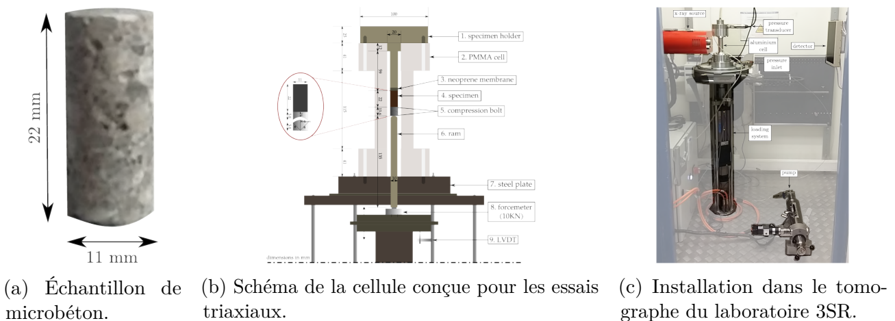
Fig. 15 – Issu de [Stamati et al., 2021b] : Essais triaxiaux in-situ sur des échantillons de microbéton dans le microtomographe du laboratoire 3SR.
