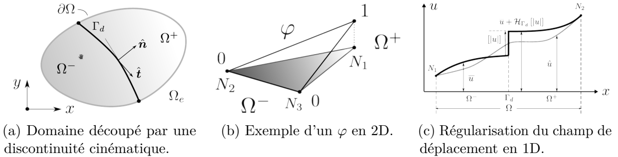
Fig. 5 – Issu de [Ortega Laborin et al., 2021c] : Illustrations classiques de la cinématique des discontinuités fortes.
