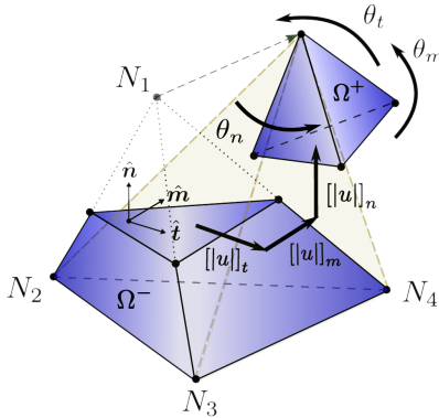
(a) Illustration d'une cinématique généralisée d'un mode de rupture sur un tétraèdre
