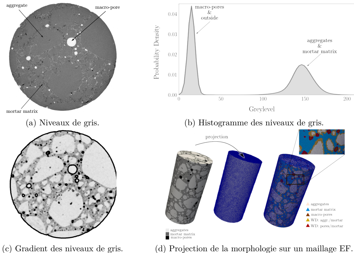
Fig. 19 – Issu de [Stamati et al., 2018a] : Méthode d'identification des phases de tomographies de béton.
