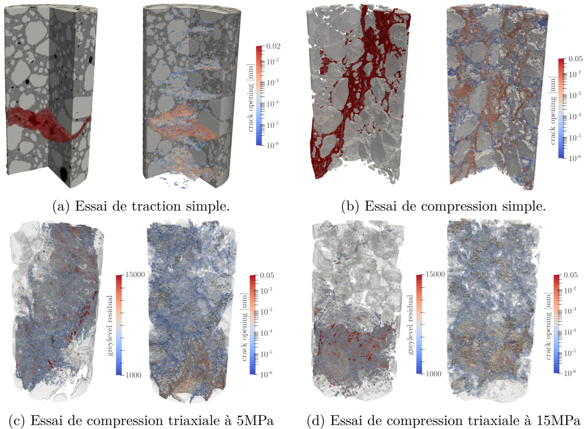
Fig. 22 – Issu de [Stamati, 2020] : Comparaison des faciès de fissuration expérimentaux (à gauche) et numériques (à droite). Les faciès de fissuration expérimentaux sont obtenus par seuillage de niveau de gris pour (a) et (b) et par seuillage de résidu \eta pour (c) et (d).
