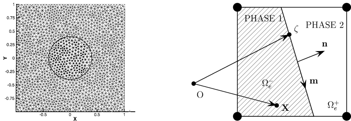
(a) Issu de [Sukumar et al., 2001] : Maillage non conforme utilisé pour une simulation X-FEM d'un matériau biphasique. (b) Issu de [Markovic, 2004] : Interface entre deux phases.
