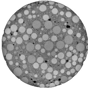
(a) Issu de [Paulina, 2013] : Tranche d'une tomographie d'un des bétons utilisés (billes de verre) pour la comparaison.
