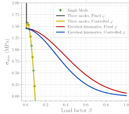
(b) Différents comportements de la contrainte de cisaillement en fonction de la complexité cinématique du modèle.
