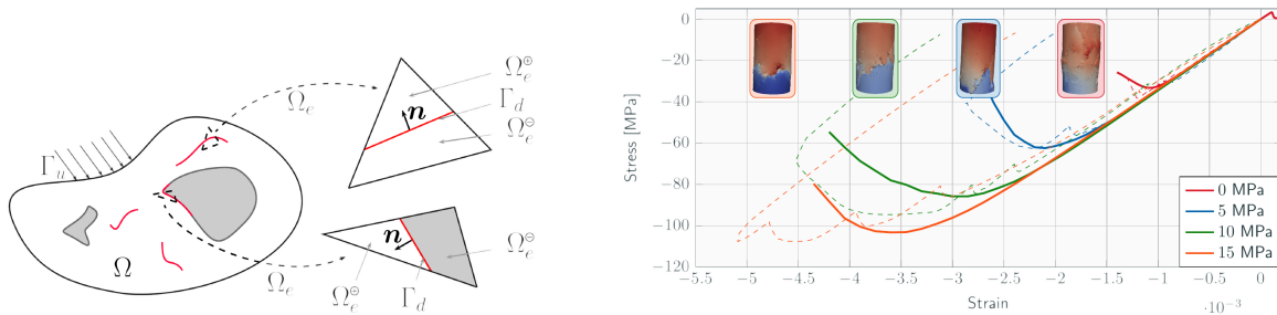
Fig. 31 – Modèle mésoscopique utilisé [Roubin et al., 2015b]
