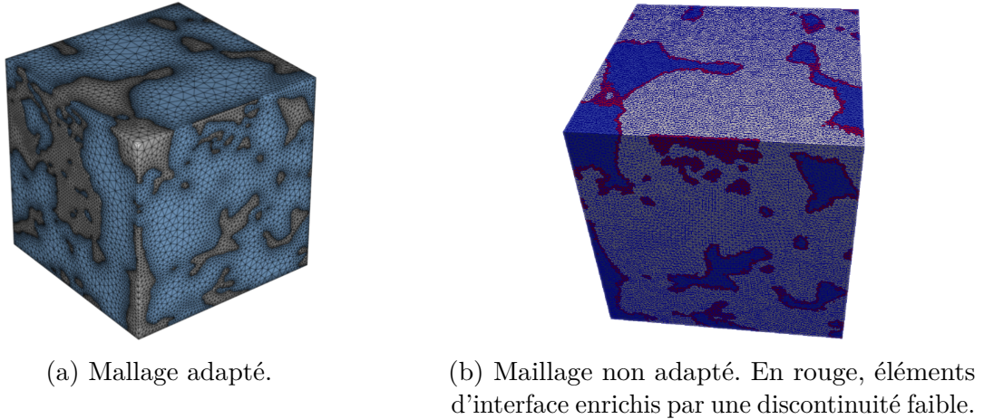
Fig. 7 – Issu de [Ehab Moustafa Kamel et al., 2019] : Illustration des différentes méthodes de maillage sur la même morphologie.
