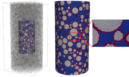
(b) Projection de la morphologie simulée par un empilement de sphères sur le maillage EF.
