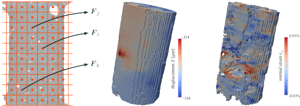
Fig. 27 – Issu de [Stamati, 2020] : principe de la méthode de corrélation d'images dite "locale".
