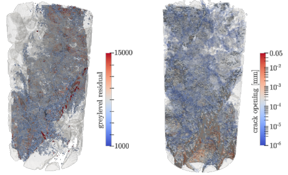
(b) Faciès de fissuration en compression confinée à 5MPa (gauche : expérimental, droite : numérique)
