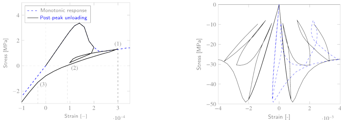
(a) (1) Fissuration en traction. (2) État de compression. (3) Récupération de la rigidité avec la fermeture des fissures. (b) Boucles d'hystérésis lors d'essais de compression cyclique.
