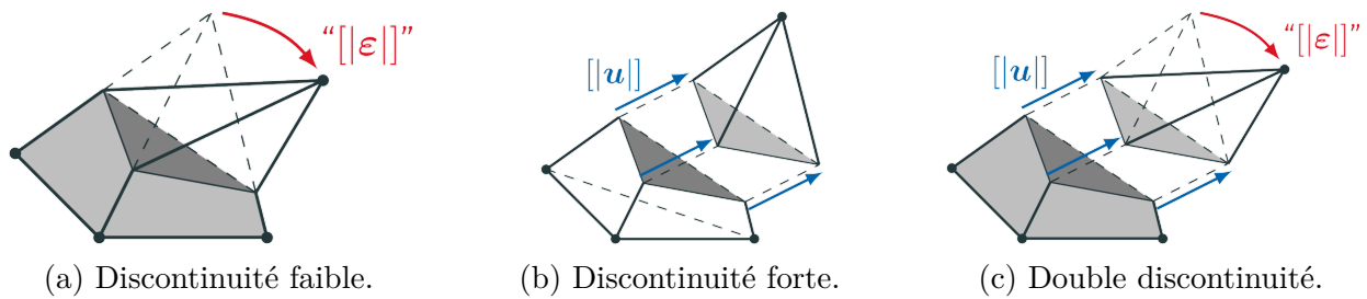
Fig. 8 – Issu de [Roubin et al., 2019b] : Représentation des discontinuités faibles et fortes au sein d'un élément fini dans le cas d'une ouverture en mode I.
