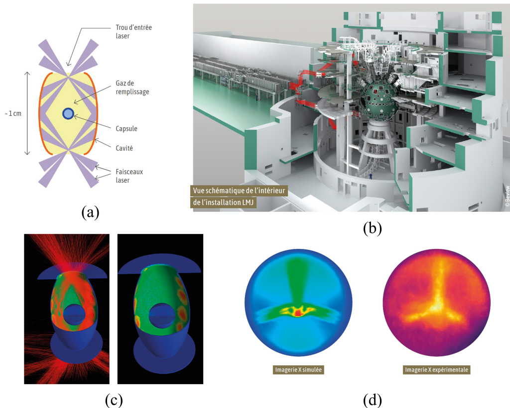
FIGURE 1.2 – Expérience de fusion nucléaire réalisée au Laser Mégajoule (LMJ) au CEA Cesta (extrait de http://www-lmj.cea.fr/docs/2020/Plaquette-LMJ-fusion.pdf ). (a) Schéma de l'expérience physique étudiée, (b) installation physique permettant de réaliser l'expérience, (c) simulation effectuée sur le supercalculateur Tera 1000-2 et (d) comparaison entre l'expérience physique et la simulation.
