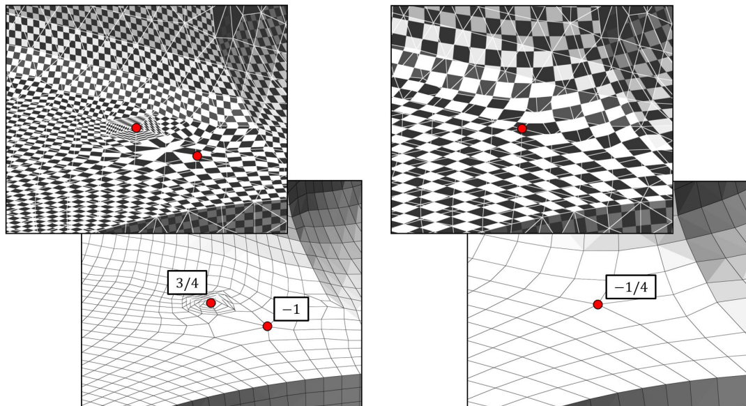
FIGURE 3.44 – Le lisseur variationnel peut générer des superpositions (en haut à gauche). Il produit un sommet singulier supplémentaire dans le maillage quadrangulaire (en bas à gauche). Nous pouvons résoudre ce problème en utilisant notre ajout de triangles fantômes.
