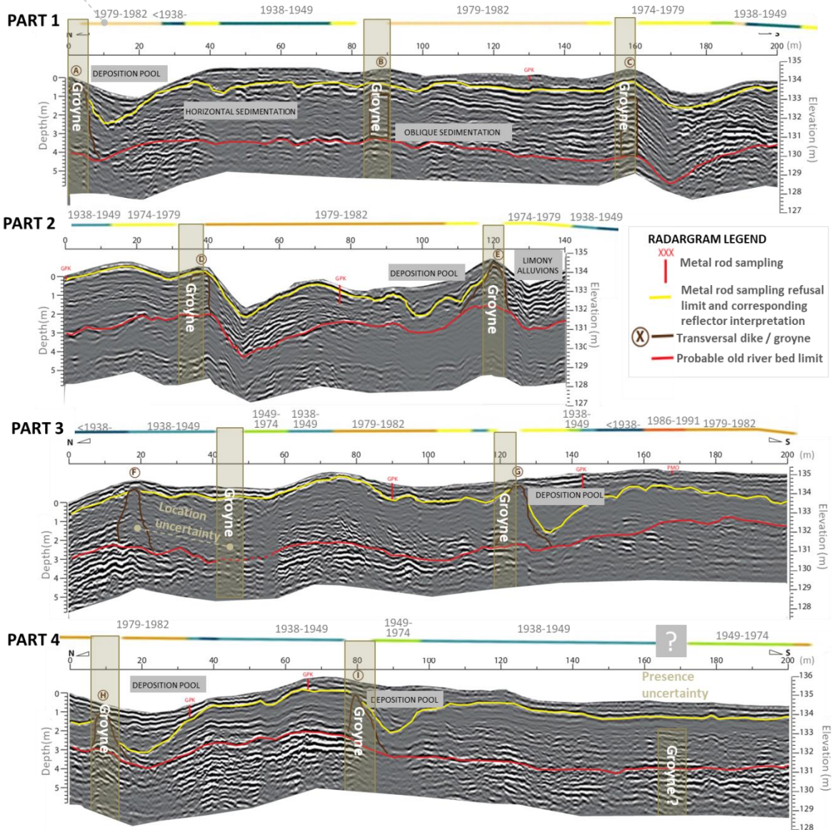
Figure 125 : Radargramme « B » traversant des champs d'épis (succession de structures ouvertes) à PDR (PK 54, rive droite) et sa contextualisation chrono-planimétrique. Source des radargrammes interprétés : T.Winiarski (ENTPE, OSR4)
