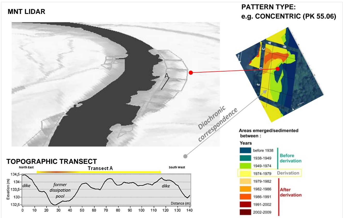
Figure 55 : Principe d'échantillonnage pour les correspondances topographiques des patrons 2D
