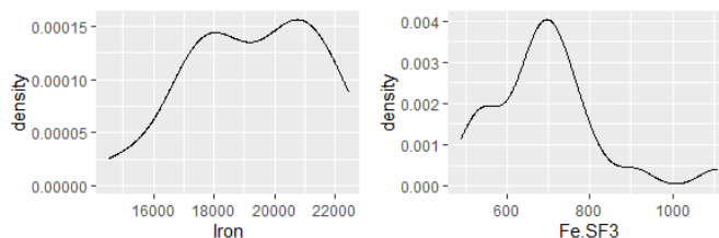
Figure 62 : Distributions du fer et du ratio fer/Fraction SF3 [0,63\mu\text{m}-2\mu\text{m}] %
