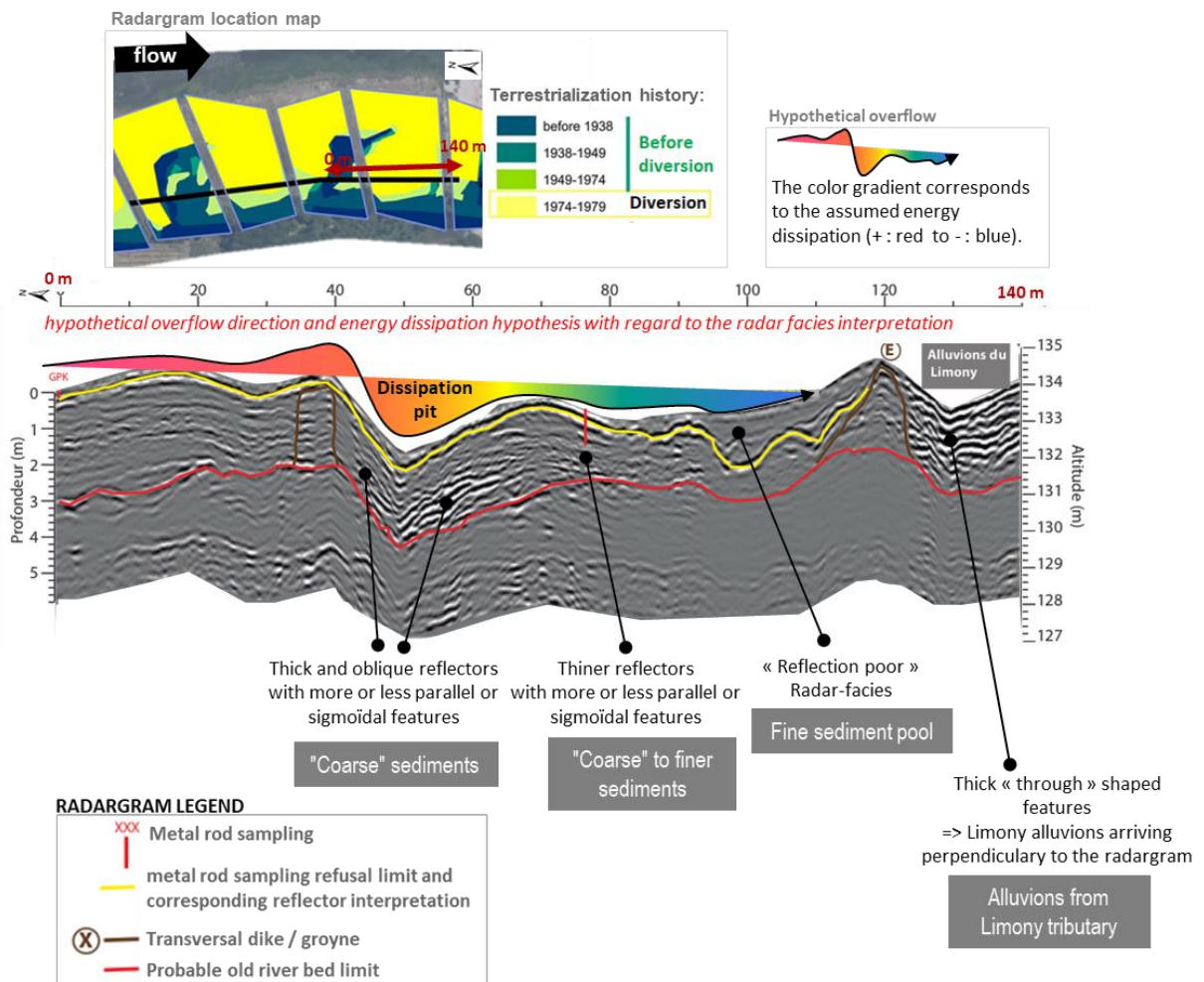
Figure 130 : Fosse de dissipation mise en évidence par l'interprétation des radarfaciès sur la partie 2 du GPR B -213-
