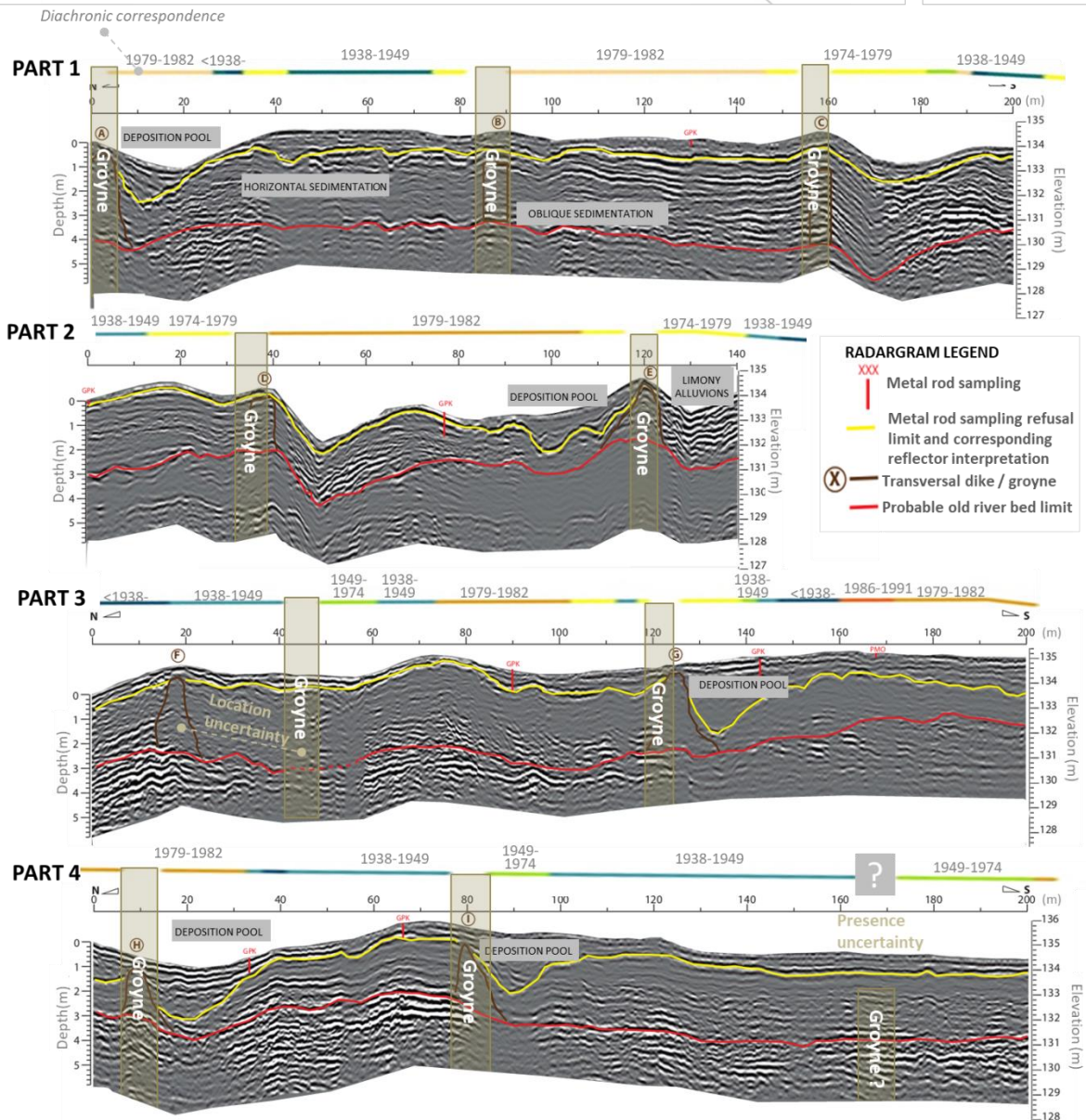
Figure 125 : Radargramme « B » traversant des champs d'épis (succession de structures ouvertes) à PDR (PK 54, rive droite) et sa contextualisation chrono-planimétrique. Source des radargrammes interprétés : T.Winiarski (ENTPE, OSR4)
