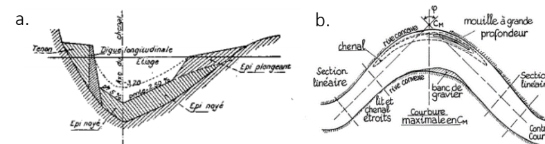
Figure 30 : a. Courbure maximale et son angle associé \phi , b. Schéma de la géométrie des ouvrages où la courbure est la plus forte, issu de Combe et
