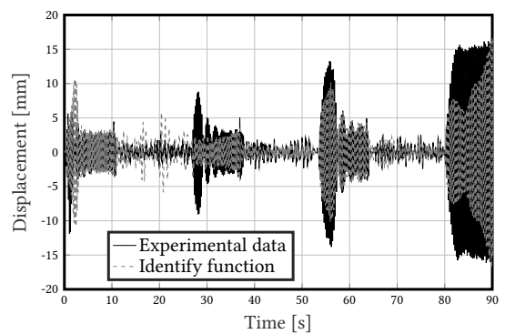
(d) DSS3 test - displacement
