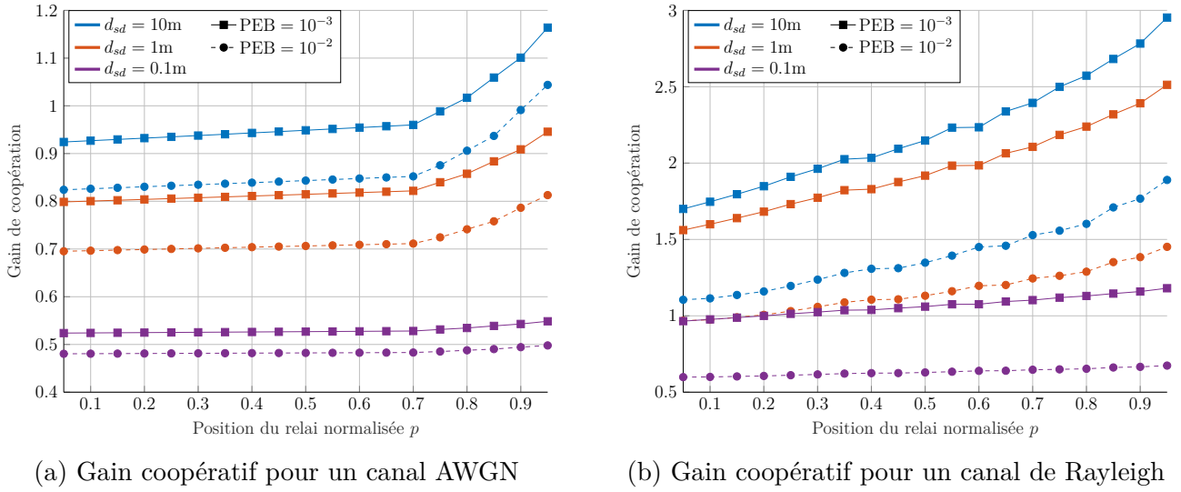
FIGURE 4.25 – Gain de coopération pour une M-QAM ( M = 2^b ) sur un canal AWGN ou de Rayleigh en fonction de la position normalisée du relai pour différentes PEB
