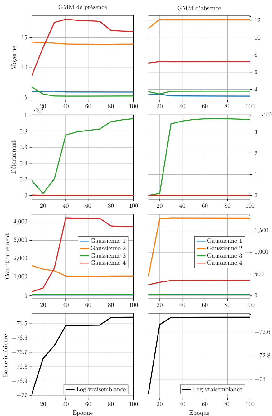
FIGURE 2.8 – Evolution de la moyenne, du déterminant et du conditionnement de la matrice de covariance pour chacune des quatre gaussiennes, et borne inférieure de la log-vraisemblance au cours du temps (en époque), pour les classifieurs de présence (à gauche) et d'absence (à droite) et la classe people speaking
