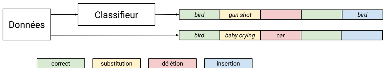
FIGURE 2.5 – Schéma du comptage des substitutions, délétions et insertions
