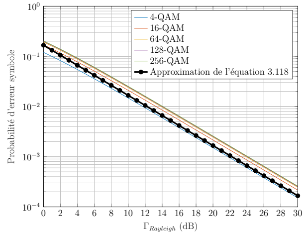
(b) PEB en fonction de la pénalité en RSB symbole \Gamma_{Rayleigh} pour une source modulée dans un canal de Rayleigh
