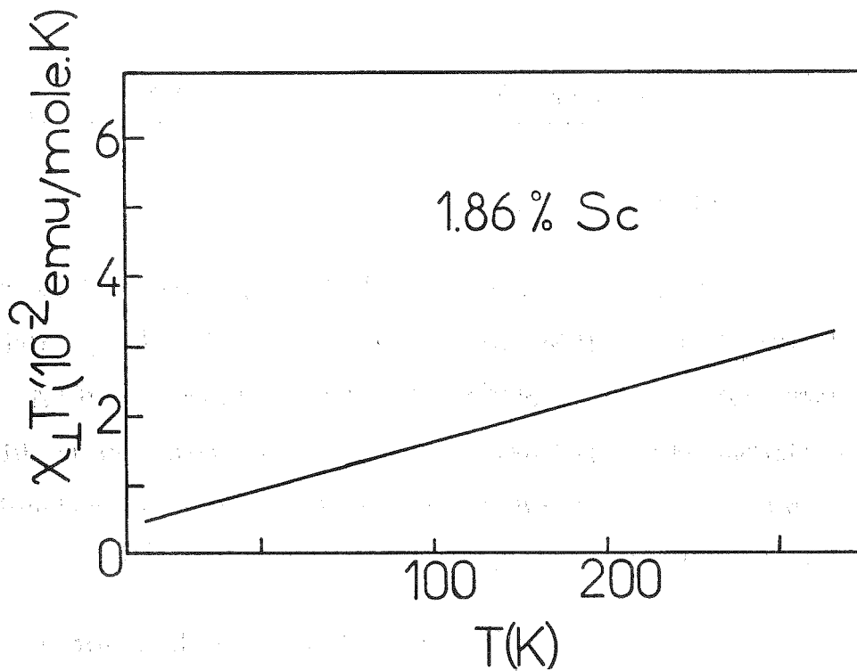
Fig. 36 : \chi T en fonction de T pour Ti_2O_3 dopé au Sc.
