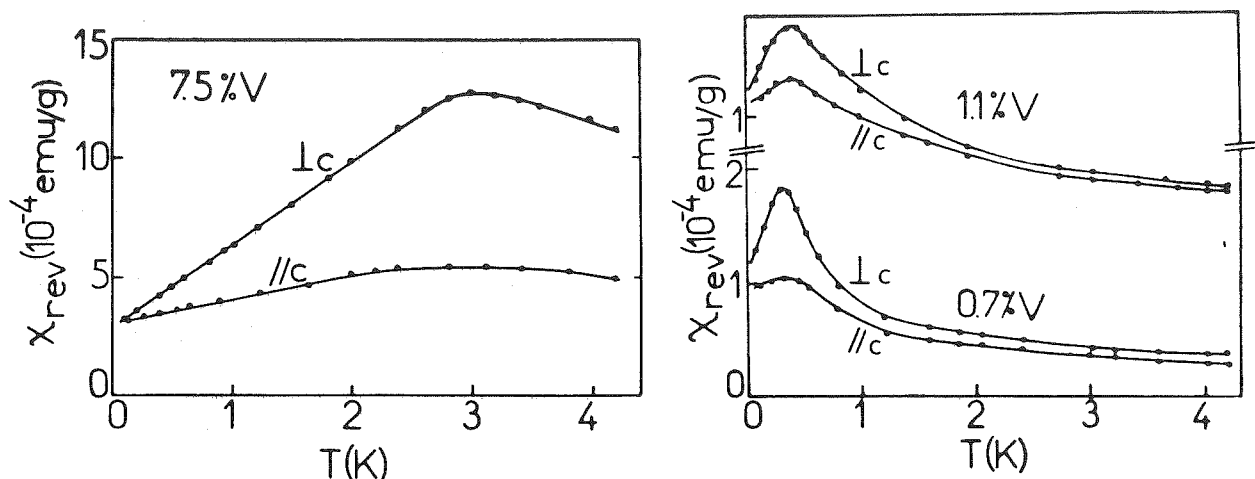
Fig. 73 : \chi_{rev//} et \chi_{rev\perp} pour x = 7,5\% V . Fig. 74 : \chi_{rev//} et \chi_{rev\perp} pour x = 1,1\% V ; x = 0,7\% V .
