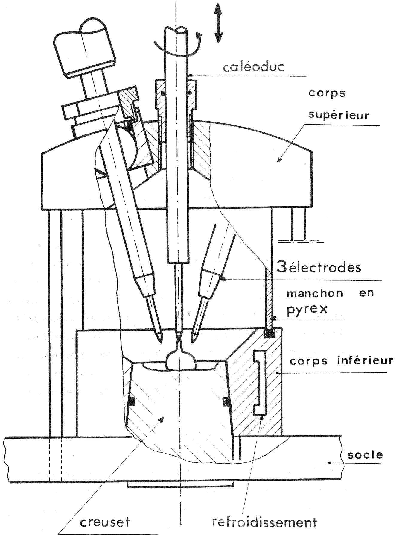
Fig. 29 : Schéma du four Triarc (Echelle 1/1).
