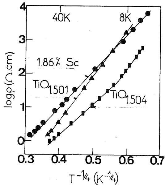
Figure 47 : Résistivité de \text{Ti}_2\text{O}_3 et de \text{Ti}_2\text{O}_3 dopé au Sc en fonction de T^{-1/4} .
