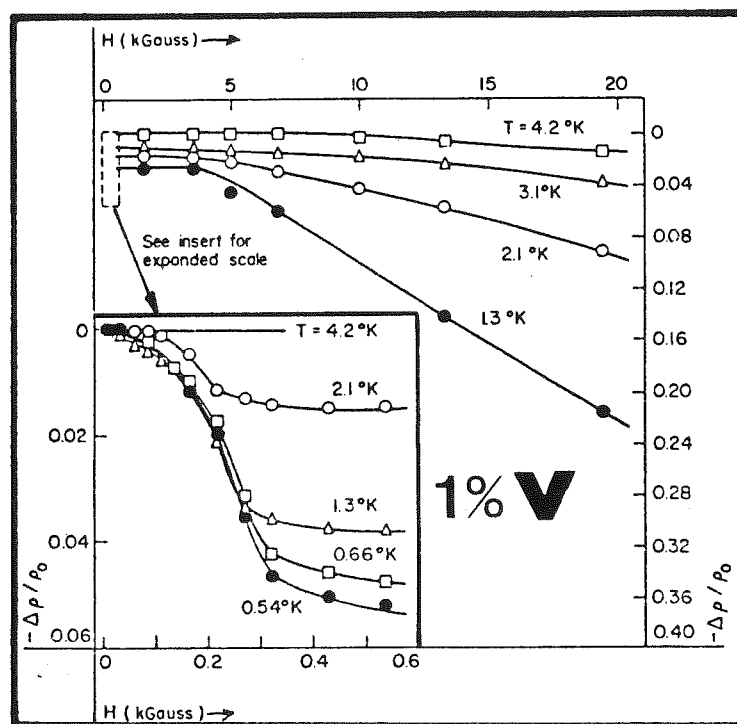
Fig. 17 : Magnétorésistance négative en fonction du champ appliqué.
