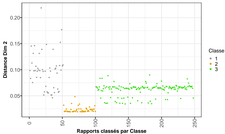
FIGURE 5.3 – Distance entre les représentations des textes et leurs projections pour la classe 2 HDDC pour la représentation unigramme.
