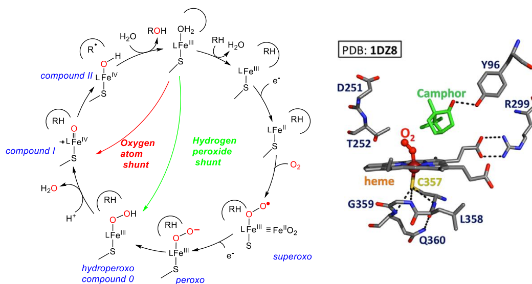
Figure 88 (Gauche) Cycle catalytique proposé pour les enzymes Cyt P450. Toutes les espèces intermédiaires citées ont été observées dans littérature par spectroscopie, mais la structure cristalline des intermédiaires, y compris les Cmpd I et II peroxy et hydroperoxy, n'est pas encore disponible. (Droite) Vue rapprochée du oxy-Cyt P450 mettant en évidence le substrat camphre, le centre hémique hexacoordinné et les interactions critiques de liaison H impliquant le résidu cystéine.
