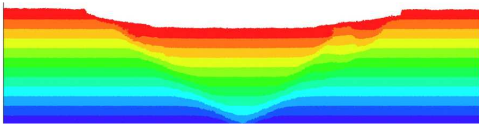
FIGURE 4.7 – Résultat préliminaire d'une simulation de la déformation d'un matériau granulaire cohésif et friable sous l'effet d'une extension, imposée ici via une vitesse radiale fixe des particules constituant la paroi inférieure.
