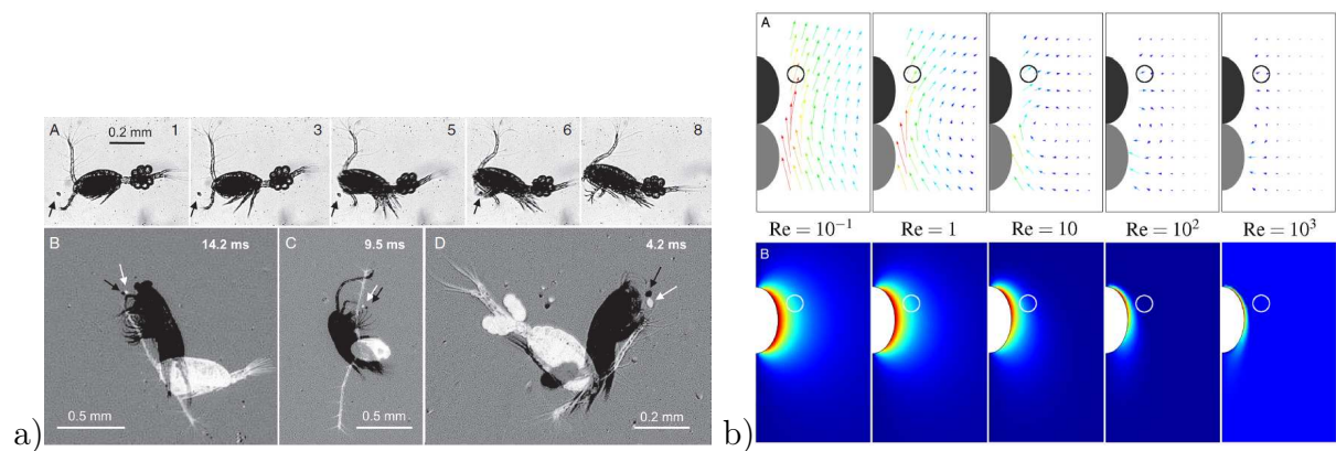
FIGURE 5.15 – a) Attaque d'un organisme unicellulaire par un copéode : les flèches indiquent la position de la proie aux instants initial et final. On constate qu'elle n'a quasiment pas bougé sous l'effet du saut. b) Modèle hydrodynamique des déplacements induits au voisinage du copéode par son mouvement d'attaque : on observe que le nombre de Reynolds doit dépasser un certain seuil pour que la proie ne soit ni repoussée ni avertie par un cisaillement significatif [10].
