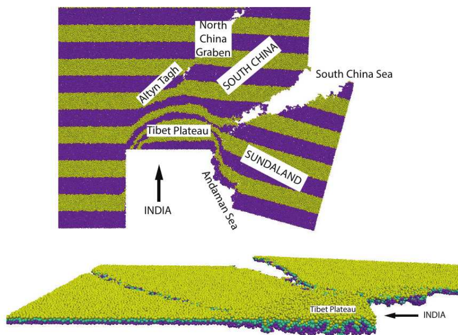
FIGURE 4.6 – Exemple de simulation en éléments discrets de la déformation lithosphérique due à la collision Inde-Asie [Jiao, 2016].
