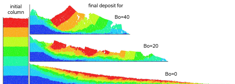
FIGURE 2.4 – Aspect du dépôt final pour des valeurs décroissantes du nombre de Bond initial. Les couleurs indiquent la provenance verticale des particules dans la colonne initiale [7].
