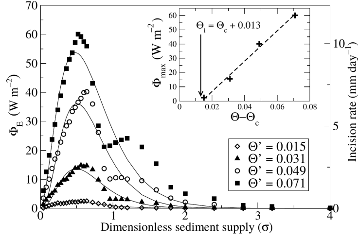
FIGURE 1.9 – Énergie \Phi_E dissipée sur le socle par les impacts de charriage, par unité de temps et de surface, en fonction de la quantité de sédiments disponibles. Le taux d'incision équivalent est calculé via l'équation 1.9 [6].
