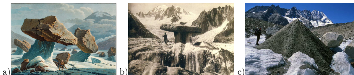
FIGURE 5.9 – a) « Les pierres sur le glacier de l'Aar » [aquarelle J. Hürlimann, 1822]; b) table glaciaire sur le glacier du Talèfre [photographie R. Vivian]; c) Cône de débris sur le glacier de l'Unteraar (Suisse) [photographie J. Alean].
