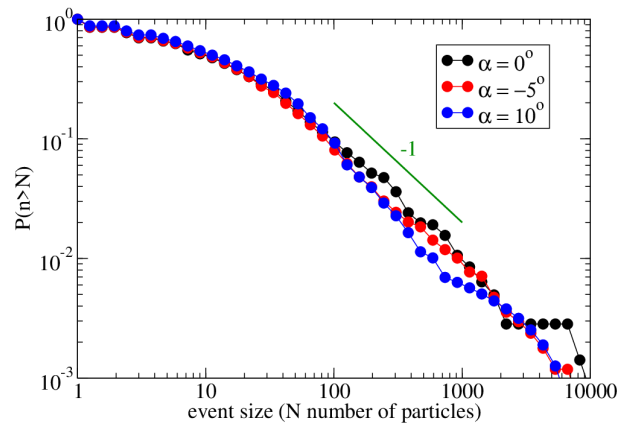
FIGURE 2.13 – Distribution des tailles d'éboulements observés dans la simulation, en fonction du pendage des couches lithologiques. Comme sur le terrain, on observe une décroissance en loi de puissance (similaire à la loi de Gutenberg-Richter pour les séismes).
