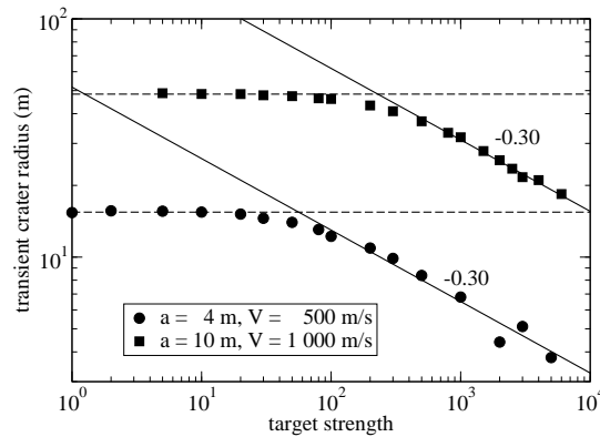
FIGURE 3.8 – Rayon maximal du cratère transitoire (quasi-circulaire) en fonction de la résistance du matériau cible, pour deux impacts d'énergie cinétique différente.
