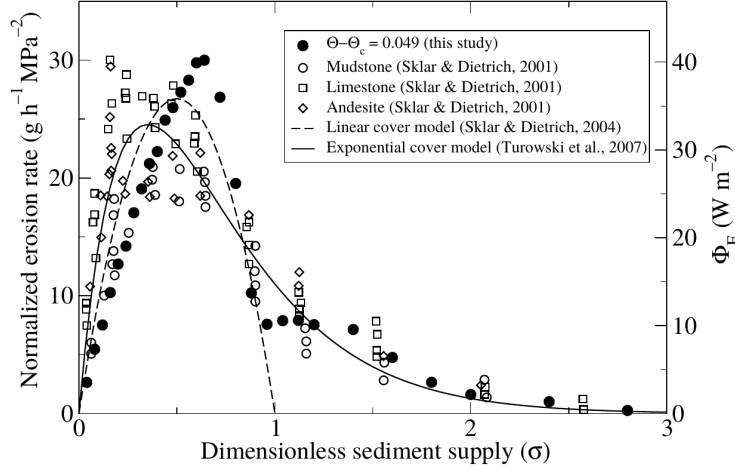
FIGURE 1.8 – Énergie dissipée sur le socle par les impacts de charriage, par unité de temps et de surface, en fonction de la quantité de sédiments disponibles [6] : comparaison entre nos résultats, les courbes expérimentales et deux modèles analytiques.
