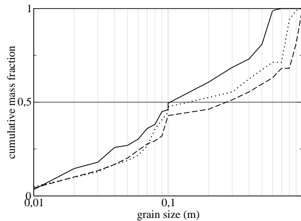
FIGURE 1.13 – Courbe granulométrique dans une section de rivière, à trois instants successifs, dans une simulation de transport lagrangien : on constate l'arrivée progressive des plus gros blocs venus de l'amont et la stabilisation de la quantité des particules plus fines.
