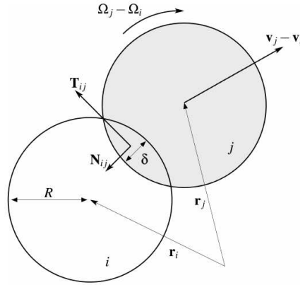
FIGURE 3 – Interactions entre deux particules en contact : forces normale et tangentielle.
