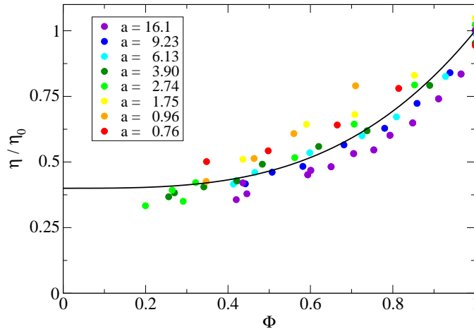
FIGURE 2.8 – Portée normalisée par la portée de l’effondrement granulaire \eta_0 , en fonction du taux de fragmentation observé dans le dépôt final [7].
