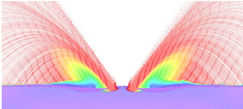
FIGURE 3.9 – Nappe d'éjectats : trajectoire intégrée de toutes les particules éjectées, coloriées selon leur vitesse instantanée. Les lignes plus saturées représentent la forme de la nappe à des instants successifs.
