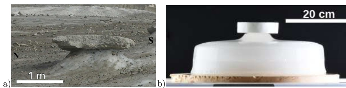
FIGURE 5.10 – Exemples de tables glaciaires suivies (a) sur la Mer de glace et (b) en laboratoire [stage M. Vicet].
