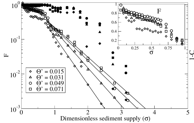
FIGURE 1.10 – Symboles creux : fonction de couverture F définie par l'équation 1.10 ; symboles pleins : fraction « libre » du socle rocheux, 1-C , en fonction de la quantité de sédiments disponibles et pour plusieurs valeurs de l'écart au seuil \Theta' = \Theta - \Theta_c [6].
