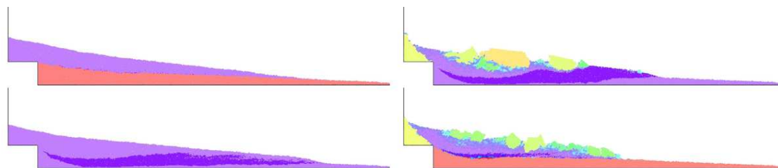
FIGURE 2.10 – Dépôt final observé après l'éboulement d'une colonne sur un substrat érodable (initialement en pente douce). Les particules du substrat ayant été entraînées sont représentées avec une saturation plus importante. L'échelle de couleur donne, comme précédemment, la taille logarithmique des blocs.
