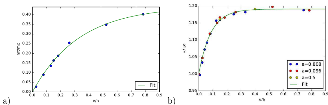
FIGURE 2.11 – a) Masse entraînée par la coulée, rapportée à sa masse « initiale », en fonction de l'épaisseur du substrat érodable. b) Portée de l'éboulement (rapportée au cas d'un effondrement sur socle rigide) en fonction de l'épaisseur du substrat granulaire (rapporté à la hauteur de la colonne) : on observe une saturation exponentielle, quelque soit le rapport d'aspect initial.
