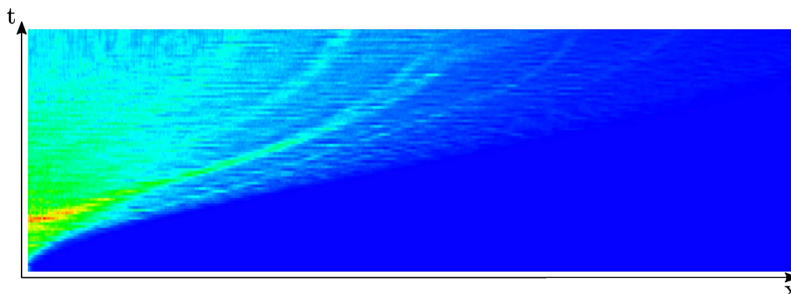
FIGURE 2.9 – Amplitude de la force normale exercée par la coulée sur le sol, en fonction de la distance x au pied de la colonne et du temps.
