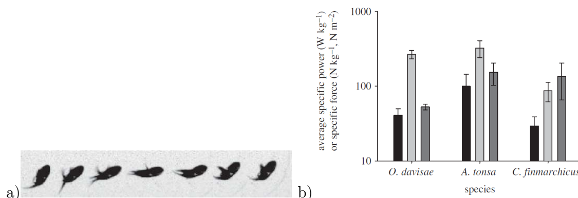
FIGURE 5.14 – a) Détail des étapes du mouvement des pattes pendant un cycle de mouvement de fuite chez un copépode ; b) Puissance et force spécifiques nécessaires à ce mouvement, mesurées chez trois espèces différentes [9].
