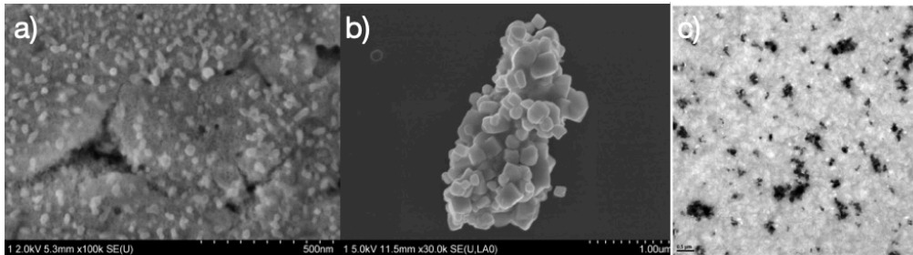
Figure II.9 : Observations de LiNbO 3 et du nanocomposite LiNbO 3 @PVDF-TrFE. Micrographies (a) et (b) MEB de LiNbO 3 pur obtenu à partir de LiH dans le toluène à 110°C, après recuit à 550°C pendant 30 min, et (c) MET de LiNbO 3 @PVDF-TrFE (10 % massique).
