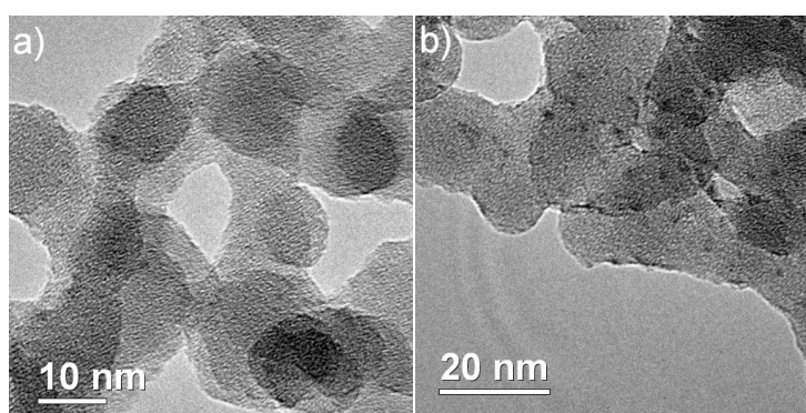
Figure II.6 : Micrographies MET du système Ni(acac)/SiO 2 . (a) après traitement thermique à 600°C sous argon, et (b) après 5 min d'irradiation.
