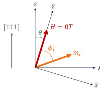
FIGURE 6.22 – Schéma permettant de visualiser l'angle \Phi_i associé à un moment m_i ainsi que l'angle \theta entre les deux repères (x, z) et (\tilde{x}, \tilde{z}) .
