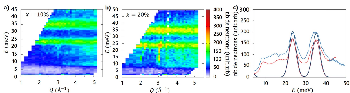
FIGURE 3.6 – (a-b) - Cartes en intensité (nombre de neutrons) de l'énergie E en meV en fonction du paramètre Q en \text{\AA}^{-1} réalisées à 4K pour une énergie incidente de 50meV pour les deux composés dopés : 10% (a) et 20% (b). Les résultats sont soustraits avec les mesures de boîte vide. c - Coupes en moyenne sur l'ensemble des valeurs en Q présentant l'évolution de l'intensité en fonction de l'énergie ainsi que le résultat du fit par le code numérique pour les deux échantillons : 10% (rouge) et 20% (bleue).
