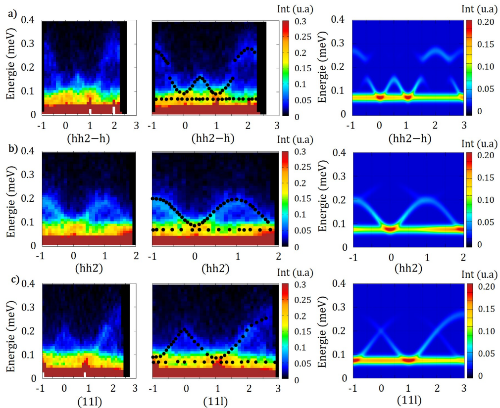
FIGURE 5.11 – Coupes en énergie à une température de 45mK selon trois axes de coupe : (hh2-h) (a), (hh2) (b) et (111) (c). À gauche se situe la coupe issue des cartes en énergie, au centre les mêmes coupes avec le fit manuel de la branche plate et des branches dispersives, et enfin, à droite, le résultat des simulations numériques pour le jeu de paramètres d'échange retenus pour le composé dopé 2.5%.
