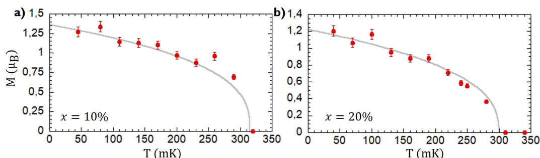
FIGURE 4.8 – Résultats des moments magnétiques affinis par le logiciel FullProf en fonction de la température à partir des mesures sur poudre pour le composé 10% (a) et 20% (b). La ligne grise est un guide pour les yeux tandis que les points rouges sont les résultats de ces affinements.
