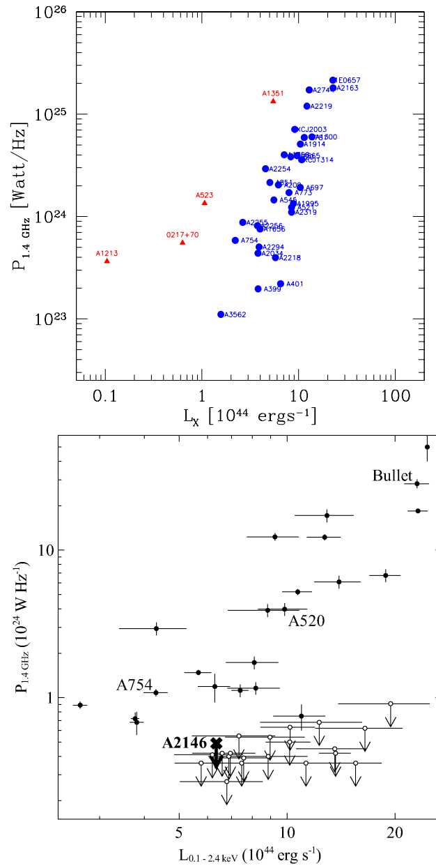
Figure 2.13 – Images extraites de Giovannini et al. (2011) (à gauche) et Russell et al. (2011) (à droite) qui montrent la corrélation entre la luminosité à 1.4 GHz des halos connus et la luminosité X de leurs amas hôtes. Dans le panneau de droite les triangles rouges indiquent la position de halos radio découverts récemment ( Giovannini et al. 2011 , et références incluses). Les flèches dans le panneau de droite correspondent à des limites supérieures de la luminosité radio de plusieurs amas estimées par Brunetti et al. (2007) . La croix montrée dans le cas d’A 2146 indique en revanche la valeur de P_{1.4 \text{ GHz}} obtenue récemment par Russell et al. (2011) . Voir texte pour plus de détails.
