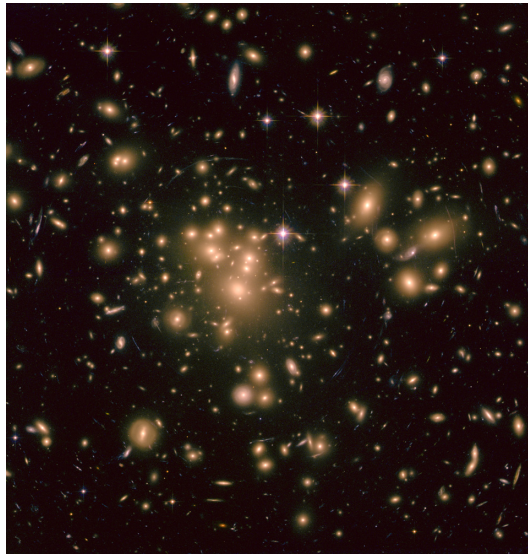
Figure 1.37 – Image de l’amas A1689 observé par le télescope spatial Hubble qui montre des exemples spectaculaires d’arcs gravitationnels : le potentiel gravitationnel des amas donne lieu aux plus grands effets de déflexion de la lumière (avec des angles de déflexion de l’ordre de la moitié d’un minute d’arc), en produisant les plus spectaculaires effets de lentille gravitationnelle de l’Univers (e.g. Hattori et al. 1999). On remarque aussi que la majorité des galaxies appartenant à l’amas sont caractérisées à peu près par la même couleur (voir aussi panneau de droite de Fig. 1.36). (Crédits : NASA, ESA, E. Jullo, Jet Propulsion Laboratory ; P. Natarajan, Yale University ; J.-P. Kneib, Laboratoire d’Astrophysique de Marseille, CNRS, France).
