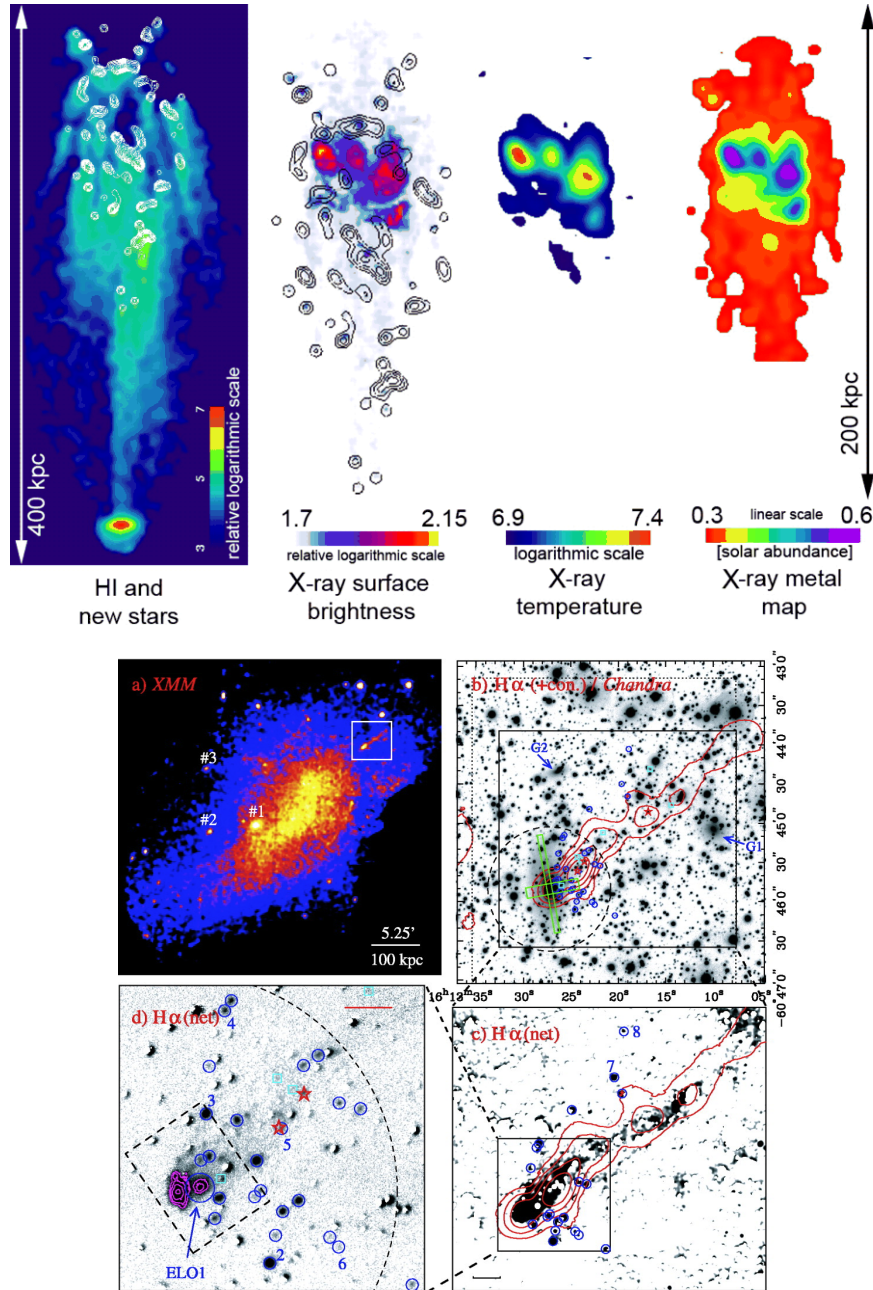
Figure 2.4 – En haut : distribution simulée du gaz chaud (observable en X) et froid (observable à 21 cm), ainsi que des régions de formation stellaire, pour une galaxie qui bouge avec v_{gal} = 1000 km/s depuis 500 millions d’années à l’intérieur d’un amas avec densité du gaz de 1 \times 10^{-27} g cm ^{-3} (Kapferer et al. 2009). En bas : image en bande X (a) et images dans le filtre H_{\alpha} avec contours d’émission X (b,c,d) pour l’amas de galaxies A3627 (la taille du champ montré diminue progressivement du panneau en haut à gauche au panneau en bas à droite, Sun et al. 2007). Nous observons clairement des régions de formation stellaire (émission H_{\alpha} ) dans une longue ( \approx 100 kpc) queue de gaz chaud associée à une galaxie qui est en train de tomber vers le centre de l’amas.
