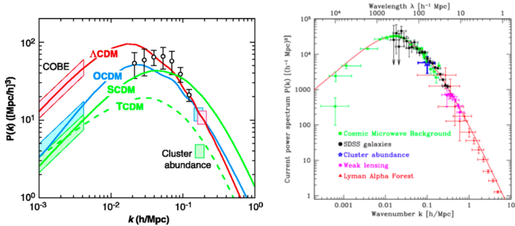
Figure 1.7 – À gauche : les courbes de cette figure (extraite de 1999) montrent le spectre de puissance des fluctuations prévu par différents modèles (voir texte) et normalisé en utilisant les observations du CMB , les comptages de galaxies et l’abondance d’amas à z \sim 0 . À droite : des résultats observationnels plus récents sont disponibles (Tegmark 2002; Tegmark et al. 2004). Les paramètres obtenus par Tegmark et al. (2004) correspondent à un Univers plat, avec h\Omega_m = 0.213 \pm 0.023 , \sigma_8 = 0.89 \pm 0.02 et h = 72 \text{ km s}^{-1} \text{ Mpc}^{-1} .
