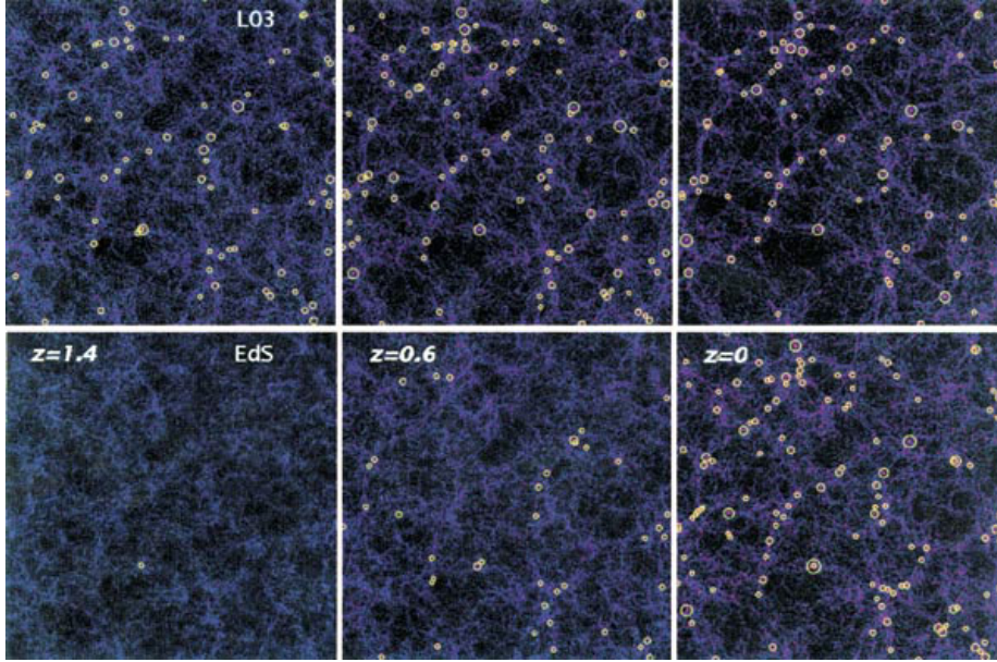
Figure 1.9 – Figure extraite de Borgani & Guzzo (2001) qui montre l'évolution de la population d'amas dans depuis des simulations numériques à N-corps basées sur deux différents modèles cosmologiques. En haut : modèle avec \Omega_m = 0.3 et \Omega_\Lambda = 0.7 . En bas : modèles EdS ( \Omega_m = 1 et \Omega_\Lambda = 0.3 ). Dans les deux cas, les paramètres des simulations ont été choisi pour arriver approximativement à la même densité spatiale d'amas à z = 0 . La largeur et l'épaisseur comobiles des boîtes sont de 250 h^{-1} Mpc et 75 h^{-1} Mpc. Les images montrent la distribution de matière noire, les cercles indiquent la position des amas massifs.
