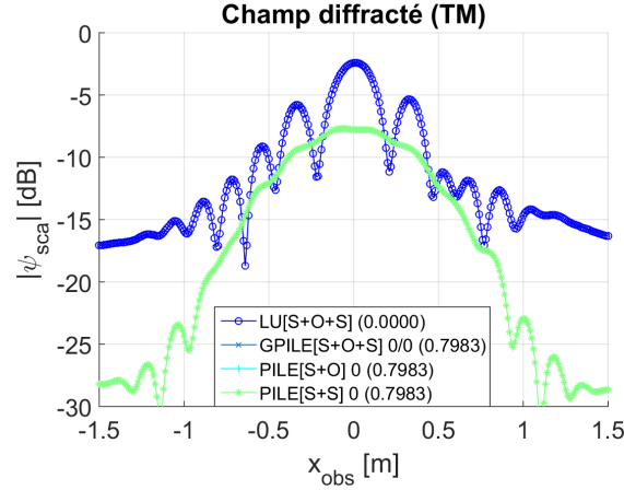
FIGURE 2.10 – Module des champs diffractés en décibels ( 10 \log_{10} |\psi_{\text{sca}}| ) par rapport à l'abscisse d'observation ( x_{\text{obs}} \in [-L/2; L/2] ) et pour une hauteur d'observation z_{\text{obs}} = 470 mm. Les paramètres de surfaces sont les mêmes que dans la figure 2.2. L'onde incidente est une onde de Thorsos avec les mêmes paramètres que dans la figure 2.3. L'ordre P = 0 .
