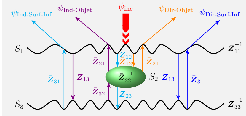
FIGURE 2.9 – Représentation graphique des contributions de l’objet et de la surface inférieure. Les contributions directe et indirecte de l’objet sont respectivement notées : \psi_{\text{Dir-Objet}} et \psi_{\text{Ind-Objet}} . Celles de la surface inférieure sont respectivement notées : \psi_{\text{Dir-Surf-Inf}} et \psi_{\text{Ind-Surf-Inf}} .
