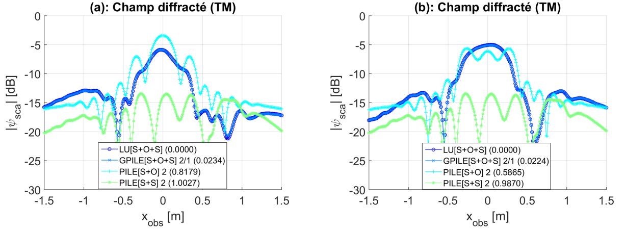
FIGURE 2.15 – Module des champs diffractés en décibels ( 10 \log_{10} |\psi_{sca}| ) par rapport à l'abscisse d'observation ( x_{obs} \in [-L/2; L/2] ) et pour une hauteur d'observation z_{obs} = 470 mm. Les paramètres de surfaces sont les mêmes que dans la figure 2.2, excepté l'épaisseur entre les deux surfaces H = 240 mm. L'onde incidente est une onde de Thorsos avec les mêmes paramètres que dans la figure 2.3. Les ordres P = 2 et Q = 1 . Les dimensions du cylindre elliptique sont a = 100 mm et b = 10 mm. Le centre du cylindre varie. (a) C = (0, -0.1H) . (b) C = (0, -0.15H) .
