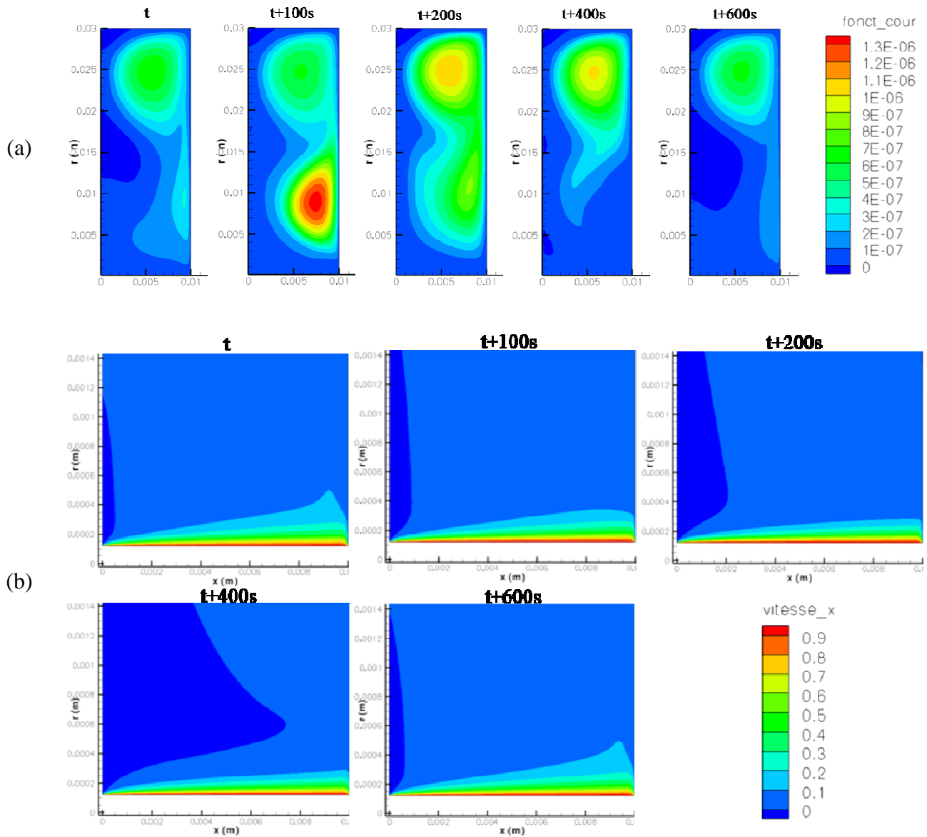
Figure 4-3 – Evolution au cours du temps (a) de la fonction courant pour le plomb-étain et (b) de la couche limite
