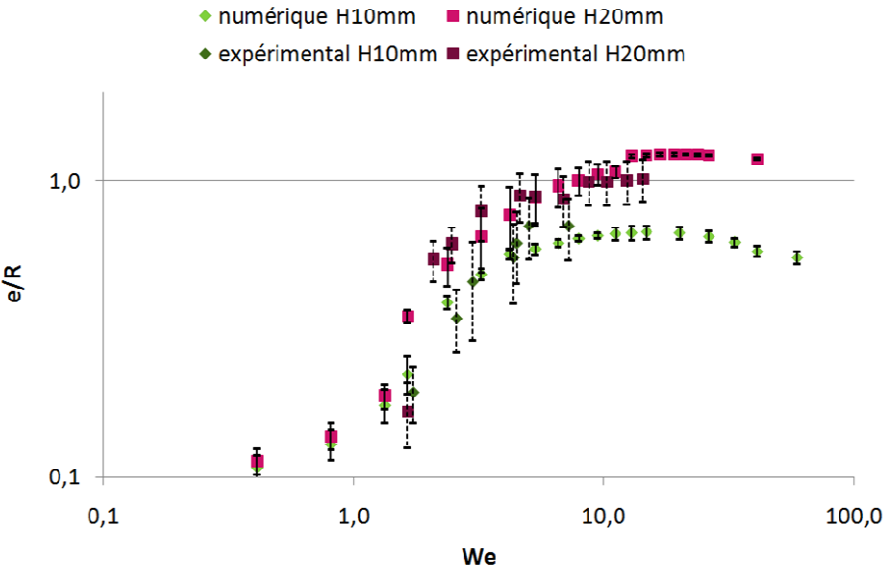
Figure 4-1 – Influence de la profondeur du bain sur l'épaisseur adimensionnée emportée
