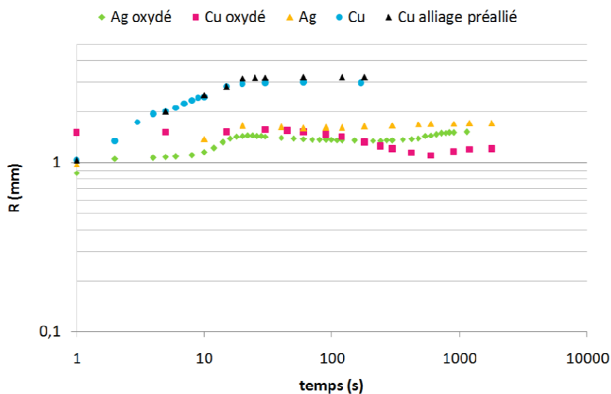
Figure 4-13 – Etalement de l'eutectique pur ou pré-allié sur différents substrats en fonction du temps
