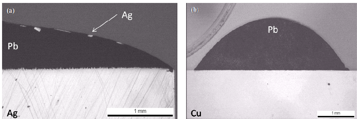
Figure 4-8 – Mouillage (a) de l'argent et (b) du cuivre par du plomb pur
