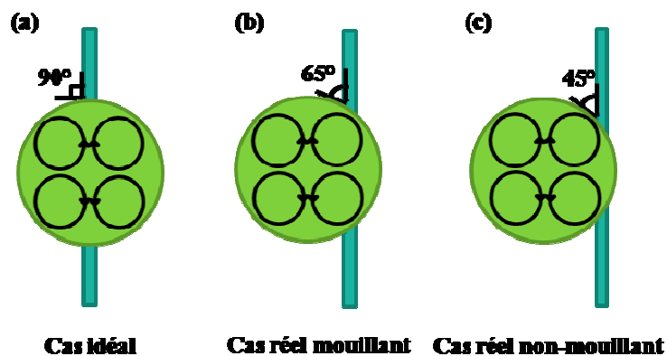
Figure 5-1 – Angle d'induction liés au mouillage filament/alliage et flux induit par le champ électromagnétique
