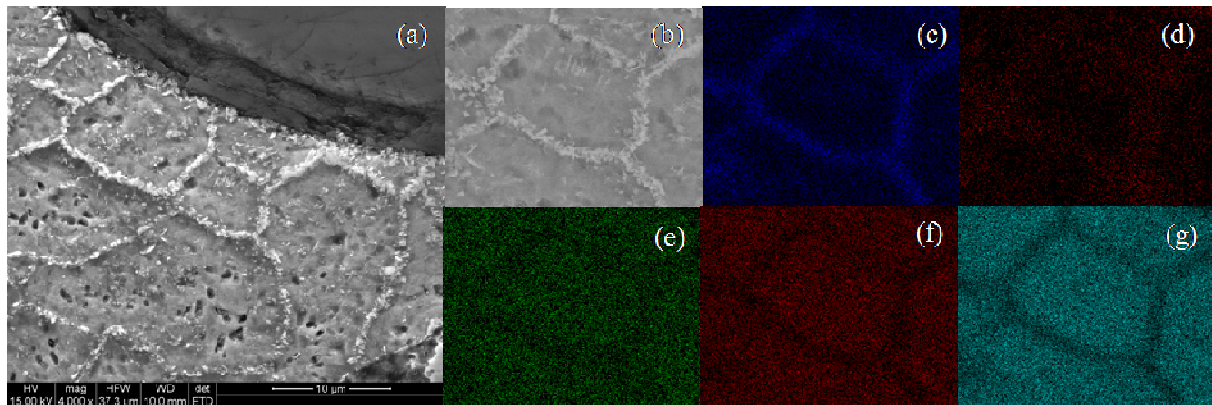
Figure 0-15 – Analyse de l’interphase : (a) vue d’ensemble de l’interphase, (b) vue de la zone analysée et répartition des espèces chimiques dans la zone (c) élément carbone, (d) élément zirconium, (e) élément aluminium, (f) élément vanadium et (g) élément titane.
