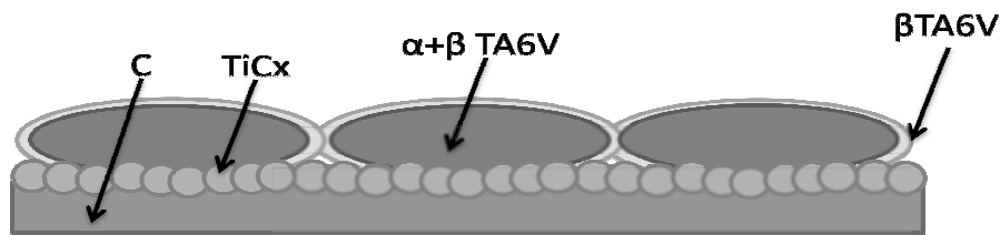
Figure 5-6 – Description des grains de matrice de TA6V
