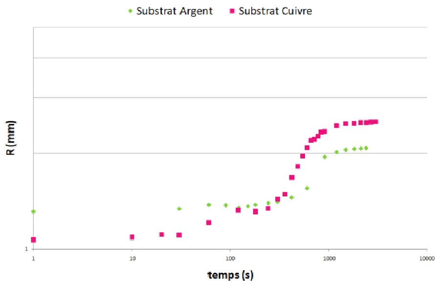
Figure 4-11 – Etalement (R) de l'étain pur sur un substrat de cuivre et d'argent en fonction du temps
