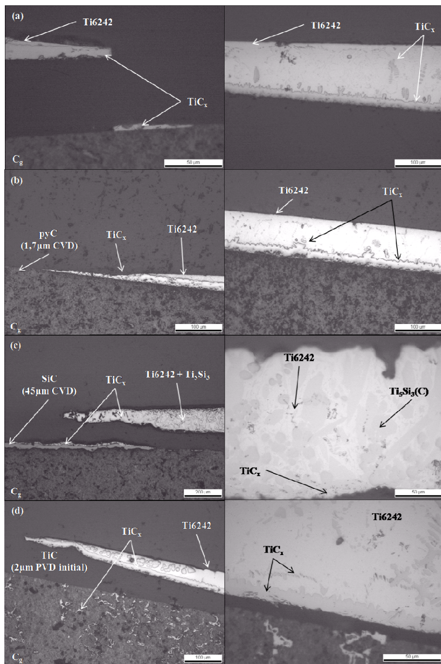
Figure 0-6 - Coupe et observation post-mortem du mouillage du Ti6242 sur différents substrats céramiques : (a) sur du carbone graphite, (b) sur du carbone graphite initialement couvert de pyrocarbone, (c) sur du carbone graphite initialement couvert de carbure de silicium et (d) sur du carbone graphite initialement couvert de carbure de titane
