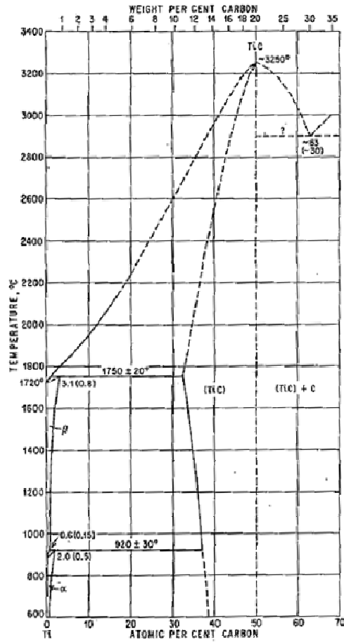
Diagramme binaire C-Ti
