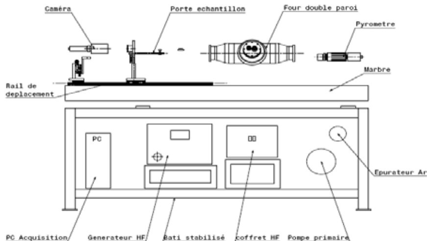
Figure 2-14 – Schéma technique du four Haute Température réalisé [GUI10]
