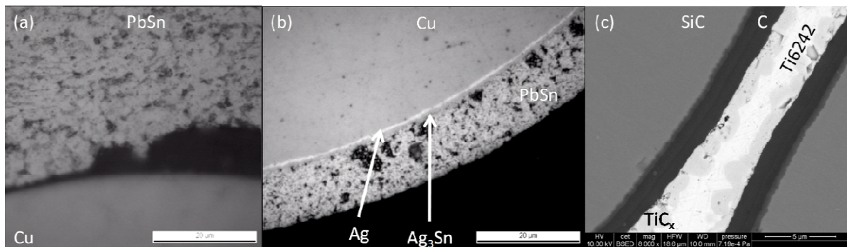
Figure 4-17 – Zones interfaciales (a) d'un filament de cuivre traité gainé de PbSn_E , (b) d'un filament de cuivre couvert d'argent gainé de PbSn_E et (c) comparaison avec un filament SCS-6 gainé de Ti6242
