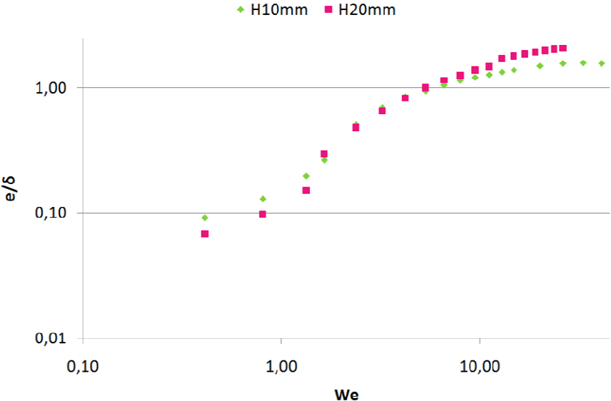
Figure 4-2 – Epaisseur emportée adimensionnée par le paramètre de couche limite en fonction du nombre de Weber
