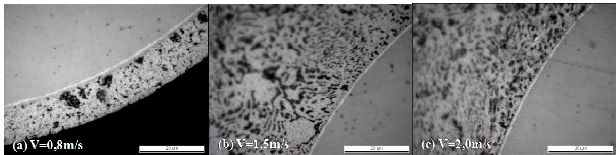
Figure 4-16 - Enduction de filaments argentés traités en série pour un bain de plomb-étain de H=20mm à 200°C
