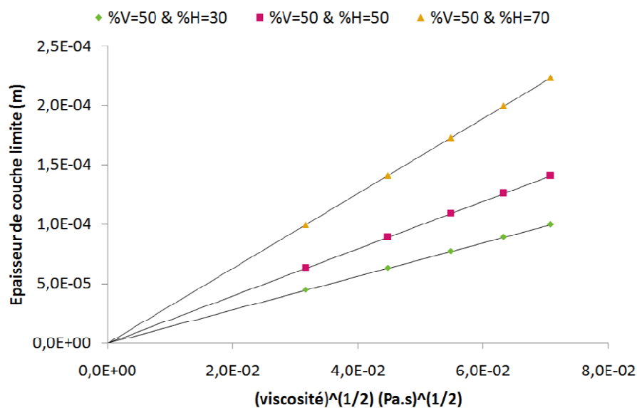
Figure 4-1 – Influence de la viscosité sur l'établissement de la couche limite
