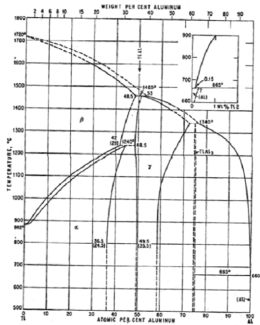
Diagramme binaire Al-Ti
