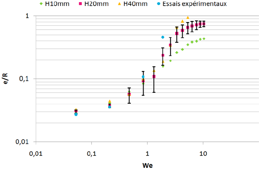
Figure 5-2 – Evolution de l’épaisseur emportée de titane adimensionnée par le rayon du filament en fonction du nombre de Weber
