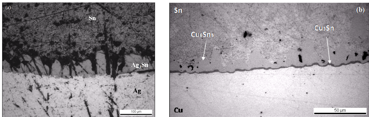
Figure 4-10 - Mouillage (a) de l'argent et (b) du cuivre par de l'étain pur
