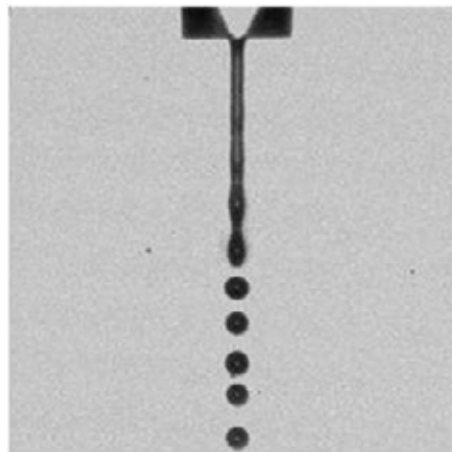
Figure 1-14 – Représentation des déstabilisations du mode Rayleigh
