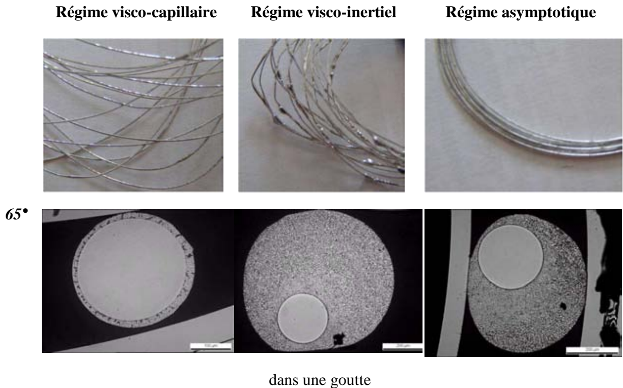
Figure 4-21 - Gaine d'eutectique et régimes d'enduction
