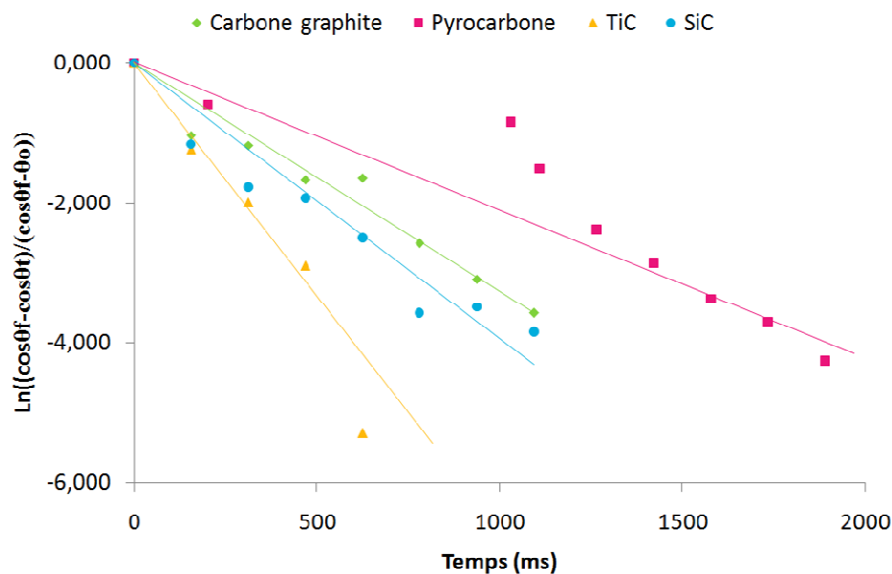
Figure 0-7 – Logarithme Néperien de (\cos\theta_F - \cos\theta_t)/(\cos\theta_F - \cos\theta_0) en fonction du temps pour les différents substrats céramiques
