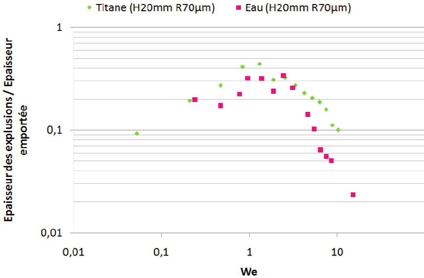
Figure 5-3 – Evolution de la taille des excroissances expulsées adimensionnée par l’épaisseur moyenne emportée en fonction du nombre de Weber
