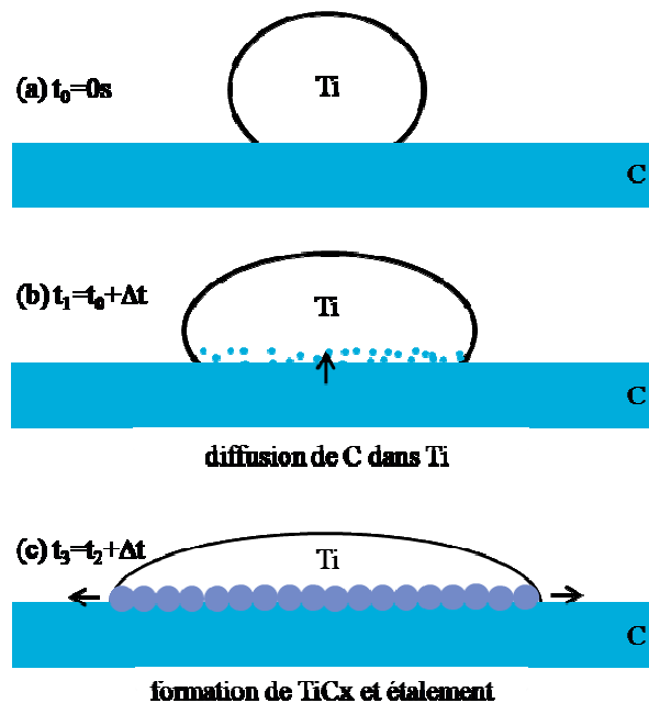
Figure 1-20 – Quelques étapes du mouillage du carbone par un alliage de titane : (a) premier temps de contact, (b) diffusion du substrat dans le liquide et (c) mouillage par formation d'un produit interfacial
