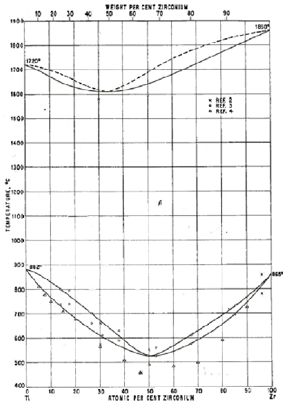
Diagramme binaire Ti-Zr
