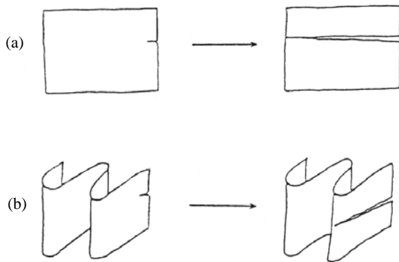
Figure. I.37: Modes de fracture pour 2 fibres ex-Brai (a) plans droits, (b) plans pliés [Endo, 1988].
