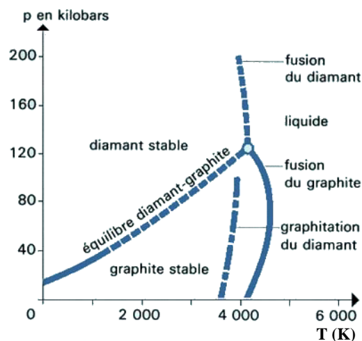
Figure I.2: Diagramme de phase du carbone
