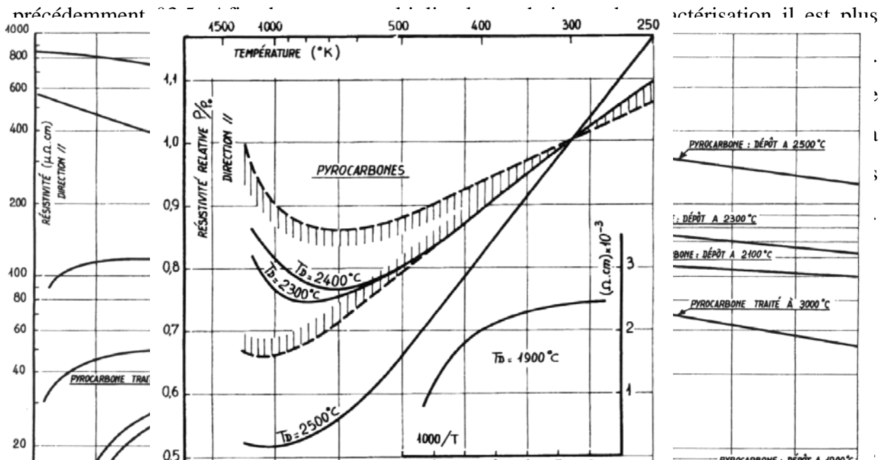
Figure. I.62: Evolution de la résistivité longitudinale à haute température pour différents pyrocarbones (élaborés à différentes températures) [Klein, 1962b].
