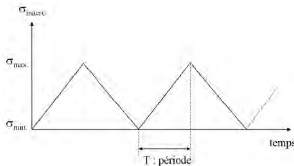
FIG. 5.5 – Schéma du chargement macroscopique axial cyclique appliqué à la cellule périodique ( f = \frac{1}{T} et R_\sigma = \frac{\sigma_{min}}{\sigma_{max}} ).
