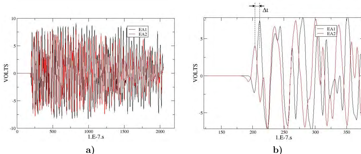
FIG. 3.3 – Illustration de l'enregistrement d'un évènement acoustique durant un essai, avec les signaux issus des deux capteurs. En a) : ensemble de l'échantillon de signal enregistré ; en b) : zoom sur le début de l'enregistrement où est indiquée une lecture visuelle du décalage entre les signaux.
