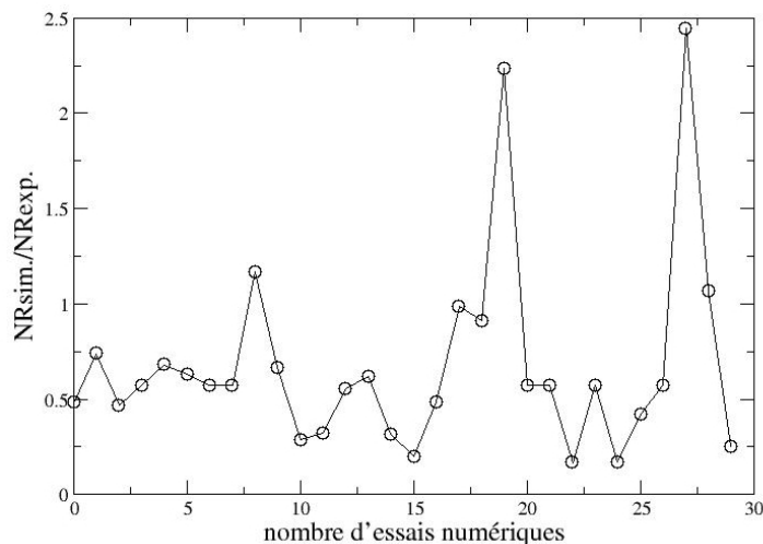
FIG. 5.32 – Durées de vie obtenues par la simulation normées par la durée de vie expérimentale. Trentes essais numériques. \sigma_{max}=1100 MPa, T=350^{\circ}\text{C} , f_{\text{experimentale}}=5 Hz, f_{\text{simulation}}=1 Hz ; 100 fibres, longueur de jauge = 13 mm, Vf=20%.
