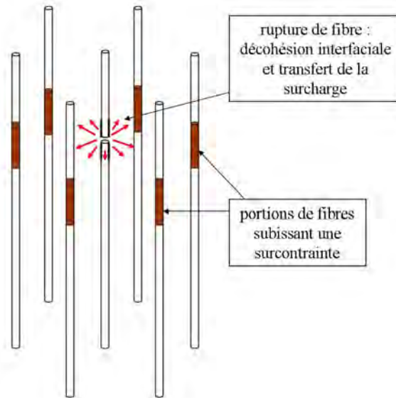
FIG. 2.5 – Schéma illustrant le transfert de charge associé à la rupture d'une fibre. Les fibres voisines de la rupture subissent une surcontrainte.
