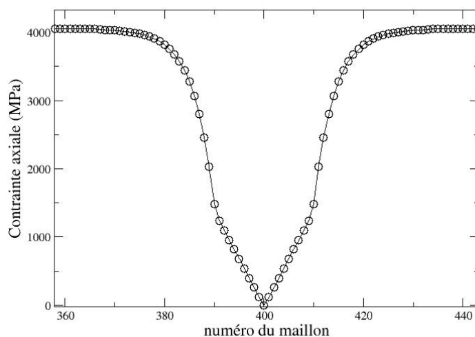
FIG. 3.36 – Détail du champ de contrainte axial au voisinage d'une rupture avec la discrétisation adoptée. Les zones linéaires associées à la décohésion et les zones non linéaires sont bien reproduites par rapport aux profils des simulations EF.
