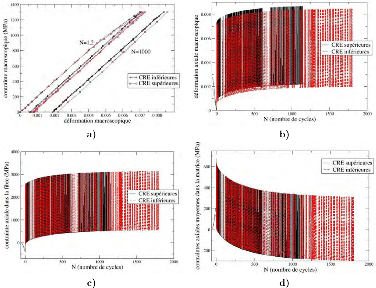
FIG. 5.11 – Comparaison des réponses cycliques du composite et de ses constituants pour deux intensités du champ de contraintes résiduelles. \sigma_{max}=1300 MPa, T=450^{\circ}\text{C} , V_f=35\% , vitesse de chargement de 13 MPa/s.
