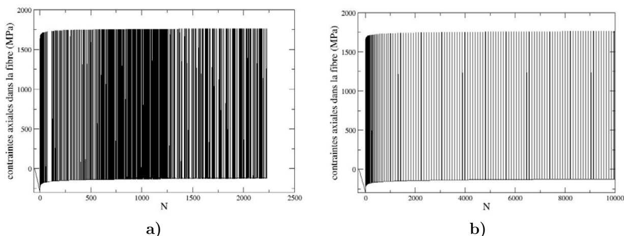
FIG. 5.18 – Évolution des contraintes axiales moyennes dans la fibre en fonction du nombre de cycles pour deux vitesses de chargement : \sigma_{max}=950 MPa, Vf=35\% , 450^\circ\text{C} . En a) : 10 MPa/s., en b) : 95 MPa/s..
