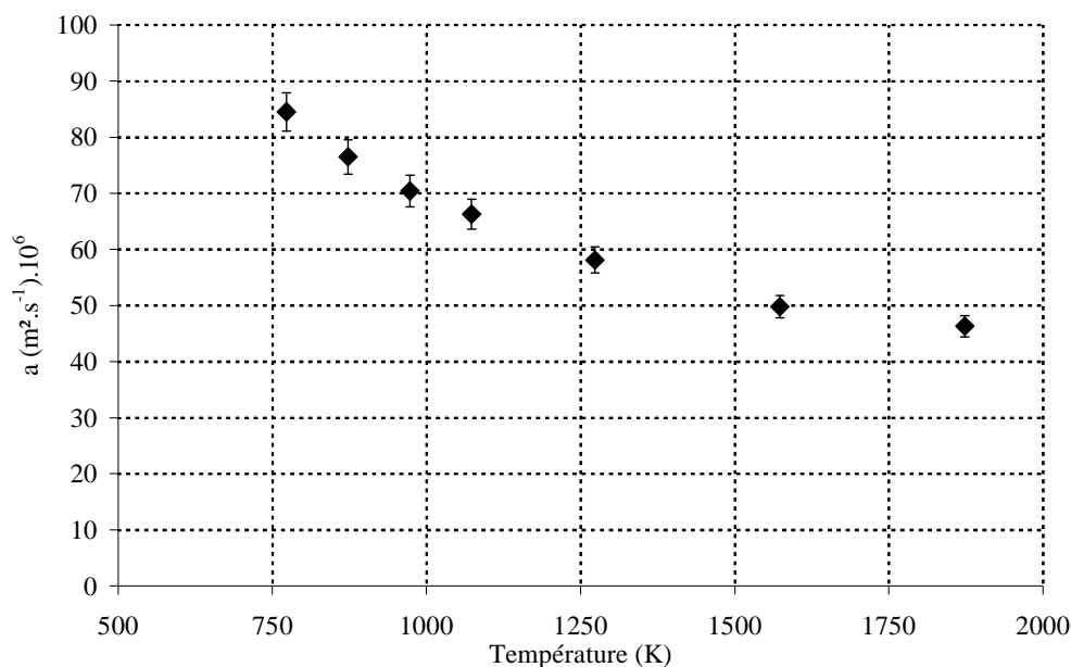
figure 6.30 : Mesure de la diffusivité thermique longitudinale de la fibre P100 brute.
