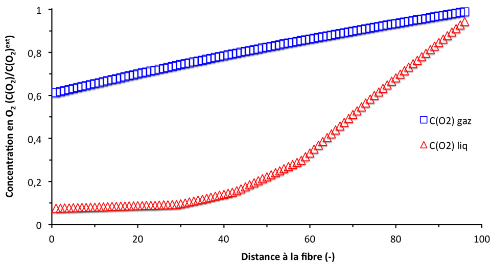
Figure II.6 – Quantité d'oxygène présent dans la fissure, initialement remplie de gaz (bleu) puis lorsque l'oxyde a totalement bouché la zone considérée (rouge) - (à titre de schéma, valeurs arbitraires)
