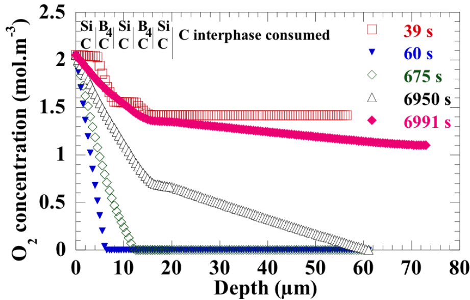
Figure I.26 – Profil de la concentration en O_2 dans la fissure pour un composite SiC/C/SiC/(SiC/B 4 C/SiC/B 4 C/SiC) à 900 °C [Rebillat 04a]
