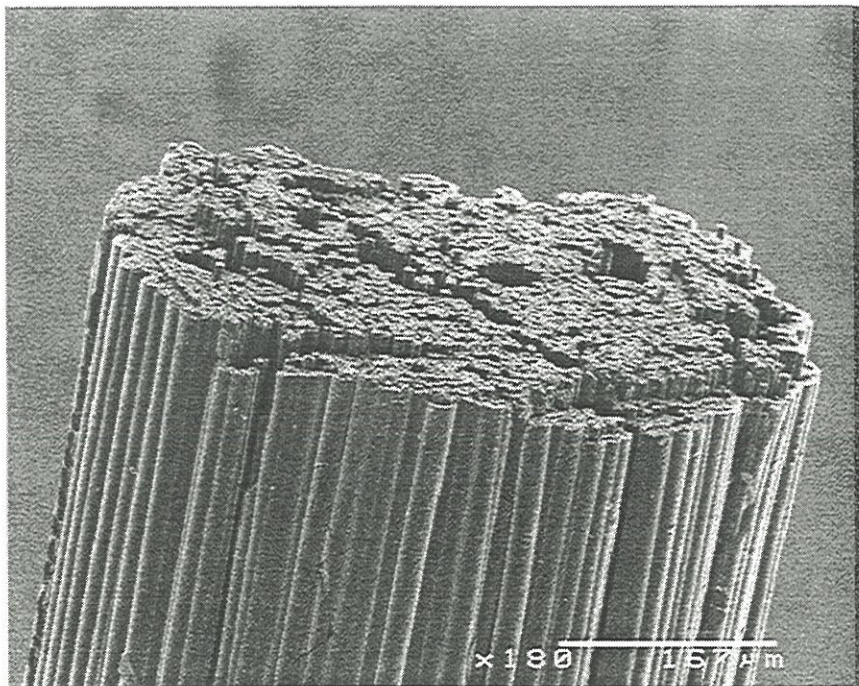
Figure 41: faciès de rupture plat pour le minicomposite A/M
