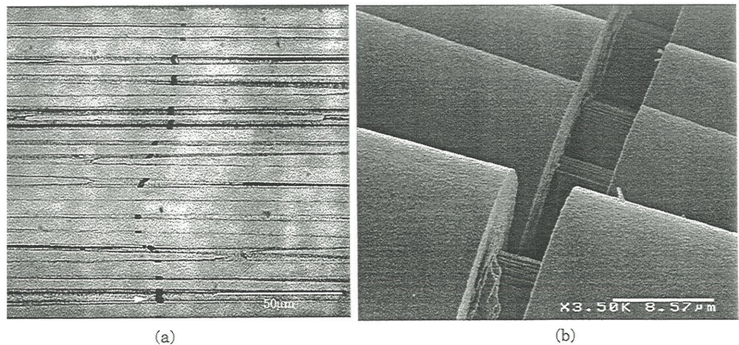
Figure 44: fissuration matricielle (a) vue en microscopie optique d'un minicomposite A-HTT/M en coupe longitudinale polie (déviation de la fissure à l'interface fibre/matrice); (b) d'un minicomposite A-HTT 1 /M vu au MEB à plus fort grandissement (pontage des fissures par les fibres)
