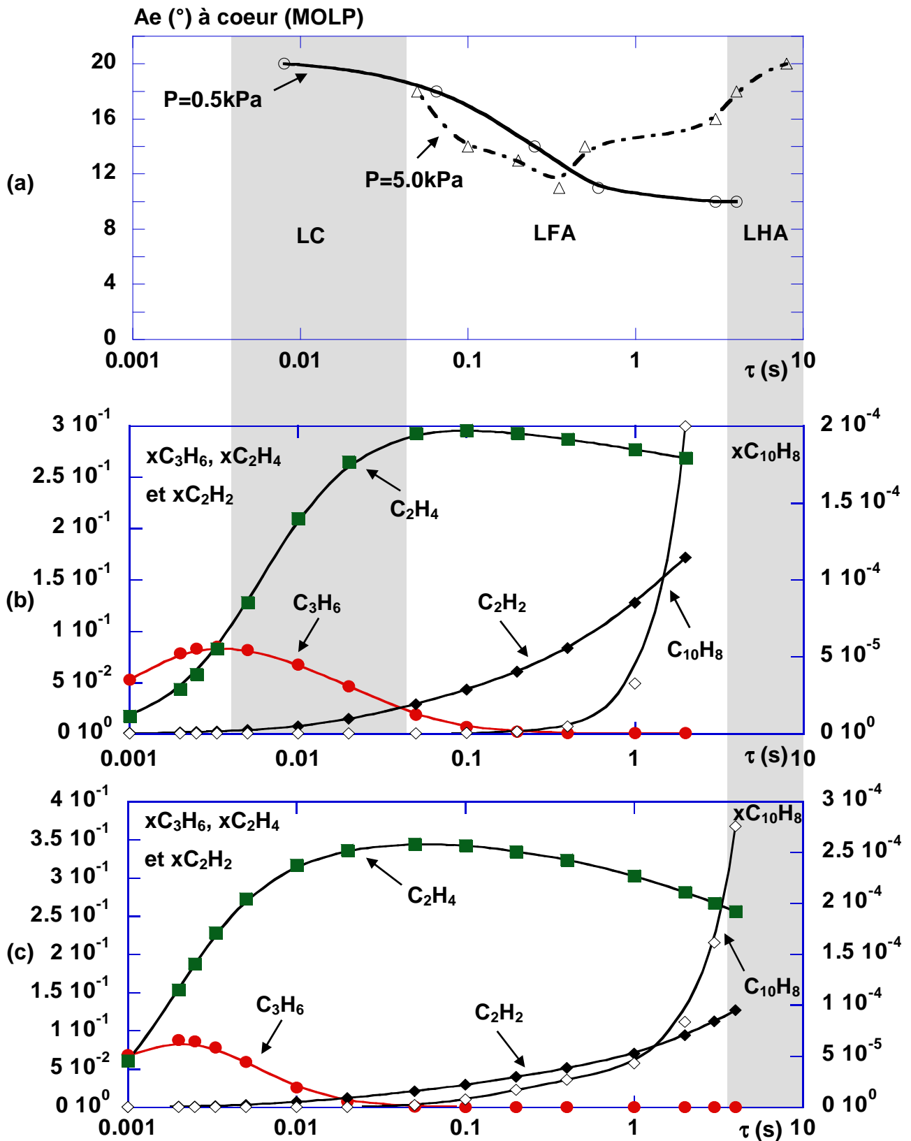
Figure 3-14 : Corrélation entre (a) l'angle d'extinction à cœur de préforme déterminé par MOLP (d'après [Le Poche, 2003]) et les fractions molaires de propylène, d'éthylène, d'acétylène et de naphthalène calculées pour T=950^\circ\text{C} à (b) P=0,5\text{kPa} et (c) 5,0\text{kPa} – Etude en fonction du temps de passage à partir du précurseur propane
