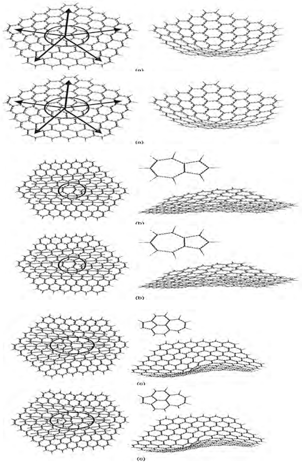
Figure 3-18 : Défauts de structure résultant (a) d'un cycle à 5 isolé entouré de cycles à 6 (la symétrie C_5 est représentée par les flèches), (b) d'un cycle à 5 en voisinage direct avec un cycle à 7 et (c) d'un cycle à 5 en voisinage indirect avec un cycle à 7 (séparés par une unité type naphthalène) – d'après Dong et Hüttinger [Dong et Hüttinger, 2002]
