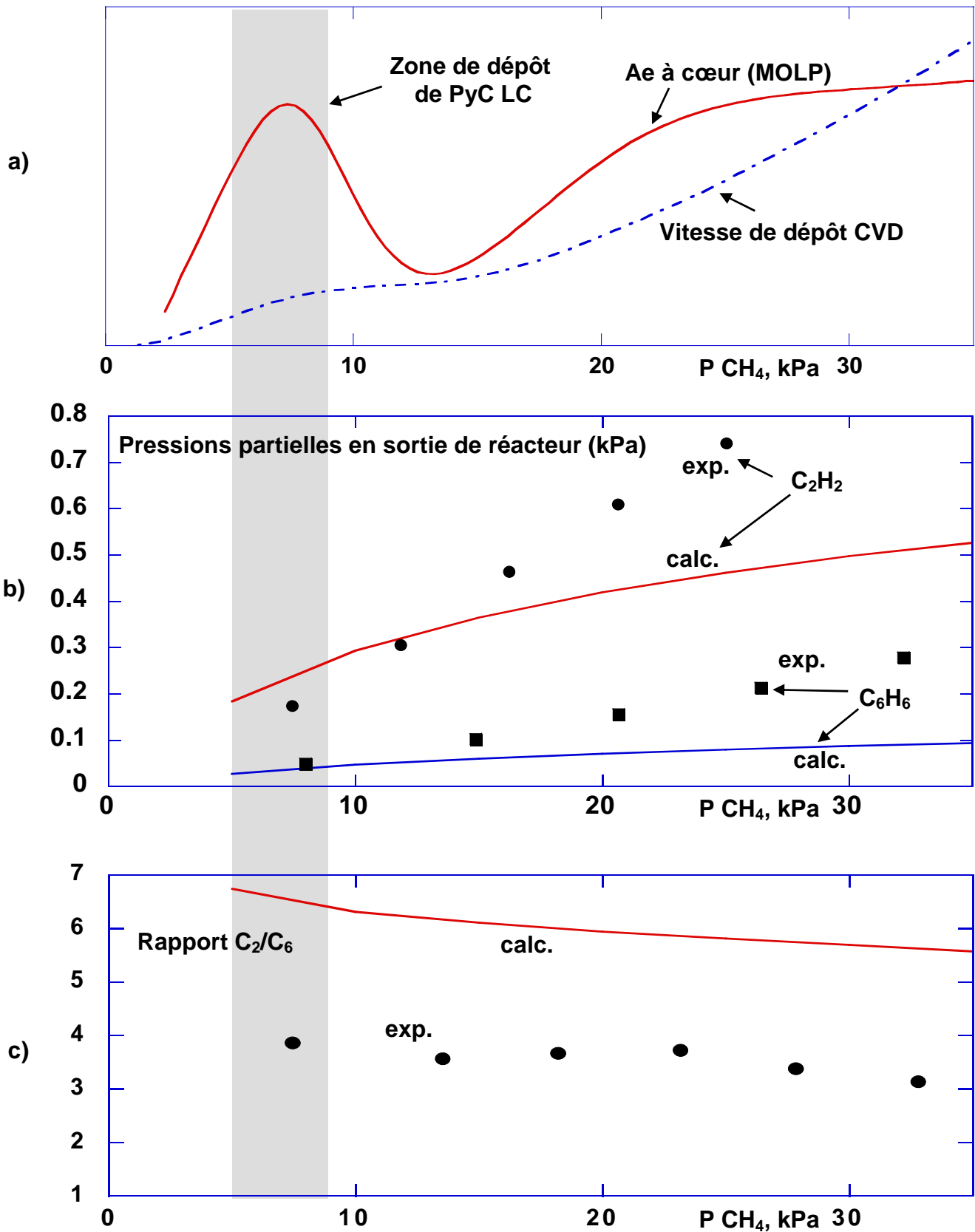
Figure 3-13 : Confrontation entre le rapport C 2 /C 6 expérimental [Becker et Hüttinger, 1998C] et calculé [cette étude], l'angle d'extinction à cœur de préforme et la vitesse de dépôt CVD déterminés par Guellali [Guellali et al., 2002] – Etude en fonction de la pression initiale de méthane
