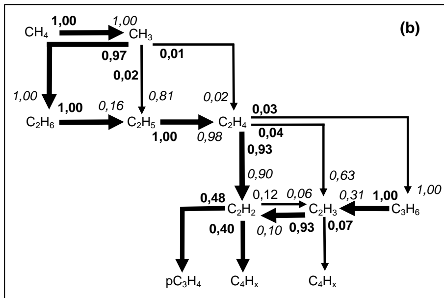
Figure 3-10 : Flux réactionnels pour la décomposition (a) du propane ( T=950^{\circ}\text{C} et P=0,5\text{kPa} ) et (b) du méthane ( T=1100^{\circ}\text{C} et P=10\text{kPa} avec P_{\text{totale}}=100\text{kPa} )
