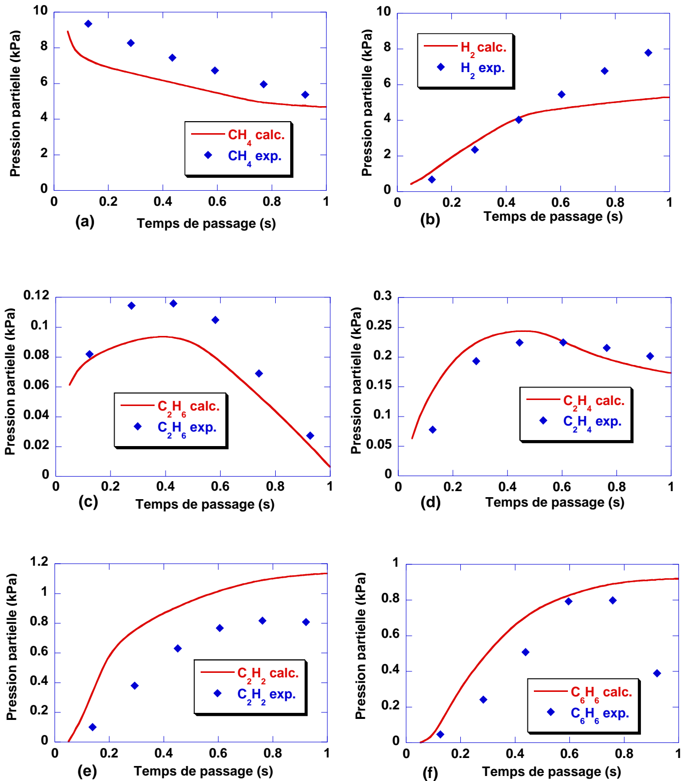
Figure 3-9 : Comparaison de la composition de la phase gazeuse en sortie de réacteur : Modélisation 1D ( Kinvf ) / analyse CPG [Becker et Hüttinger, 1998C] – Pyrolyse du méthane \tau = 0,05 à 1,0s pour T = 1100^\circ\text{C} , P_{\text{CH}_4} = 10\text{kPa} et P_{\text{totale}} = 100\text{kPa}
