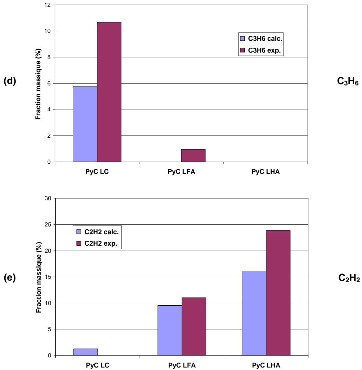
Figure 3-6 : Comparaison de la composition de la phase gazeuse en sortie de réacteur : modélisation 1D ( Kinvf ) / analyse CPG – (d) C 3 H 6 et (e) C 2 H 2 – Conditions de pyrolyse des dépôts LC, LFA et LHA
