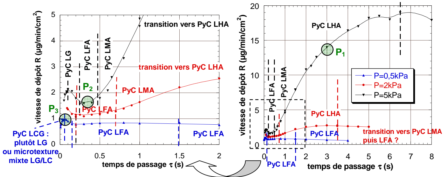
Figure 2-2 : Corrélation entre cinétique de dépôt (prise de masse) et microtexture pour la CVD du PyC en fonction du temps passage, à partir du précurseur propane et pour T = 950^{\circ}\text{C} d'après Le Poche [Le Poche, 2003] – Conditions retenues dans la présente étude (P1, P2 et P3)
