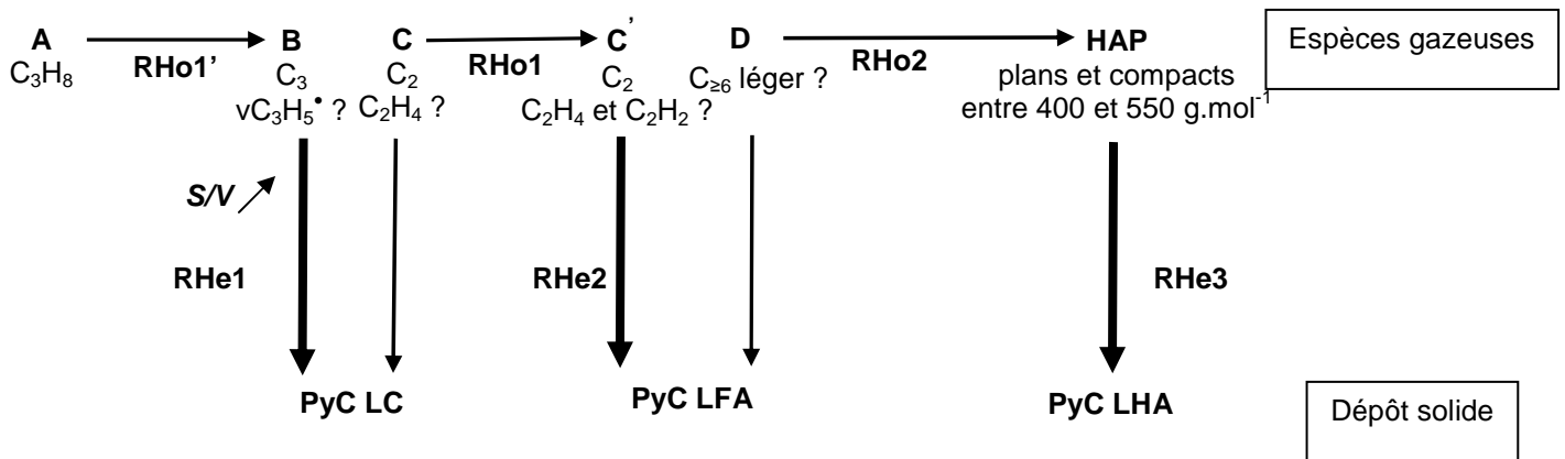
Schéma 4-1 : Modèle qualitatif de formation des pyrocarbones laminaires obtenus en CVD et CVI, à partir du précurseur propane, aux environs de 950°C et à pression réduite ( \leq 5\text{kPa} ) – L'épaisseur des flèches est représentative de la contribution des réactions hétérogènes associées aux précurseurs effectifs
