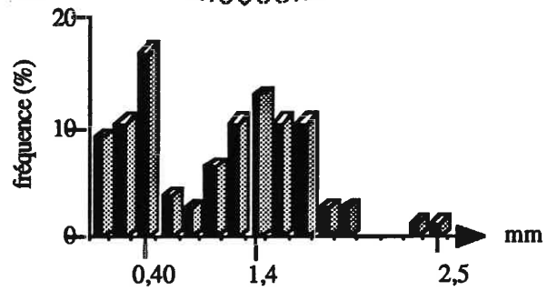
b) Déformation = 0,06 %
