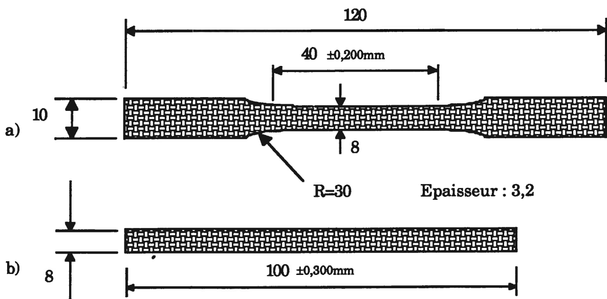
Figure 1. Eprouvetttes utilisées pour les essais : a) de traction b) de flexion.
