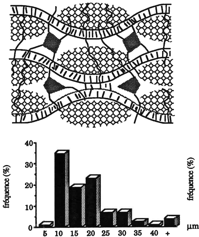
c) Déformation = 0,6 %
