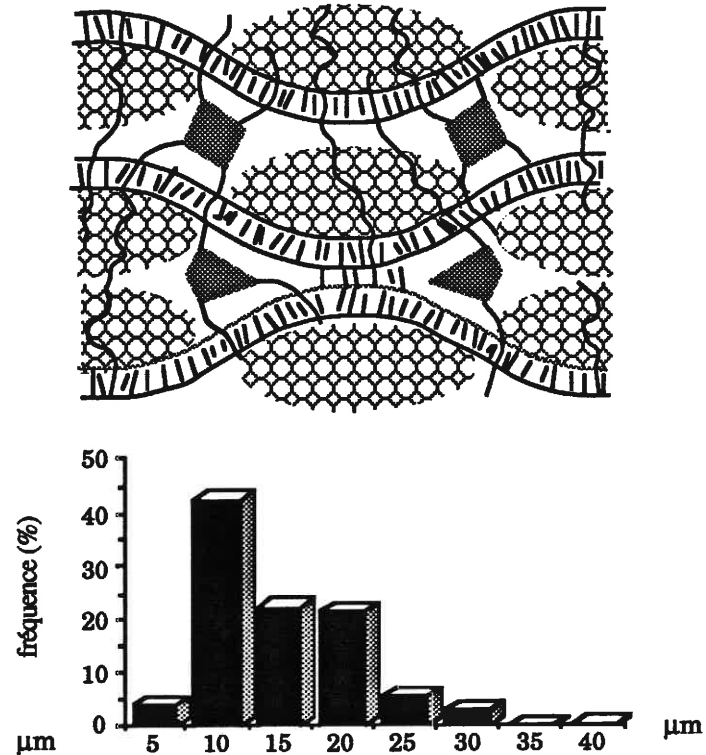
b) Déformation = 0,4 %
