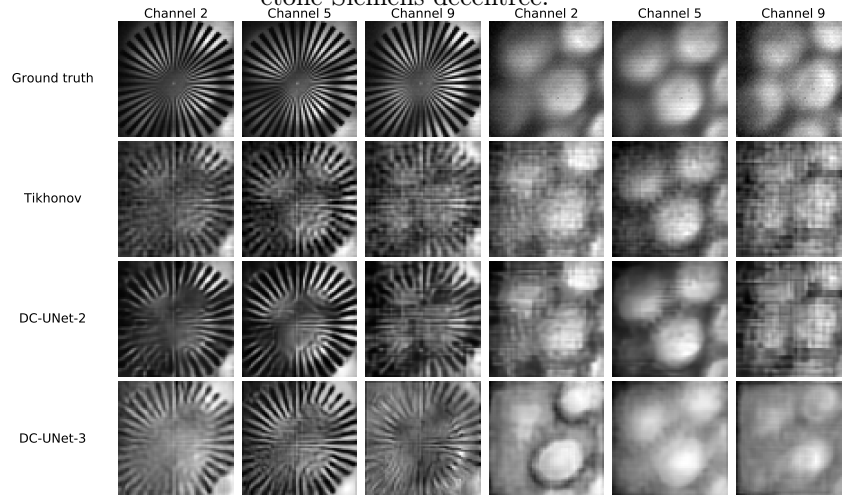
(b) Reconstruction de deux images expérimentales - cible étoilée Siemens centrée et lampe LED.
