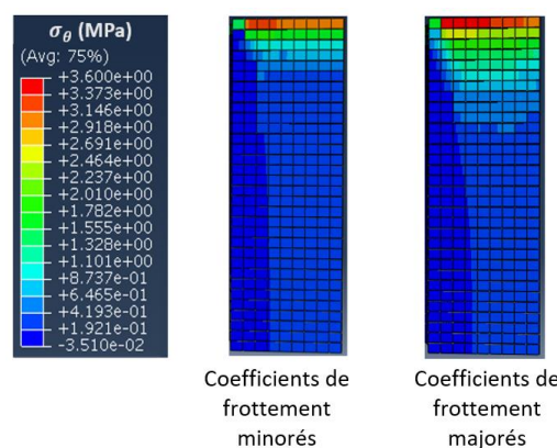
Figure III- 10 - Répartition de la contrainte mécanique (Abaqus) selon la direction u_\theta en fonction des coefficients de frottement minorés et majorés- contrainte globale théorique de 4MPa
