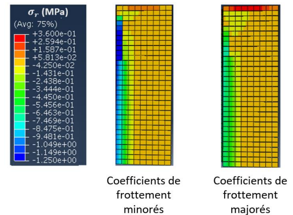
Figure III- 9 - Répartition de la contrainte mécanique (Abaqus) selon la direction u_r en fonction des coefficients de frottement minorés et majorés - contrainte globale théorique de 4MPa
