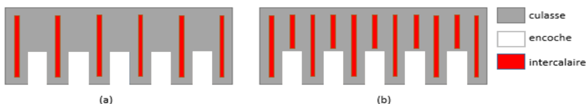
Figure III- 2 - Vue de dessus d’un stator déroulé d’un stator JEUMONT Electric - intercalaires au niveau des dents (a) et intercalaires au niveau des dents et des encoches (b)
