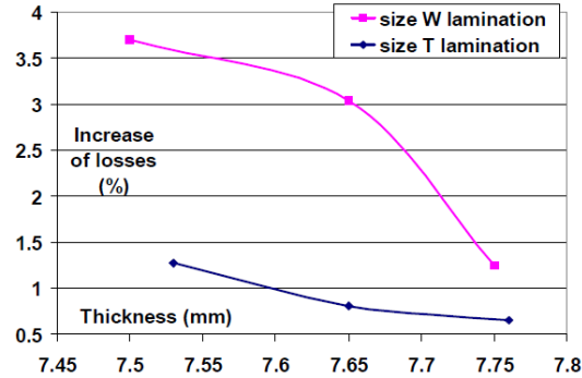
Figure II- 25 - Effet de l'effort de compactage sur les pertes Fer de stators de largeurs différentes (size W > size T) [29]
