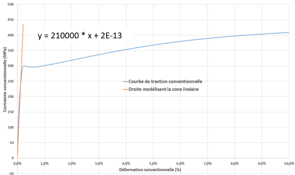
Figure V- 34 - Courbe de traction conventionnelle (bleue) et modélisation de la zone linéaire (orange) par \sigma_m = E\varepsilon_m
