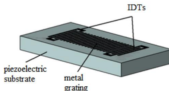
Figure1-21 Schéma d'un dispositif STW (Rocha-Gaso et al. 2009)
