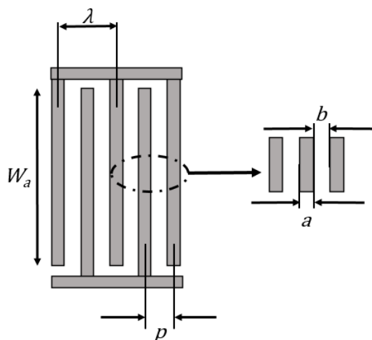
Figure 3-1 Schéma des électrodes interdigitées
