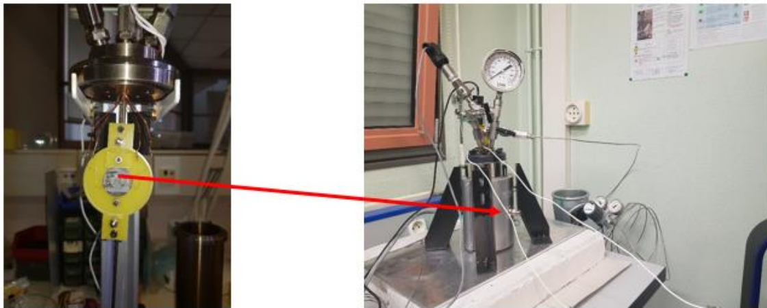
Figure 5-11 Capteur SAW de pression à l'intérieur de l'enceinte de pression
