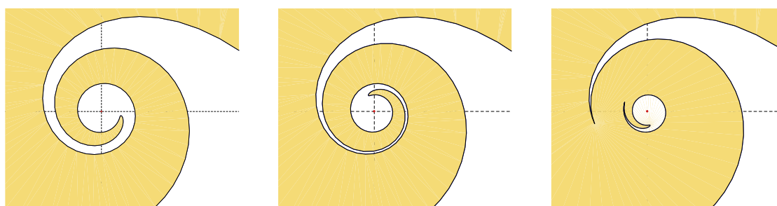
FIGURE 4.12 – Trois boules avec un zoom autour du vortex (point rouge) aux temps t \in \{2.86, 2.88, 2.9\} . Comparez avec la Figure 4.11. Pour t = 2,9 la boule \bar{\mathbb{B}}(x_0, t) est de type B et possède un petit trou en forme de fœtus.
