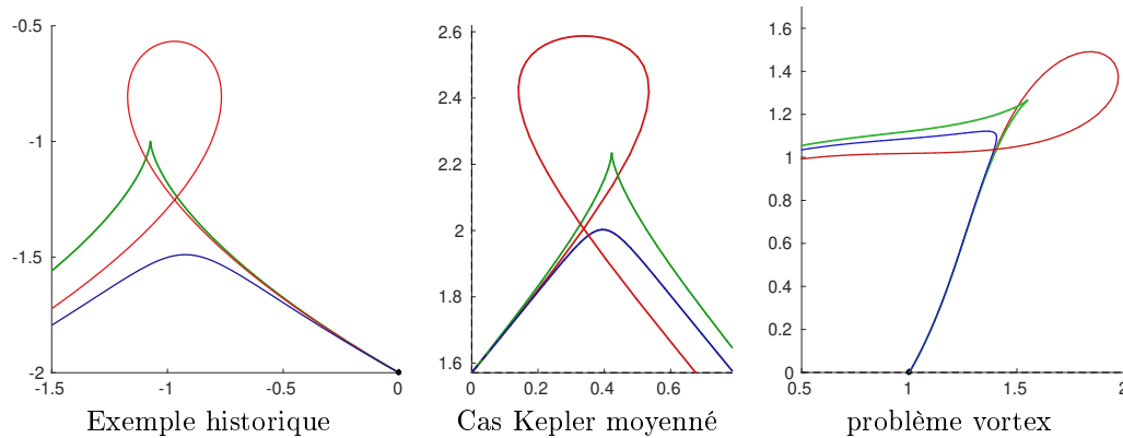
FIGURE 2.8 – Déploiement de la singularité du cusp dans les différents cas d'étude.
