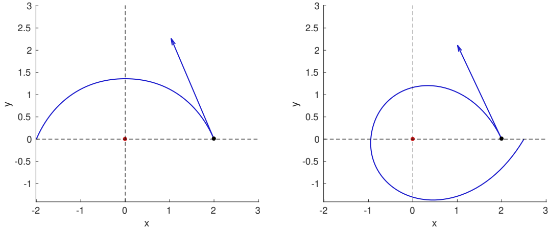
FIGURE 5.5 – Géodésique solution dans le cas d'un courant fort en q_0 : \mu = 2 \|q_0\| . (Gauche) q_0 = (2, 0) , q_f = (-2, 0) et le temps final vaut t_f \approx 1.641 . (Droite) q_0 = (2, 0) , q_f = (2.5, 0) et le temps final vaut t_f \approx 2.821 .
