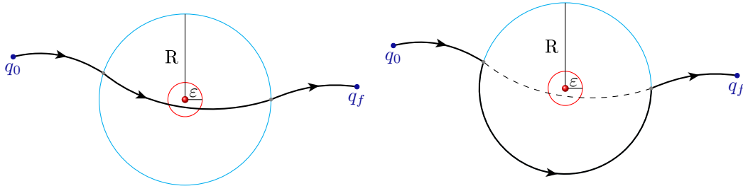
FIGURE 4.1 – Illustration de la construction d'une trajectoire admissible strictement meilleure. Le vortex est représenté par une boule rouge, tandis que les trajectoires sont les lignes noires pleines. On peut voir à gauche, une trajectoire traversant la boule de rayon \varepsilon . Cette trajectoire est remplacée sur le graphe de droite par une trajectoire admissible strictement meilleure.
