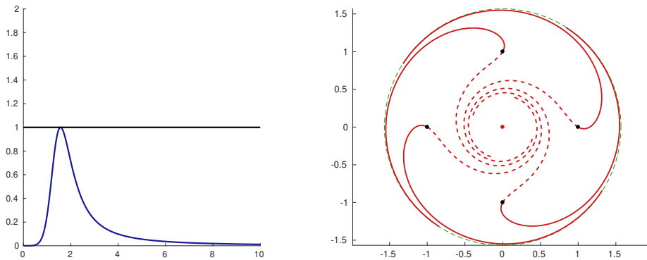
FIGURE 4.8 – Feuilletage de Reeb formé par la séparatrice paramétrée par p_\theta^1 . En trait continu les trajectoires sont parcourues en temps positif et en pointillés elles sont parcourues en temps négatif. Le vortex est représenté par le point rouge et les différents points initiaux par les points noirs. Le cercle en vert représente l'équateur associé à r_1 .
