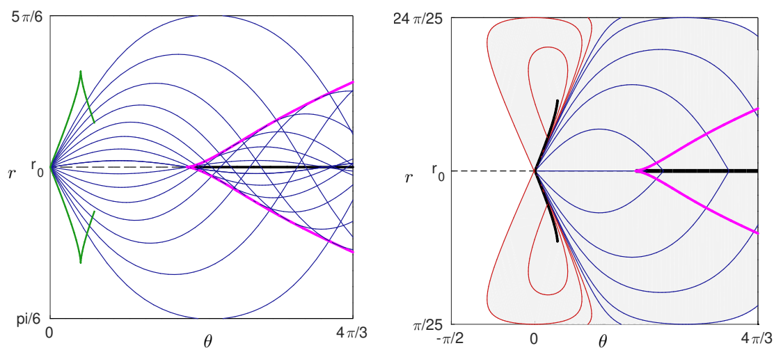
FIGURE 3.8 – (Gauche) Flot hyperbolique et lieux conjugués et de coupure. (Droite) Synthèse optimale en temps minimal dans un voisinage adapté R = \{\pi/25 \leq r \leq 24\pi/25; -\pi/2 \leq \theta \leq 4\pi/3\} . Les pseudo-méridiens (séparatrices) sont représentés en noir tandis que les géodésiques hyperboliques à gauche (resp. à droite) des séparatrices sont représentées en rouge (resp. en bleu). Les géodésiques anormales sont représentées en vert. le lieu conjugué et le lieu de coupure sont représentés resp. en magenta et en noir. le secteur hachuré en gris représente, dans le voisinage adapté considéré, le domaine atteignable. le domaine en blanc n'est pas atteignable dans le voisinage adapté. On prend \lambda = 4/5 et v = 0.9 .
