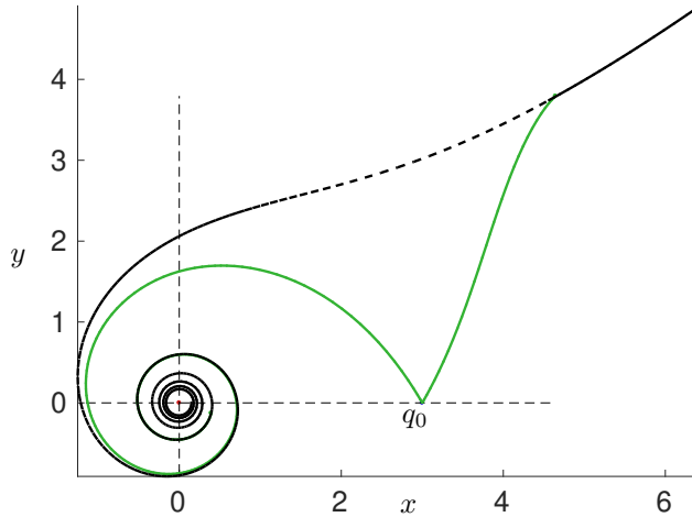
FIGURE 5.8 – Représentation du lieu de séparation isochrone (courbe noir) pour le problème à un vortex calculé par homotopie grâce au code HamPath. Il peut être décomposé en trois morceaux dont les deux morceaux représentés en trait continu sont formés de géodésiques hyperboliques et le morceau représenté par des tirets est formé de géodésiques elliptiques. En vert sont représentées les géodésiques anormales. Pour le représentation on a considéré r_0 = 3.0 et k = 2r_0 .
