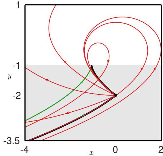
FIGURE 3.3 – Synthèse optimale en temps minimal dans un voisinage adapté contenant la boucle limite (géodésique qui repasse par q_0 ). Le point initial est q_0 = (0, -2) . Les géodésiques anormales sont représentées en vert et en rouge sont représentées les géodésiques hyperboliques. Le lieu de coupure coïncide avec l’anormale qui a un point cusp, jusqu’à ce point cusp, et est représenté en noir.
