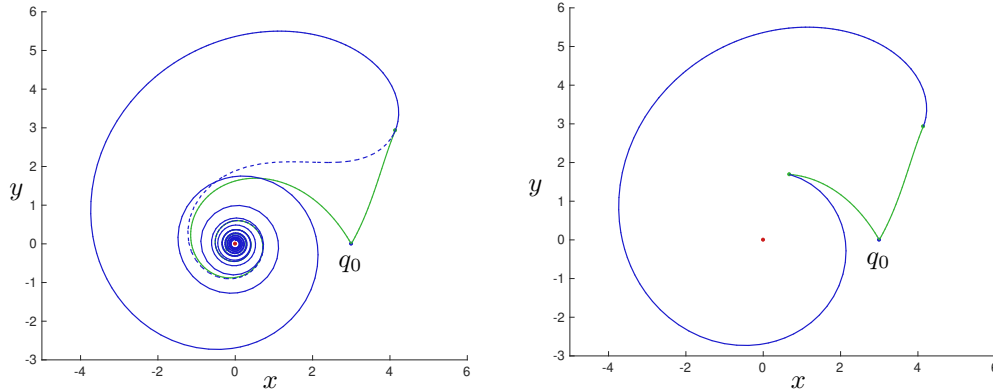
FIGURE 5.7 – front d’ondes (hyperbolique et elliptique) + anormales, sphère et boule dans le plan (x, y) au temps t_f = 2.9 dans le cas du problème vortex pour un courant fort, où on a considéré r_0 = 3.0 et k = 2r_0 .
