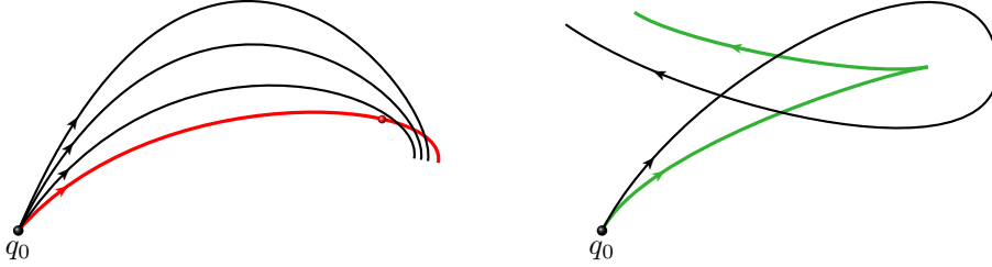
FIGURE 2.1 – Illustration de points conjugués dans le cas normal (à gauche) et anormal (à droite).
