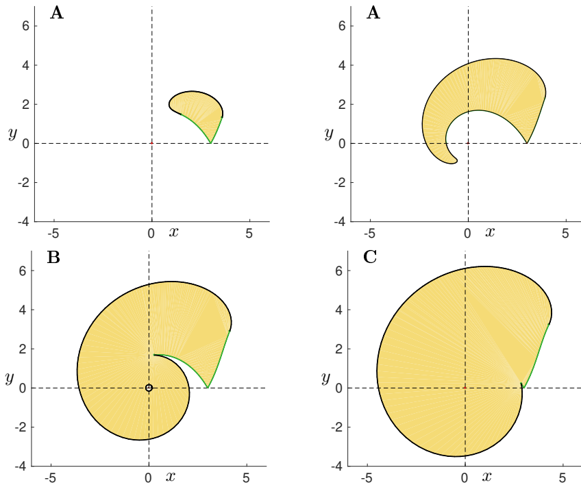
FIGURE 4.14 – Quatre boules dans le plan (x, y) aux instants t \in \{1.0, 2.0, 2.85, 6.0\} avec la condition initiale q_0 représentée par un point noir et le vortex par un point rouge. Les boules \mathbb{B}(q_0, 1.0) et \mathbb{B}(q_0, 2.0) en haut sont de type A. La boule \mathbb{B}(q_0, 2.85) (en bas à gauche) est de type B tandis que \mathbb{B}(q_0, 6.0) (en bas à droite) est de type C. En vert on a les géodésiques anormales.
