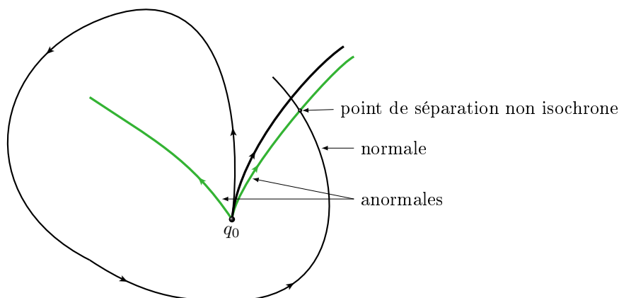
FIGURE 2.3 – Illustration d'un point de séparation non isochrone. La géodésique hyperbolique venant de l'extérieur intersecte la géodésique anormale avec un temps strictement plus grand.
