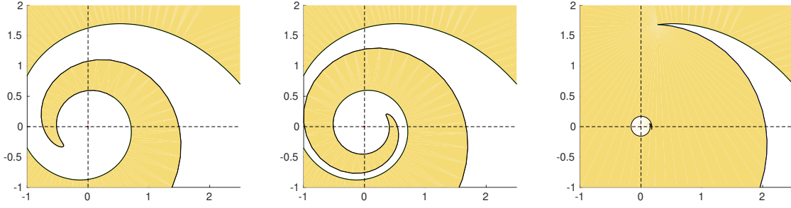
FIGURE 4.15 – Trois boules avec un zoom autour du vortex (point rouge) aux temps t \in \{2.5, 2.6, 2.85\} . Comparez avec la Figure 4.14, Pour t = 2,85 la boule \mathbb{B}(q_0, t) est de type B et possède un petit trou en forme de fœtus.
