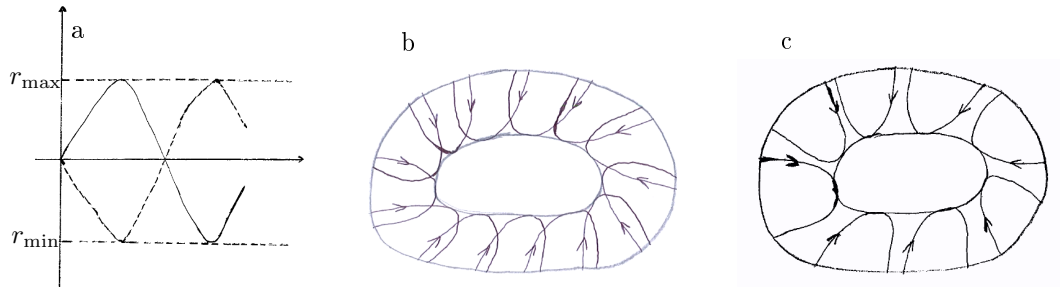
FIGURE 1.2 – Types de trajectoires dans le cas oblat de l’ellipsoïde de révolution. sur le sous-graphe (a) on donne une illustration des courbes méridiennes avec \dot{r} > 0 . Sur le sous-graphe (b) sont représentés les géodésiques denses sur le tore délimitées par l’équateur. Sur le sous-graphe (c) sont représentés les géodésiques périodiques différentes de l’équateur et des méridiens.
