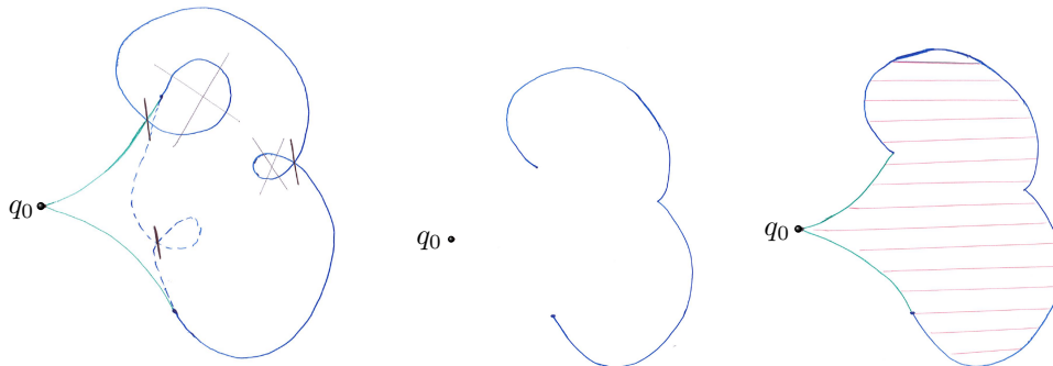
FIGURE 2.13 – Illustration du front d'ondes, de la sphère et de la boule dans le cas fort avec un point d'intersection entre le front d'ondes et une anormale. (Gauche) Front d'onde hyperbolique (bleu) et elliptique (bleu interrompu) + géodésiques anormales. (Milieu) Sphère temps minimal. (Droite) Boule délimitée par la sphère et les anormales.
