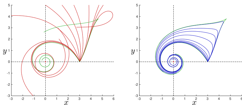
FIGURE 5.3 – Illustration du flot géodésique dans le cas du problème vortex dans le plan (x, y) avec q_0 = (3, 0)
