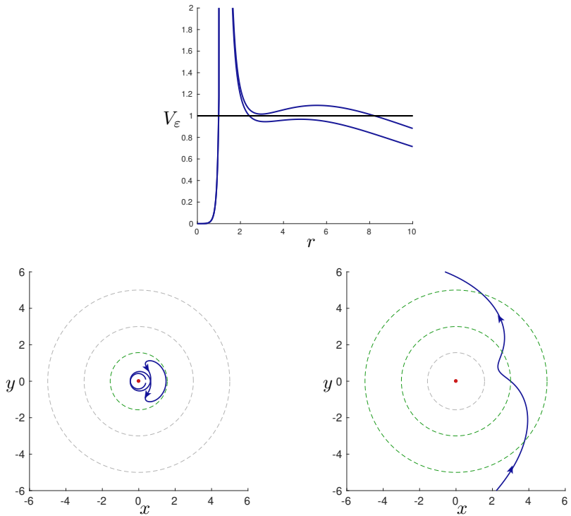
FIGURE 4.6 – Cas 2-(a). On déduit du potentiel (en haut) que les trajectoires qui proviennent du vortex retournent vers celui-ci et que celles qui démarrent d’un r_0 assez grand vont à l’infini.
