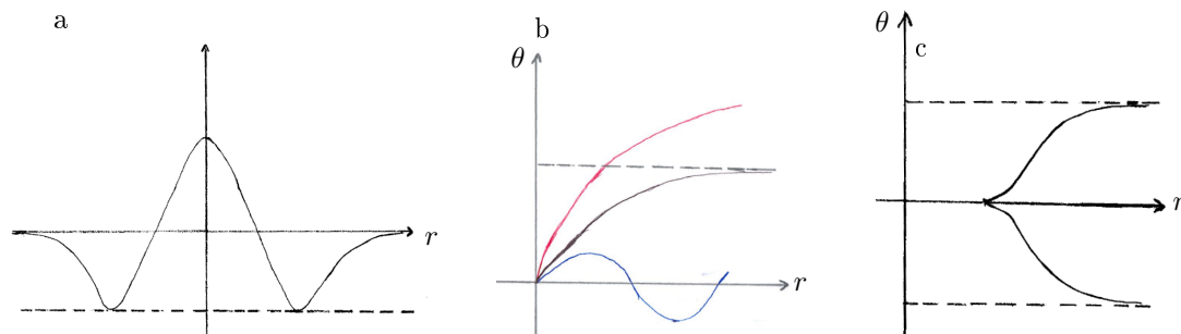
FIGURE 1.3 – Cas Serret-Andoyer : Sur le sous-graphe (a) est représenté le potentiel en fonction de r . Sur le sous-graphe (b) sont représentées les différents types de trajectoires, en noir on a la séparatrice, en bleu les trajectoires qui oscillent et en rouge celles qui font des rotations complètes. Sur le sous-graphe (c) est représenté le lieu conjugué lorsqu’on démarre de l’équateur.
