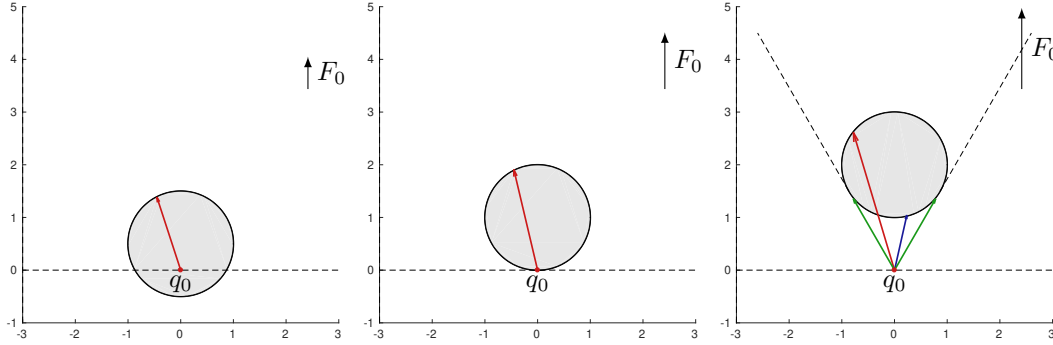
FIGURE 1 – Illustration de l'ensemble \mathcal{F}(q) = \left\{ F_0(q) + \sum_{i=1}^2 u_i F_i(q) \mid \|u\| \leq 1 \right\} des directions initiales possibles (disque gris avec son bord en noir) dans les cas Zermelo faible (gauche), Zermelo modéré (milieu) et Zermelo fort (droite), avec F_0 supposé vertical en q_0 . Les directions initiales possibles, dans le cas Zermelo fort, sont contenues dans un cône.
