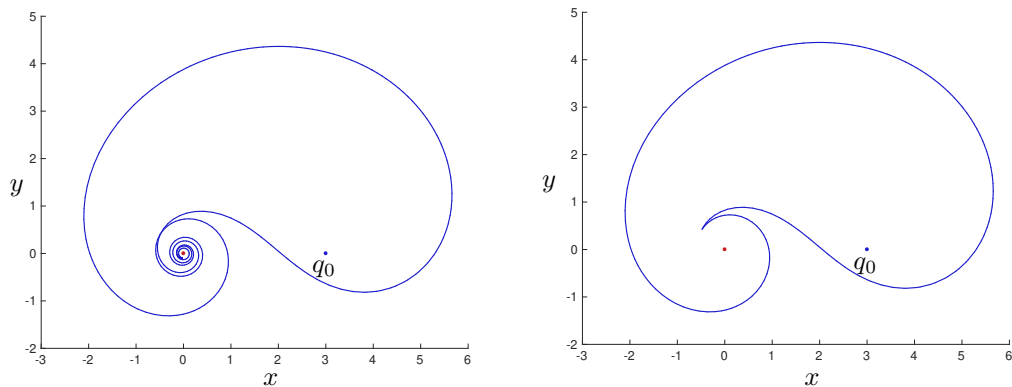
FIGURE 5.6 – front d'ondes, sphère et boule dans le plan (x, y) au temps t_f = 2.9 dans le cas du problème vortex pour un courant faible, où on a considéré r_0 = 3.0 et k = 0.6r_0 .
