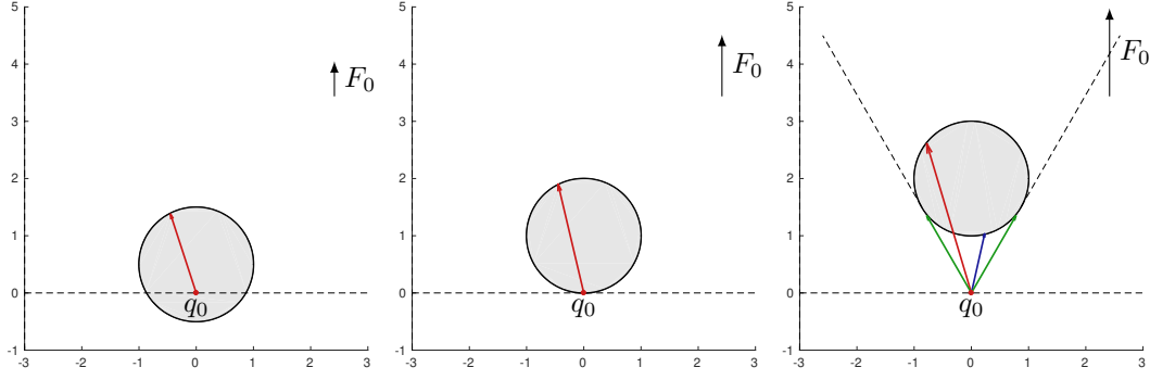
FIGURE 1.1 – Illustration des directions initiales possibles dans les trois cas pour un courant supposé vertical. (Gauche), cas Zermelo faible; (Milieu) cas Zermelo modéré; (Droite) cas Zermelo fort. En vert sont représentés les directions anormales, en rouge les hyperboliques et en bleu les elliptiques. Le points rouge correspondent au point initial.
