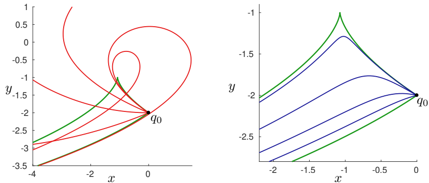
FIGURE 5.1 – Illustration du flot géodésique dans l'exemple historique dans le plan (x, y) avec q_0 = (0, -2) .
