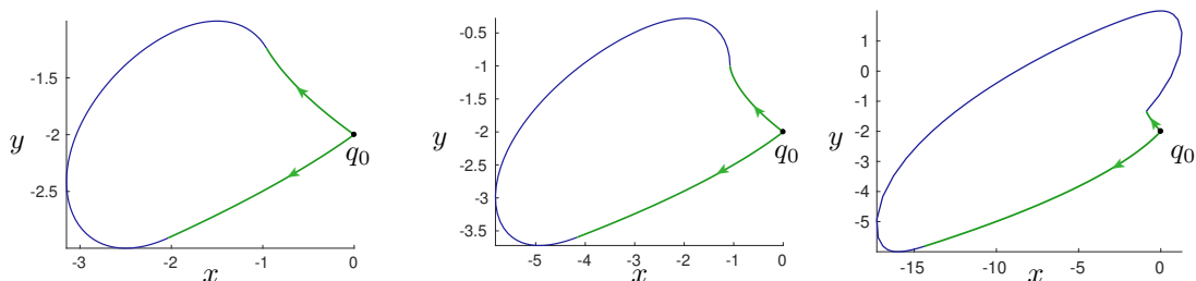
FIGURE 3.5 – Sphères et boules aux temps respectifs t_f = 1.0 , t_f = t_{\text{cusp}} , t_f = 4.0 .
