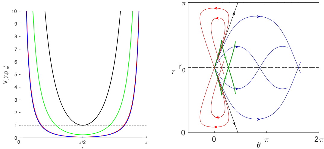
FIGURE 3.6 – (Gauche) Potentiel généralisé pour les différents types de géodésiques afin de mettre en évidence la périodicité des solutions. (Droite) Illustration des différents types de géodésiques hyperboliques dans le cas fort. Les méridiens et l'équateur sont représentés en noir tandis que les géodésiques hyperboliques à gauche (resp. à droite) de la séparatrice sont représentées en rouge (resp. en bleu). Les géodésiques anormales sont représentées en vert. Dans cette représentation, on prend \lambda = 4/5 et v = 0.9 . Toutes les trajectoires sont intégrées jusqu'au temps t_f = \pi .
