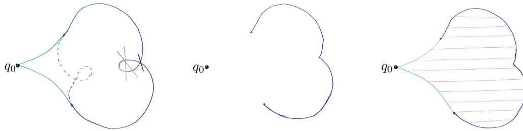
FIGURE 2.12 – Illustration du front d'ondes, de la sphère et de la boule dans le cas fort sans point d'intersection entre le front d'ondes et les anormales. (Gauche) Front d'onde hyperbolique (bleu) et elliptique (bleu interrompu) + géodésiques anormales. (Milieu) Sphère temps minimal. (Droite) Boule délimitée par la sphère et les anormales.
