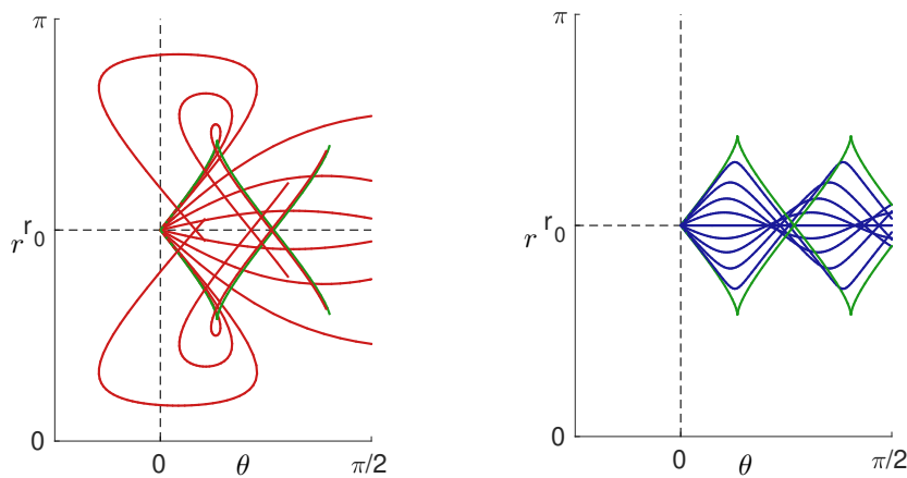
FIGURE 5.2 – Illustration du flot géodésique dans le cas du Kepler moyenné dans le plan (\theta, r) avec q_0 = (0, \pi/2) .
