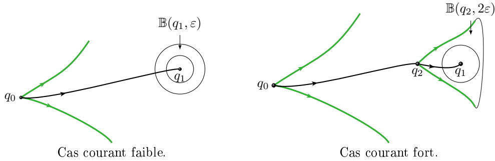
FIGURE 2.5 – Illustration de la construction d'un voisinage de q_1 contenu dans la boule zermelienne dans les cas faible et fort. En vert sont représentés les anormales et en noir la normale de référence considéré.
