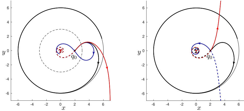
FIGURE 4.3 – (Gauche) Comportement des trajectoires autour de la séparatrice (noir). Les géodésiques en dessous de la séparatrice (bleu), c'est-à-dire paramétrées par p_\theta < p_\theta^* ( p_\theta^* paramétrant la séparatrice), convergent vers le vortex et celles au-dessus de la séparatrice (rouge) vont à l'infini. Cependant, au voisinage de la séparatrice les géodésiques proviennent toutes du vortex. (Droite) Illustration des deux pseudo-méridiens représentés en rouge et bleu. Les orbites de celles-ci ne coïncident pas à cause de la dérive. En pointillé les trajectoires sont parcourues en temps négatif.
