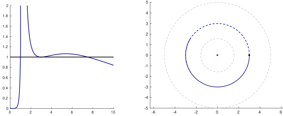
FIGURE 4.9 – Équateur L-elliptique associé à r_2 . En trait continu les trajectoires sont parcourues en temps positif et en pointillés elles sont parcourues en temps négatif. Le vortex est représenté par le point rouge et les différents points initiaux par les points noirs. Les cercles en gris représentent les équateurs associés à r_1 et r_3 .
