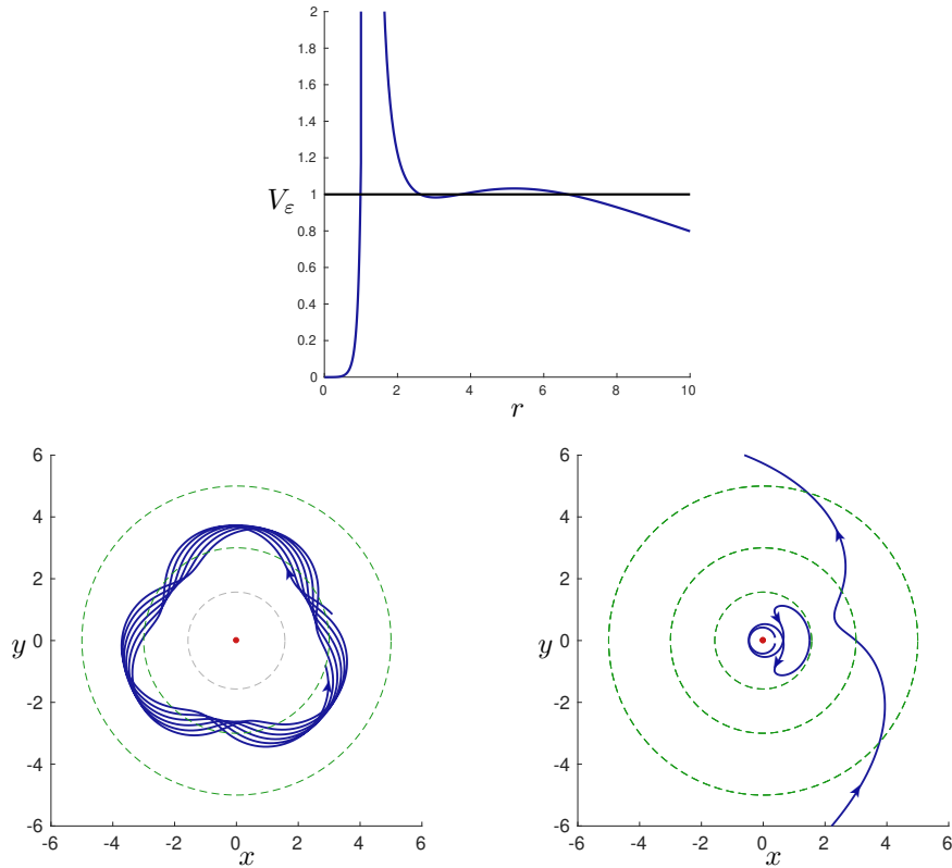
FIGURE 4.7 – Cas 2-(b). On déduit des potentiels (en haut) que les trajectoires qui démarrent entre le minimum et le maximum demeurent contenues dans une couronne, que celles qui proviennent du vortex retournent vers celui-ci et que celles qui démarrent d'un r_0 assez grand vont à l'infini. Dans le graphe en bas à gauche on représente une trajectoire compacte et dans celui de droite on affiche les deux autres situations. Sur le graphe de droite est représentée une trajectoire pour laquelle le potentiel associé a son maximum local inférieur strictement à 1 : on peut la voir osciller autour de l'équateur r_2 L-elliptique.
