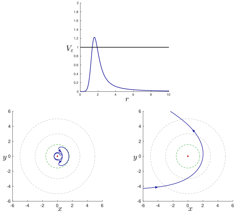
FIGURE 4.5 – Cas 1-(b). On déduit du potentiel (en haut) que les trajectoires qui proviennent du vortex retournent vers celui et que celles qui démarre à un r_0 assez grand vont à l’infini.
