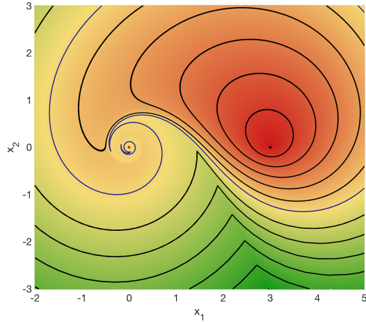
FIGURE 4.13 – Synthèse optimale dans le cas d'un courant faible. Les courbes noires représentent les sphères de types A et C. Les deux courbes bleues sont une sphère unique de type B. Puisque les boules de type B ne sont pas simplement connexes et ont un trou, les sphères correspondantes ont deux composantes connexes.
