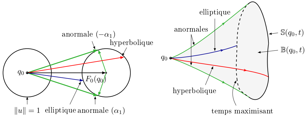
FIGURE 2.10 – (Gauche) boule de directions. (Droite) Sphère et boule en temps petit dans le cas Zermelo fort avec F_0 considéré horizontal et orienté dans le sens positif.
