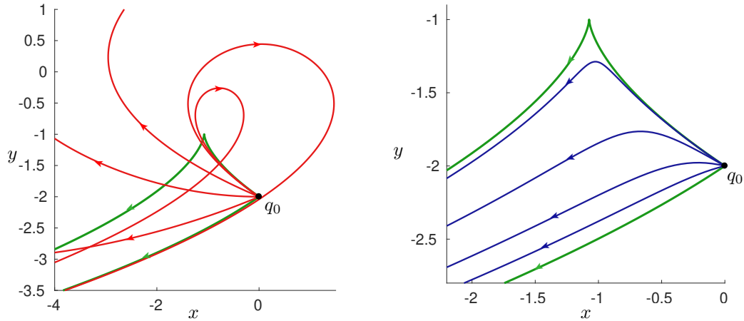
FIGURE 3.1 – Flot géodésique dans les cas hyperbolique (gauche) et elliptique (droite) dans le voisinage conique délimité par les deux géodésiques anormales (vert). Les géodésiques hyperboliques sont représentées en rouge et les elliptiques en bleu. Le point initial est pris à q_0 = (0, -2) .
