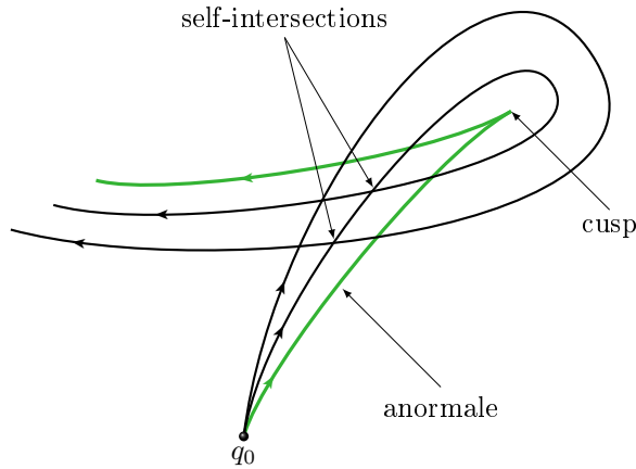
FIGURE 2.2 – Illustration d'une géodésique anormale avec un point cusp apparaissant comme limite de géodésiques hyperboliques qui se recoupent.
