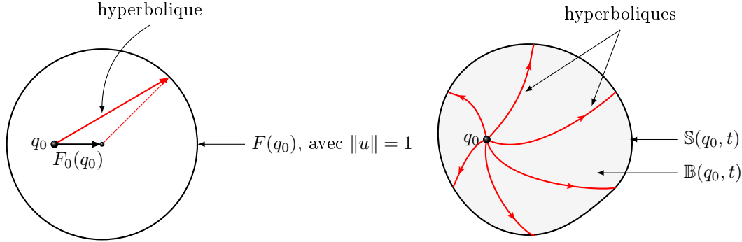
FIGURE 2.9 – (Gauche) Boule de directions dans le cas Zermelo faible. (Droite) Sphère et boule dans le cas Zermelo faible avec F_0 considéré horizontal et orienté dans le sens positif.
