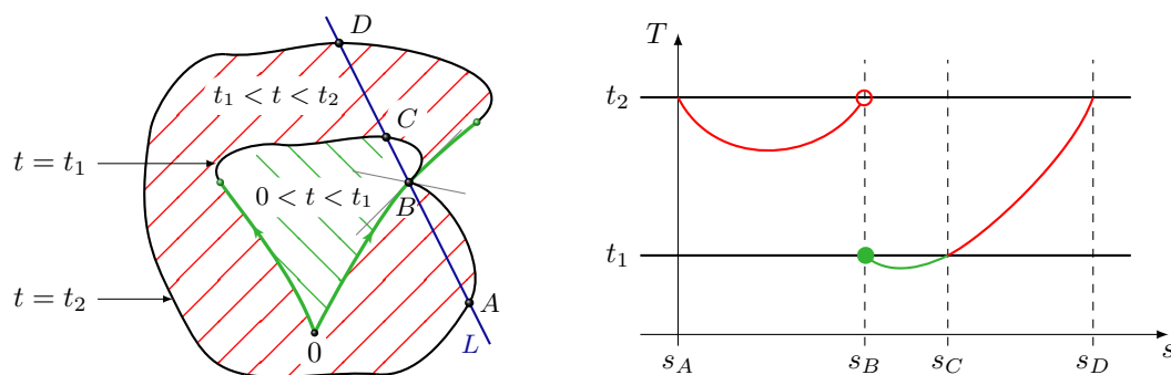
FIGURE 2.4 – Discontinuité de la fonction temps minimal V_{q_0}(\cdot) en un point de séparation non isochrone. Considérons deux temps 0 < t_1 < t_2 , avec t_1 petit et t_2 assez grand. (Gauche) Boules de rayons t_1 et t_2 avec les sphères correspondantes. La fonction temps minimal V_{q_0}(\cdot) est discontinue en B , à l'intersection de l'anormale de droite de longueur t_1 et d'une géodésique hyperbolique de longueur t_2 . (À droite) La fonction temps minimal V_{q_0}(\cdot) le long de la droite L paramétrée par s et telle que les coordonnées s_A, s_B, s_C et s_D correspondent respectivement aux points A, B, C et D . On peut voir la discontinuité de V_{q_0}(\cdot) en s_B .
