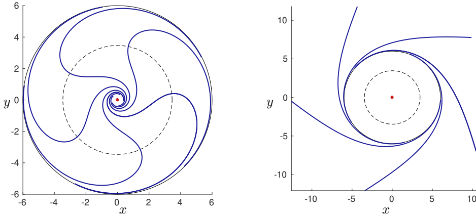
FIGURE 4.2 – (Gauche) Séparatrices formant une composante de Reeb par rotation sur l'angle \theta_0 avec singularité à l'intérieur du disque délimité par l'équateur ( r^* = 2k ). (Droite) Séparatrices émanant de l'équateur et convergeant vers l'infini pour des rayon plus grand que r^* . Sur les deux graphes, les cercles en noir et en pointillé correspondent respectivement au cercle équateur et au cercle de rayon k délimitant le domaine de courant fort. Le vortex est représenté par le point rouge.
