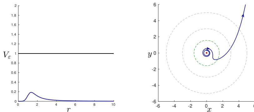
FIGURE 4.4 – Cas 1-(a). On peut déduire du potentiel représenté sur le graphe de gauche que les trajectoires proviennent nécessairement du vortex et vont à l'infini, l'orientation des trajectoires étant prise suivant le sens positif d'intégration que l'on a choisi.
