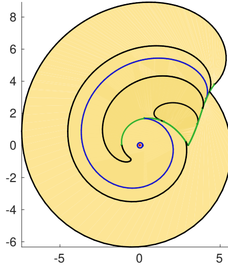
FIGURE 4.16 – Synthèse optimale dans le cas d'un courant fort. Les courbes noires représentent les sphères de types A et C. Les deux courbes bleues sont une sphère unique de type B. Puisque les boules de type B (en bleu) ne sont pas simplement connexes et ont un trou, les sphères correspondantes ont deux composantes connexes.
