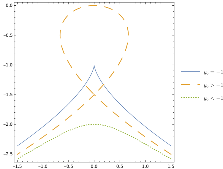
FIGURE 2.7 – Exemple historique de Carathéodory-Zermelo, "Plus rapide chemin nautique", comme un déploiement de la singularité générique du cusp le long de géodésiques anormales.
