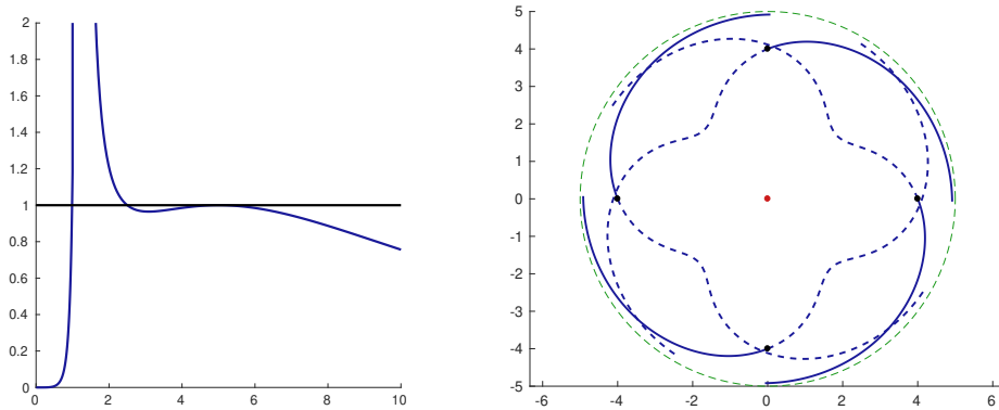
FIGURE 4.10 – Séparatrice homocline paramétrée par p_\theta^3 . En trait continu les trajectoires sont parcourues en temps positif et en pointillés elles sont parcourues en temps négatif. Le vortex est représenté par le point rouge et les différents points initiaux par les points noirs. Le cercle en vert représente l'équateur associé à r_3 .
