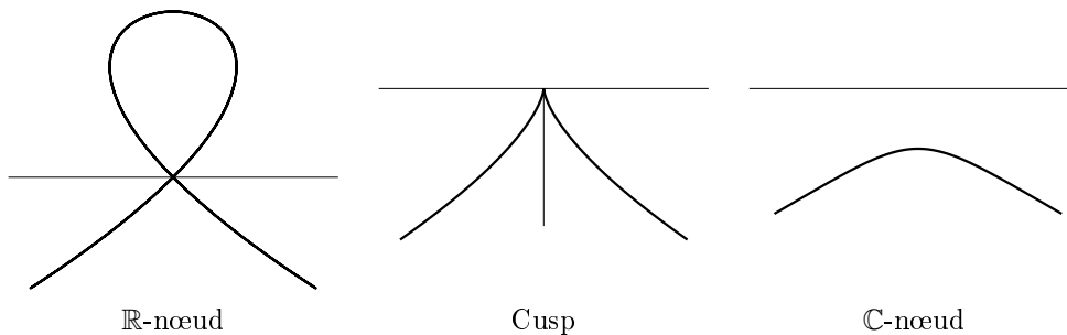
FIGURE 2.6 – Point cusp vu comme une transition entre un \mathbb{R} -nœud et un \mathbb{C} -nœud.
