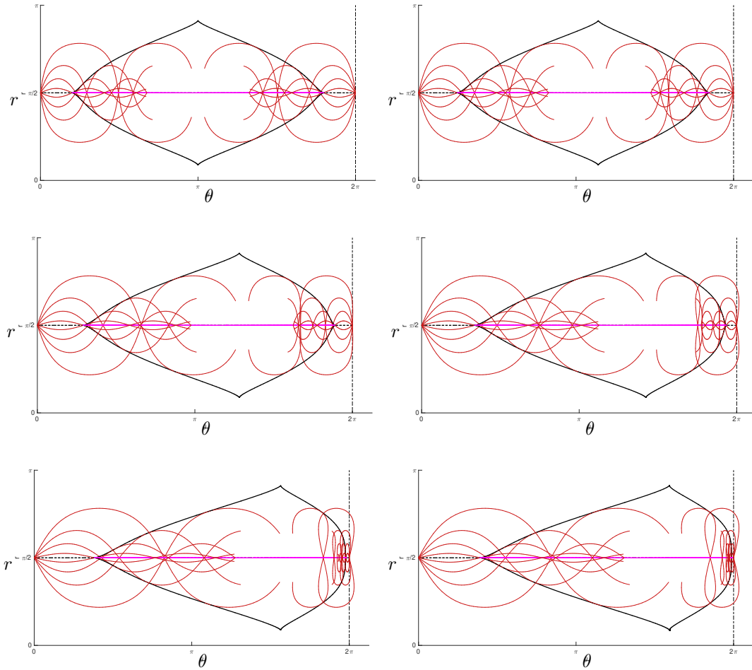
FIGURE 3.7 – Illustration de la déformation du flot géodésique et du lieu conjugué dans le cas faible. En prenant \lambda = 4/5 et v = 0.0, 0.1, 0.2, 0.3, 0.4, 0.42 respectivement de haut à gauche en bas à droite. Les géodésiques hyperboliques sont représentées en rouge, le lieu conjugué et le lieu de coupure sont respectivement représentés en noir et en magenta.
