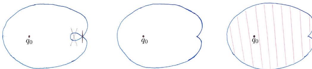
FIGURE 2.11 – Illustration du front d'ondes, de la sphère et de la boule dans le cas faible, représenté respectivement de la gauche vers la droite.
