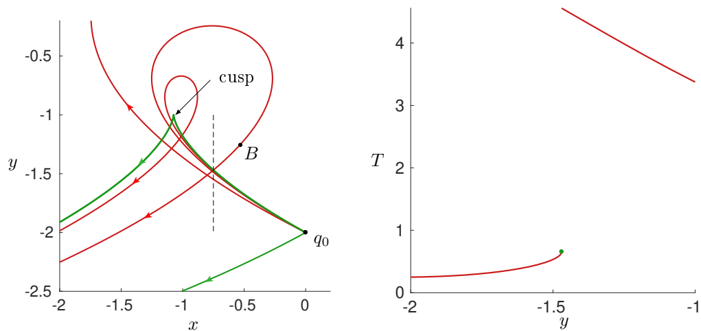
FIGURE 3.2 – Illustration de la discontinuité de la fonction temps minimale en un point de séparation non isochrone. (Gauche) Le point initial est q_0 = (0, -2) . Les géodésiques anormales sont représentées en vert tandis que les autres géodésiques en rouge sont hyperboliques. On voit que le point cusp est limite de "self-intersections" de géodésiques hyperboliques. De plus, pour atteindre le point B à partir de q_0 , on doit utiliser une géodésique hyperbolique qui a une boucle. Lorsque cette géodésique hyperbolique intersecte l'anormale, le temps est plus grand le long de l'hyperbolique que de l'anormale. À cette intersection, la géodésique hyperbolique cesse d'être optimale. (Droite) Fonction temps minimale le long du segment pointillé du sous-graphe de gauche. La discontinuité se produit à l'intersection entre les géodésiques hyperbolique et anormale. Elle est représentée par le point vert, qui est le temps le long de la géodésique anormale.
