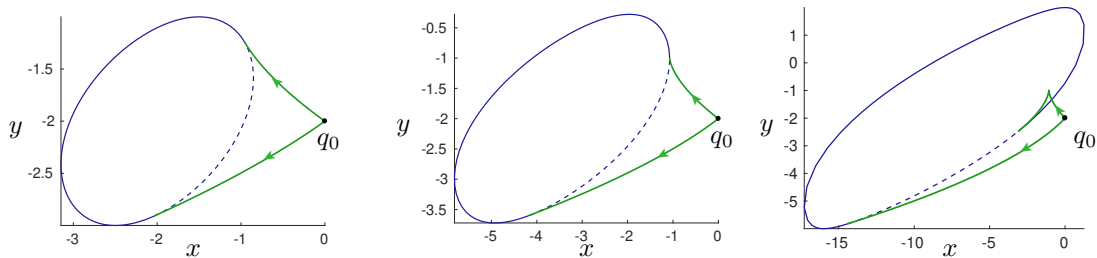
FIGURE 3.4 – Fronts d’ondes (hyperbolique en traits plein et elliptique en tirets) et anormales aux temps respectifs t_f = 1.0 , t_f = t_{\text{cusp}} , t_f = 4.0 .
