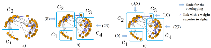
FIGURE 3.12 – Réseau de Zachary avec la fonction f_b , a) \alpha \geq 0.6 , b) \alpha \geq 0.7 c) \alpha \geq 0.8 .
