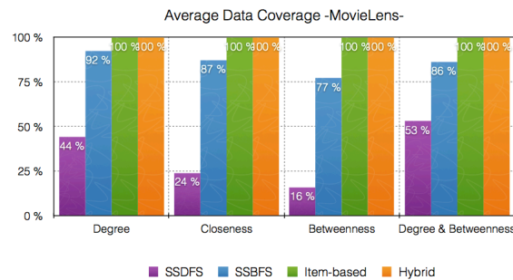
FIGURE 2.15 – Taux de couverture des données MovieLens.
