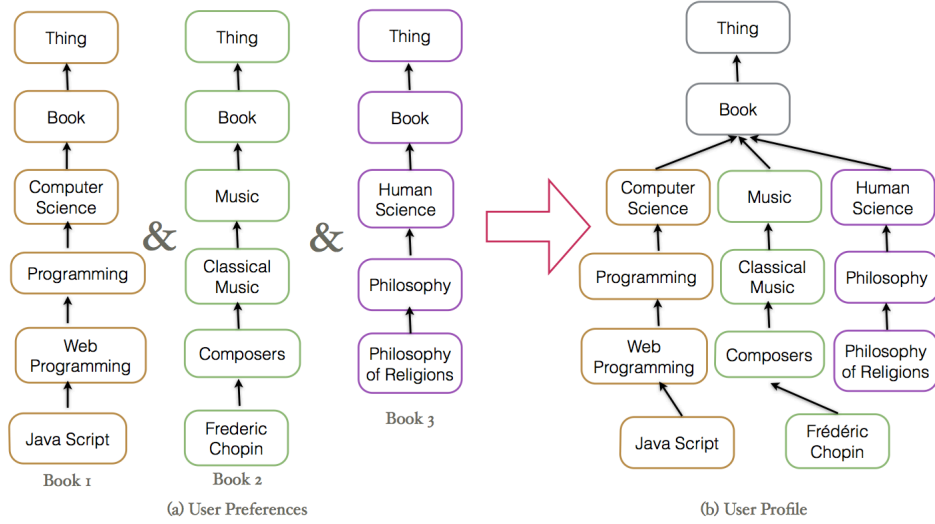
FIGURE 2.8 – Exemple d'un profil utilisateur (Sulieman et al. [129]).
