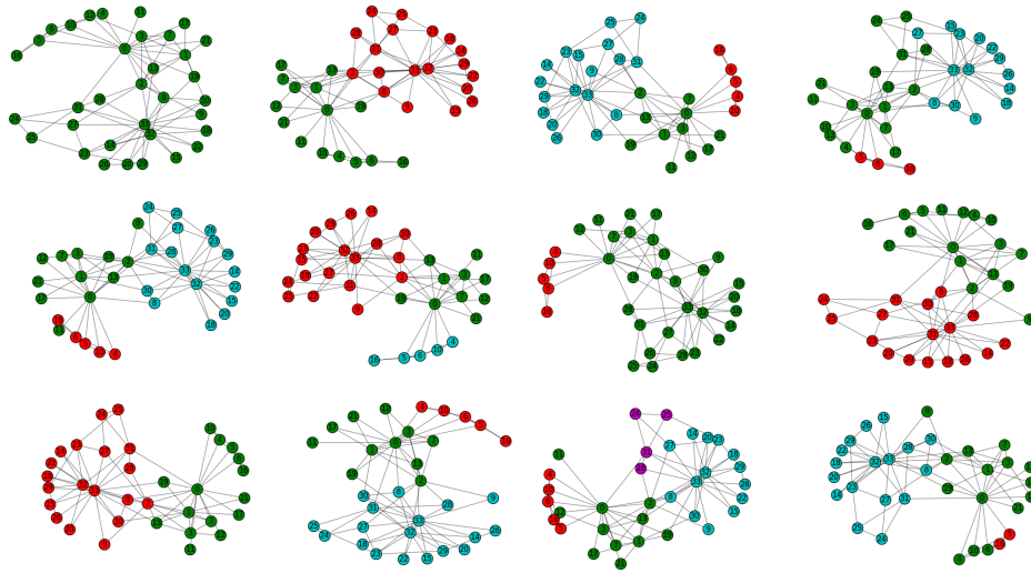
FIGURE 3.4 – La propagation de labels est un algorithme non déterministe et instable (Attal [7]). Application sur le graphe de Karaté (Zachary [146]).
