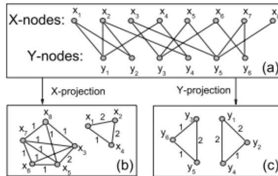
FIGURE 1.1 – Illustration de la projection d’un réseau d’affiliation (source : Zhou et al. [152]).
