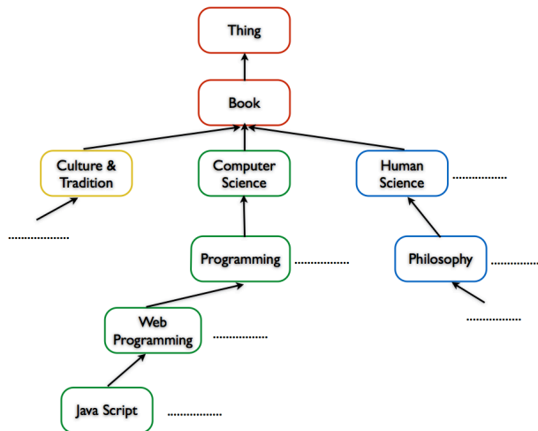
FIGURE 2.6 – Petit extrait de la taxonomie livre .
