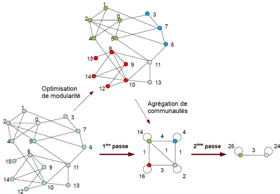
FIGURE 3.2 – Exemple d’application de la méthode de Louvain sur un graphe à 16 sommets (Extrait de Blondel et al. [24]).
