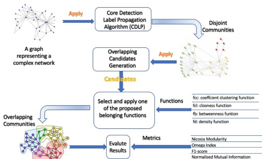
FIGURE 3.6 – Diagramme représentant notre approche de détection de communautés chevauchantes en utilisant des fonctions d'appartenance (Attal et al. [10]).
