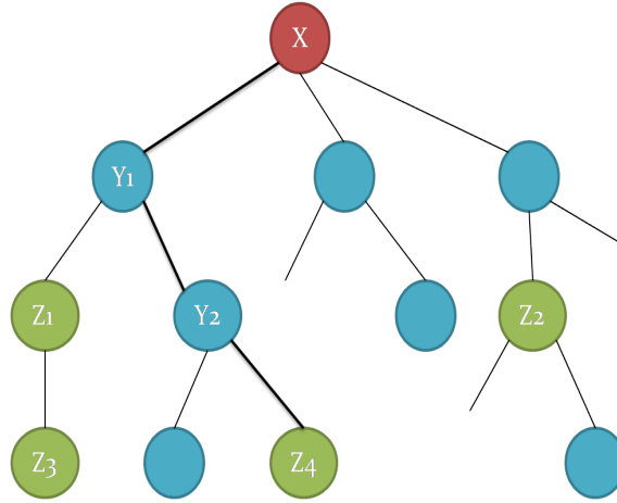
FIGURE 2.2 – Exemple du déroulement de l'algorithme de recommandation dans un arbre couvrant : X étant l'auteur qui soumet la requête ; une recherche des sommets pertinents est effectuée, soient [Z_4, Z_3, Z_1, Z_2] cette liste : un poids qui dépend de la mesure d'intermédiarité des acteurs sur le chemin (X, Z_i) est affecté à chaque sommet retenu ; la liste de sommets à recommander est [(Z_4, P_4), (Z_3, P_3), (Z_1, P_1), (Z_2, P_2)] (Kadima et Malek [65]).
