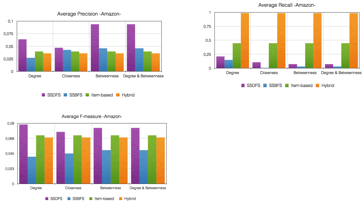
FIGURE 2.14 – Résultats des algorithmes SSDFS , SSBFS , Filtrage collaboratif centré sur les items et algorithmes hybrides sur les données de Amazon.com : précision, rappel et F -score vs. mesures de centralité (Suliman et al. [129]).
