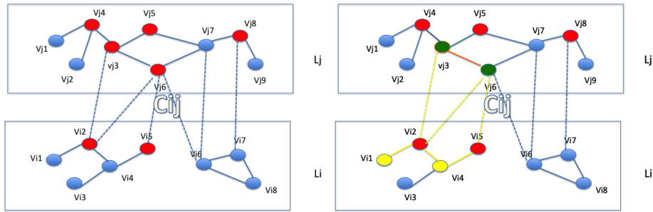
FIGURE 4.6 – Accessibilité de la couche i à la couche j : les nœuds rouges sont privés, les nœuds jaunes et verts sont des nœuds accessibles calculés à partir de la couche i , les nœuds verts sont les nœuds accessibles qui appartiennent au réseau privé de la couche j , \text{precisionR}(i, j) = 1 et \text{rappelR}(i, j) = 0.4 : cela signifie que tous les nœuds accessibles depuis la couche i sont des nœuds privés mais seulement 40 % des nœuds privés de la couche j sont accessibles depuis la couche i (Malek et al. [91]).
