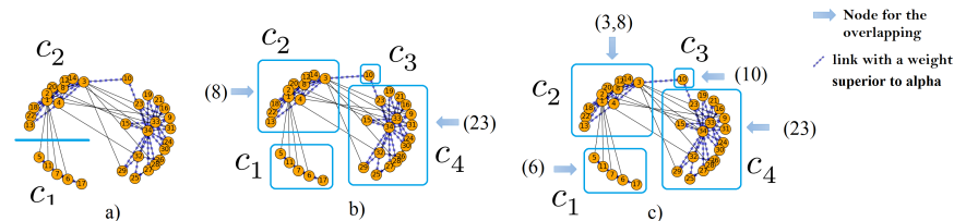
FIGURE 3.13 – Réseau de Zachary avec la fonction f_{cd} , a) \alpha \geq 0.6 , b) \alpha \geq 0.7 c) \alpha \geq 0.8 .
