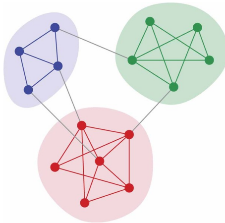
FIGURE 3.1 – Exemple d'une structure de communautés dans un graphe simple.
