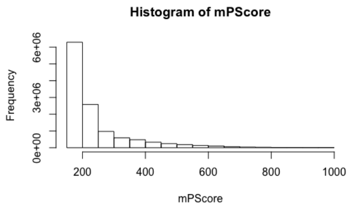
FIGURE 4.13 – La distribution du score combiné extrait de la base de données ouverte STITCH.
