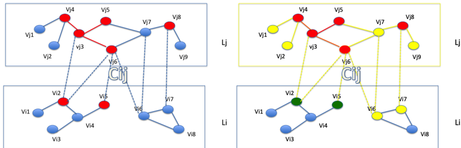
FIGURE 4.7 – Accessibilité de la couche j à la couche i : les nœuds rouges sont privés, les nœuds jaunes et verts sont des nœuds accessibles calculés à partir de la couche j , les nœuds verts sont les nœuds accessibles qui appartiennent au réseau privé de la couche i , \text{precisionR}(j, i) = 0.5 et \text{rappelR}(j, i) = 1 : cela signifie que 50% des nœuds accessibles depuis la couche j sont des nœuds privés mais tous les nœuds privés de la couche i sont accessibles depuis la couche j (Malek et al. [91]).
