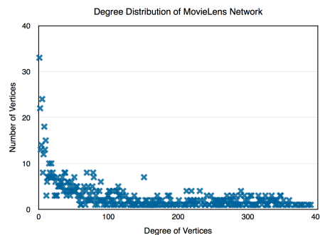
FIGURE 2.11 – Distribution des degrés du réseau de collaboration MovieLens (Sulieman et al. [129]).
