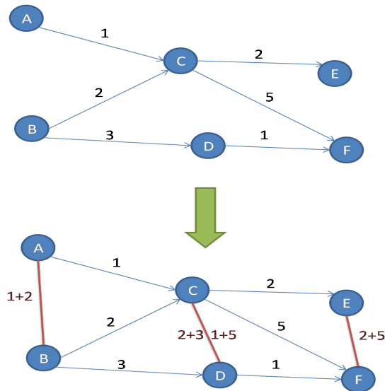
FIGURE 2.3 – Le graphe de citations (liens orientés bleus) et le graphe de similarité (lien non orientés rouges).
