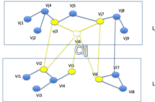
FIGURE 4.3 – Exemple d'un réseau égocentrique à 2 couches (Malek et al. [91]).
