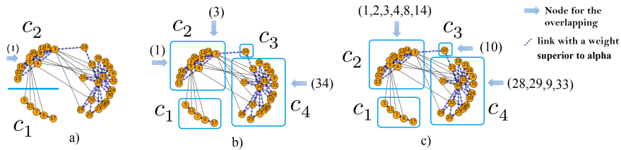
FIGURE 3.11 – Réseau de Zachary avec la fonction f_{cc} , a) \alpha \geq 0.6 , b) \alpha \geq 0.7 c) \alpha \geq 0.8 .
