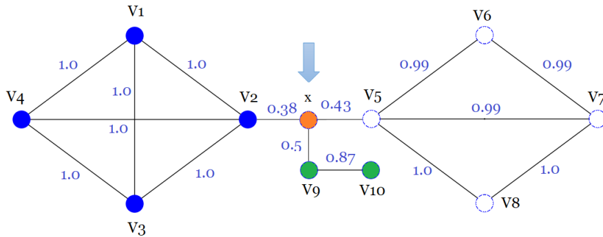
FIGURE 3.8 – Un graphe avec 3 communautés évidentes et un nœud ( x ) dont l’appartenance à une communauté spécifique est discutable.
