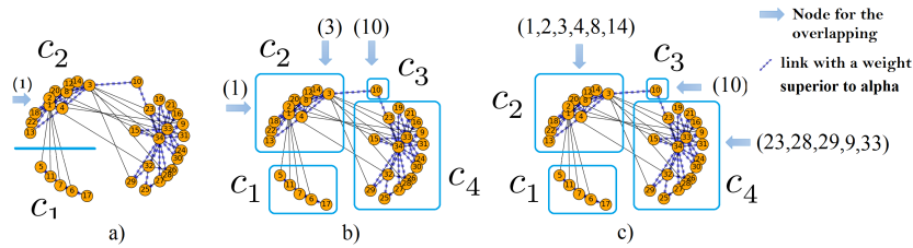
FIGURE 3.10 – Réseau de Zachary avec la fonction f_d , a) \alpha \geq 0.6 , b) \alpha \geq 0.7 c) \alpha \geq 0.8 .
