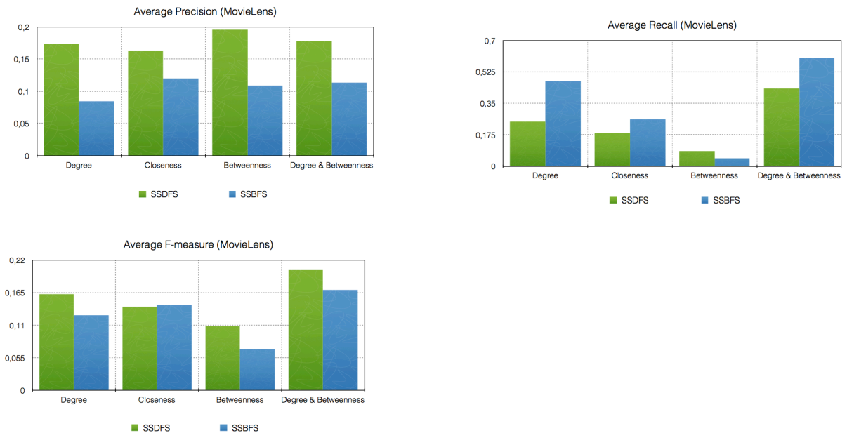
FIGURE 2.13 – Résultats des algorithmes SSDFS, SSBFS sur les données de MovieLens : précision, rappel et F -score vs. mesures de centralité (Suliman et al. [129]).
