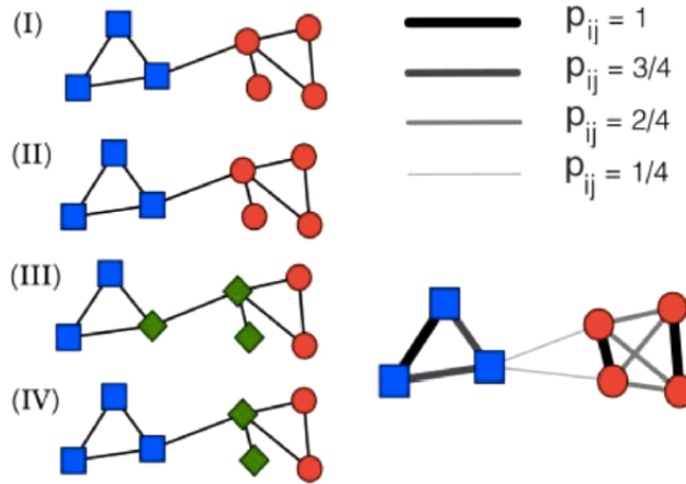
FIGURE 3.7 – Exemple des résultats obtenus en appliquant l’algorithme CDLP : communautés obtenues avec N = 4 et \alpha = 0.5 .
