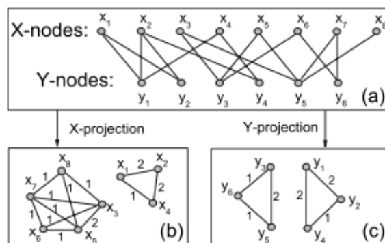
FIGURE 4.15 – Illustration de la projection d'un réseau bipartite (source : Zhou et al. [152]).
