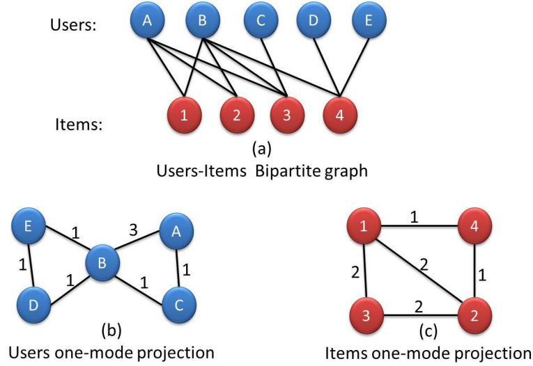
FIGURE 2.5 – (a) Exemple d'un graphe bipartit utilisateurs-items, (b) Graphe de collaboration entre utilisateurs, (c) graphe de projection sur les items (Sulieman et al. [129]).
