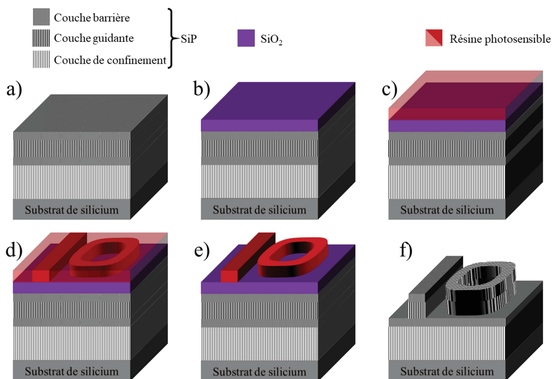
FIGURE 3.18 – Étapes de fabrication pour la réalisation d'un MR en quadricouche poreuses.
