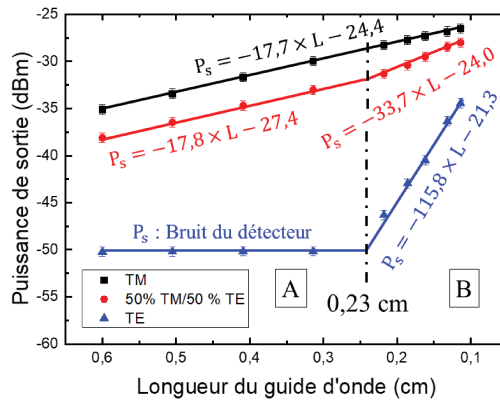
FIGURE 3.28 – Évolution de la puissance en sortie en fonction de la longueur des guides d'onde ridges rectilignes, pour trois configurations étudiées : TM, 50 % TM et 50 % TE et TE.
