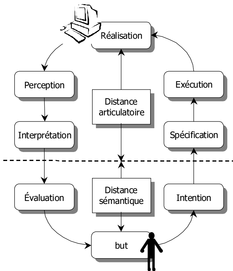
FIG. 1.2 – Distances sémantiques et distances articulatoires.
