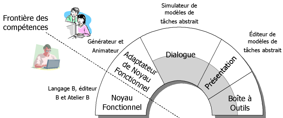
FIG. 3.9 – Conception « abstraite » du module Dialogue, Présentation et Boîte à outils de l'architecture ARCH.
