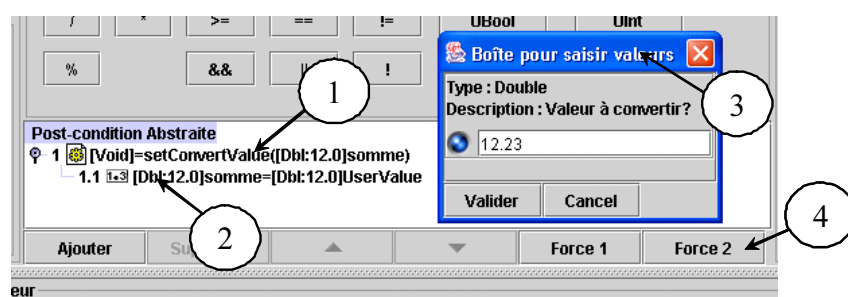
FIG. 3.15 – Exemple d'expressions pour l'action de la tâche interaction Saisir Valeur .
