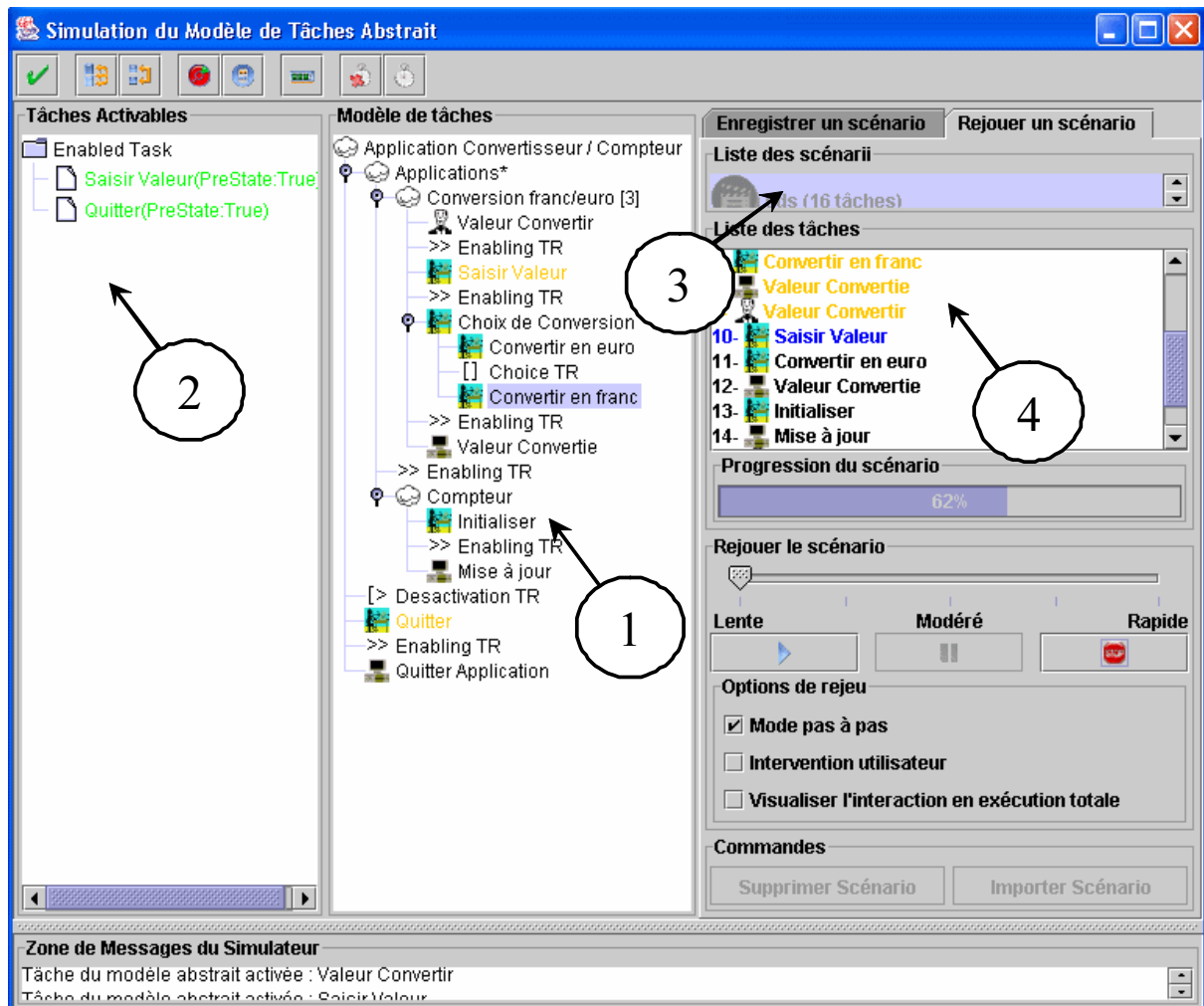
FIG. 3.18 – Capture d'écran de l'outil de simulation du modèle de tâches abstrait : Vue de la lecture d'un scénario.
