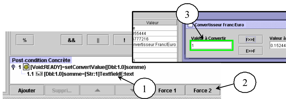
FIG. 3.25 – Expressions pour l'action de la tâche interaction concrète Zone Saisie .
