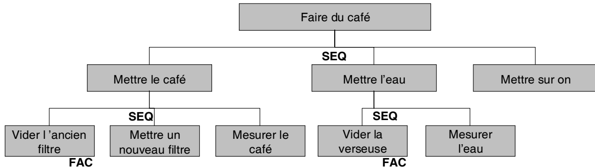
FIG. 1.6 – Faire du café , un exemple en notation MAD.
