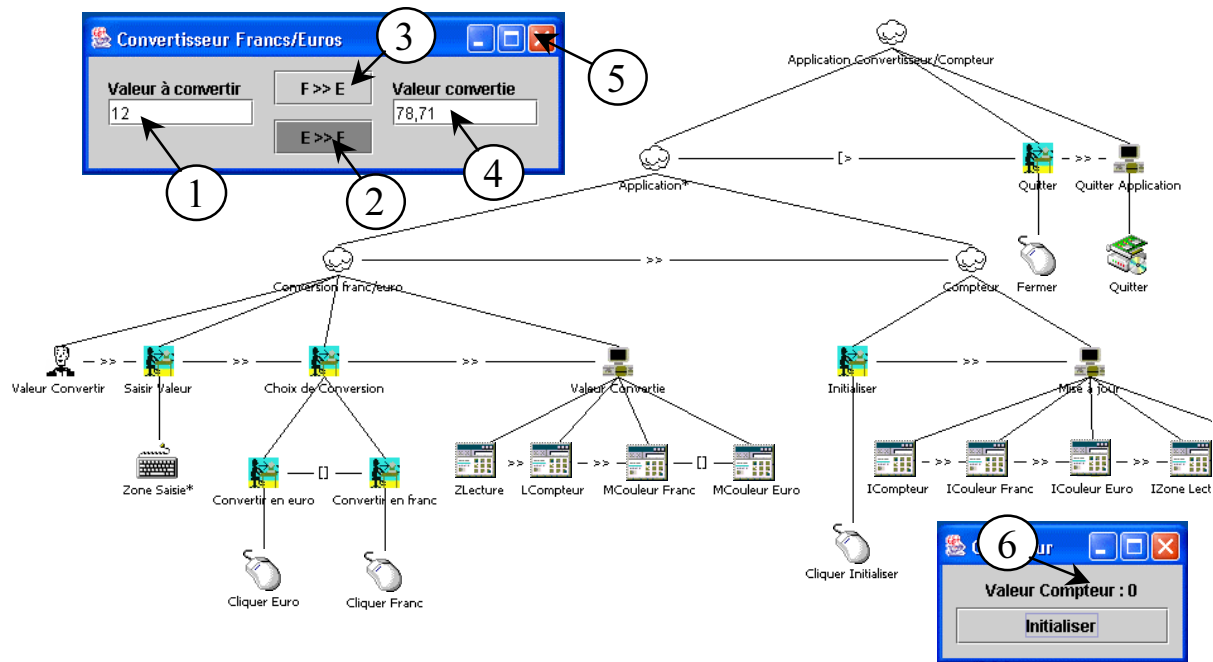
FIG. 3.21 – Extrait du modèle de tâches concret.
