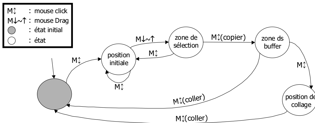
FIG. 1.12 – Copier/Coller une zone de texte, un exemple d'un système de transitions.
