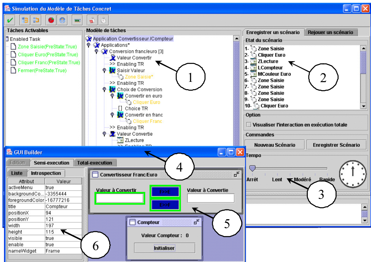
FIG. 3.27 – Capture d'écran de l'outil de simulation du modèle de tâches concret : vue de l'enregistrement d'un scénario.
