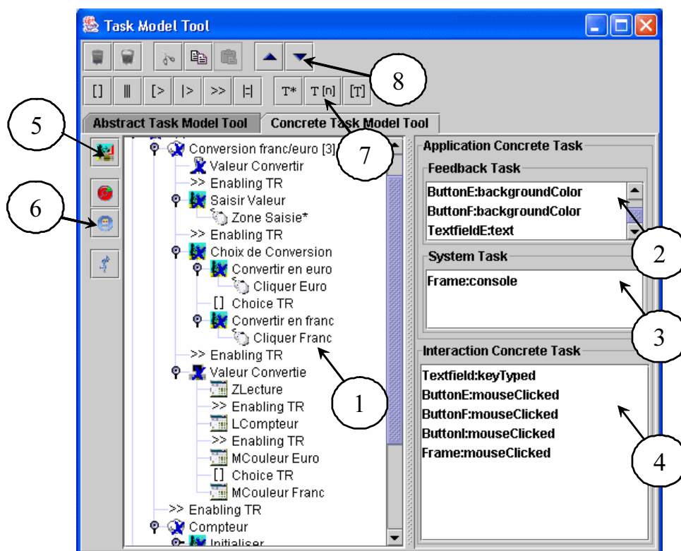
FIG. 3.23 – Capture d'écran de l'éditeur de modèle de tâches concret.
