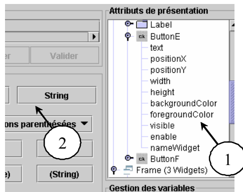
FIG. 3.24 – Capture d'écran des attributs de la présentation dans l'outil de liaison entre les objets du noyau fonctionnel et les tâches du modèle de tâches concret.
