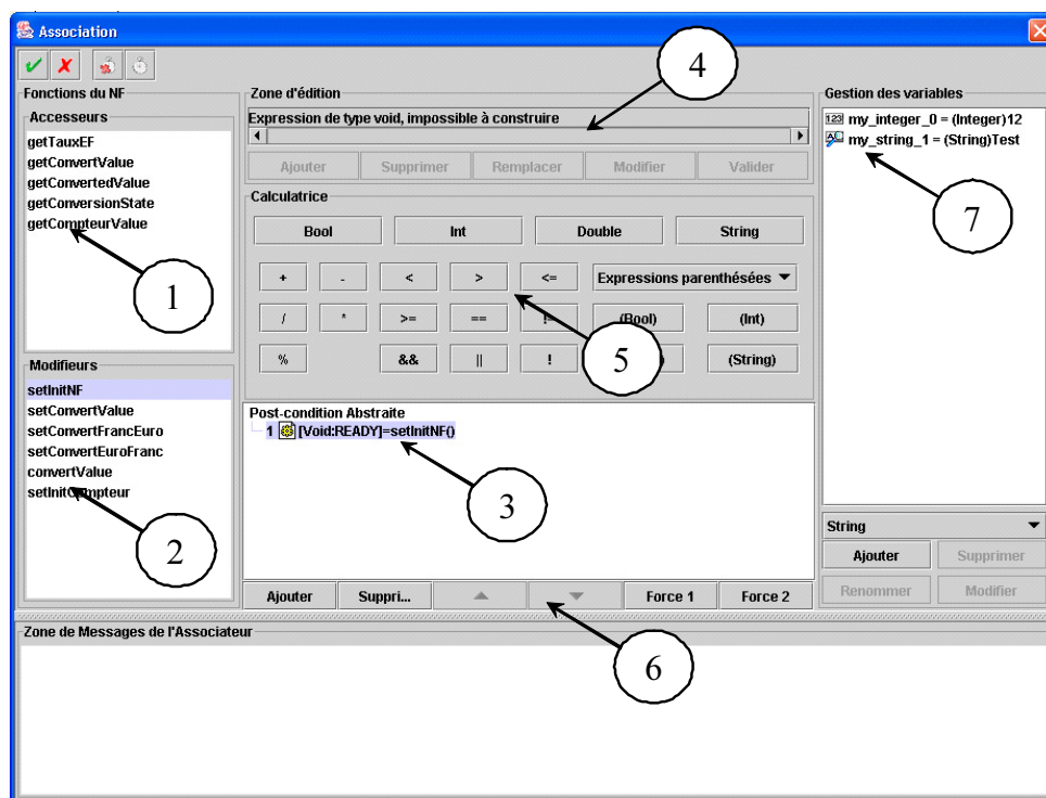
FIG. 3.13 – Capture d'écran de l'outil de liaison entre les objets du noyau fonctionnel et les tâches du modèle de tâches abstrait.
