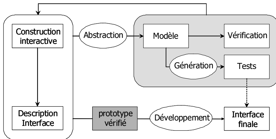
FIG. 1.20 – Approche à la fois expérimentale et formelle de [Roc98].
