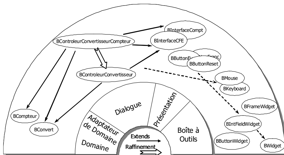
FIG. 2.14 – Décomposition en sous-systèmes convertisseur francs/euros et compteur.
