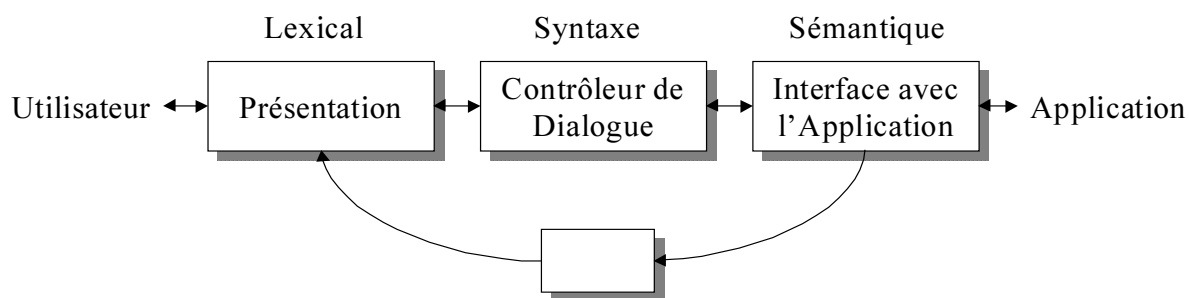
FIG. 1.8 – Le modèle SEEHEIM.
