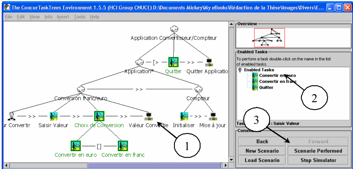
FIG. A.3 – Capture d'écran du simulateur de modèles de tâches CTT.
