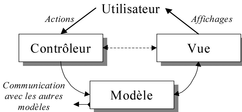
FIG. 1.10 – Le modèle MVC.
