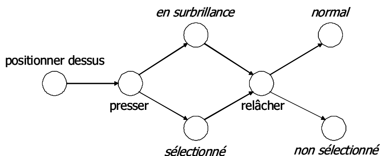
FIG. 1.18 – Comportement d'un bouton.
