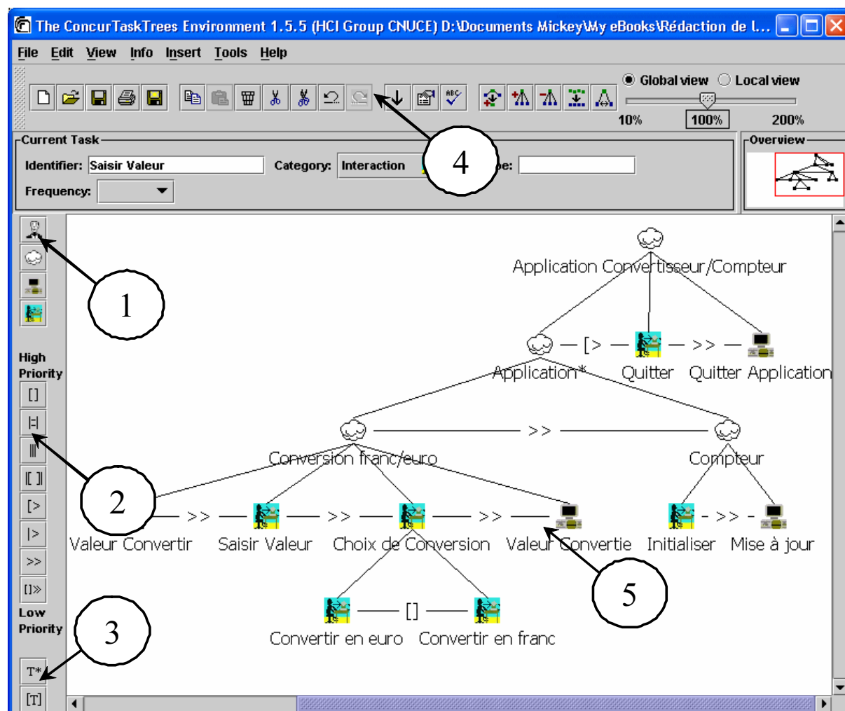
FIG. A.2 – Capture d'écran de l'éditeur de modèles de tâches CTT.
