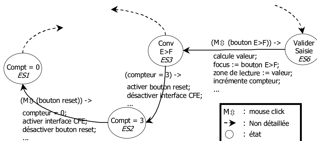
FIG. 2.13 – Extrait du système de transitions obtenu par la composition des systèmes de transitions du convertisseur et du compteur.
