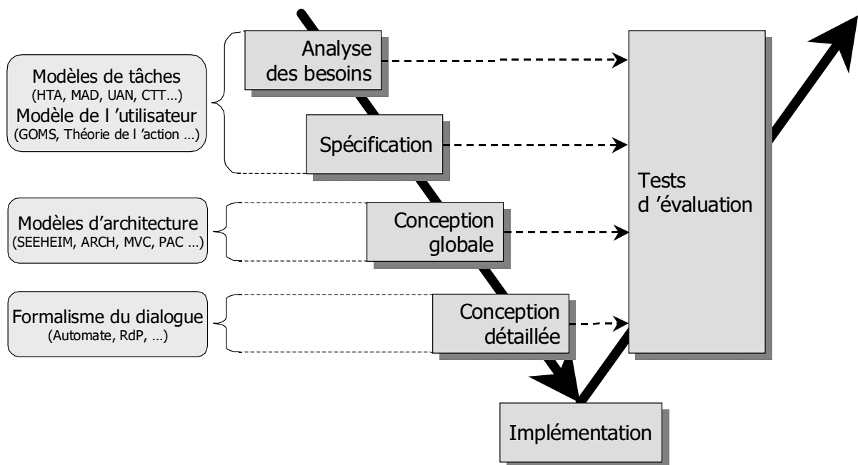
FIG. 1.4 – Modèles intervenant dans le cycle de développement en V pour les systèmes interactifs.
