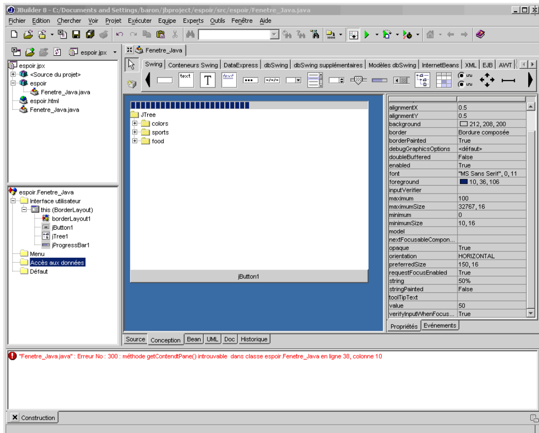
FIG. 1.24 – Exemple de GUI-Builder intégré dans l'environnement JBuilder.
