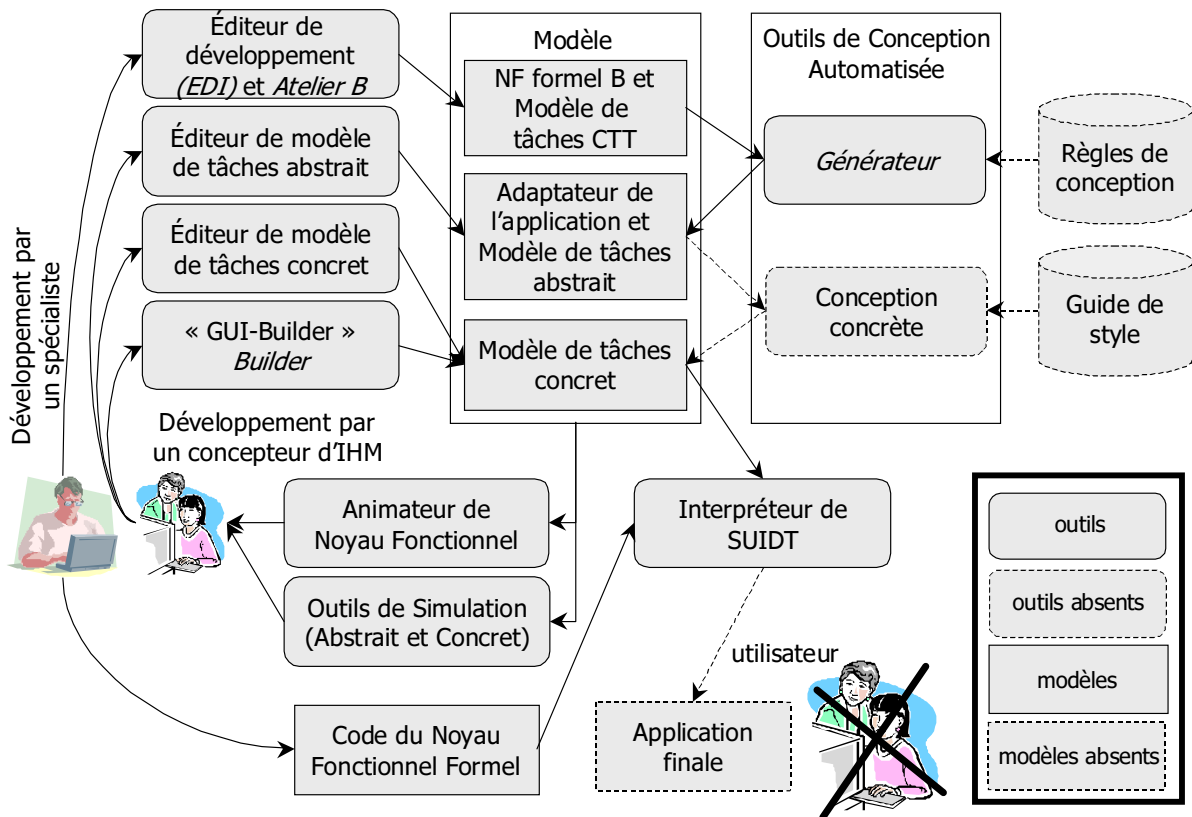
FIG. 3.28 – Architecture générique de l'environnement SUIDT.
