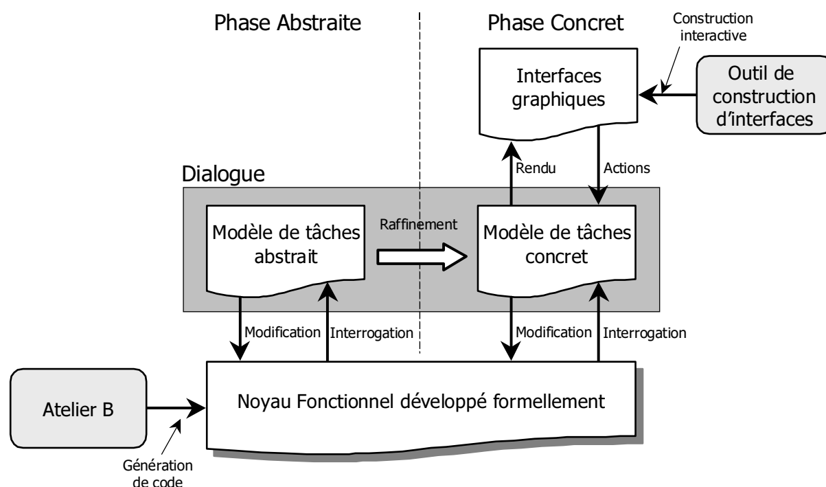
FIG. 3.3 – Description générale de l'approche SUIDT.
