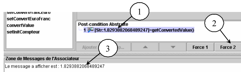
FIG. 3.16 – Exemple d’expressions pour l’action de la tâche application Valeur Convertie .
