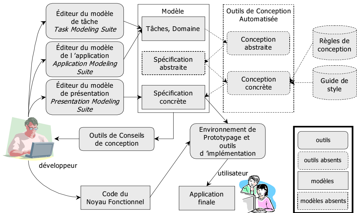
FIG. 1.29 – Architecture générique de l'environnement MASTERMIND.
