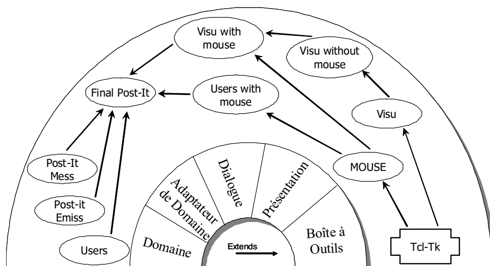
FIG. 2.3 – Relations entre machines abstraites B de la modélisation du Post-It Notes®.
