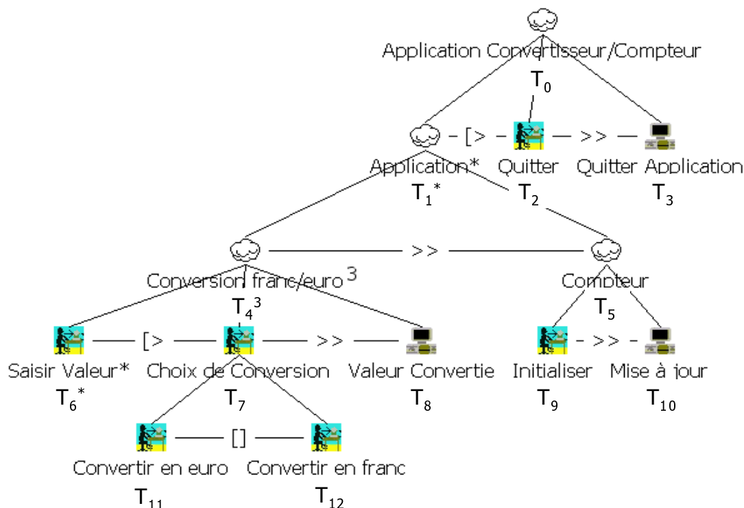
FIG. 2.16 – Modèle de tâches CTT de l'application convertisseur francs/euros et compteur.
