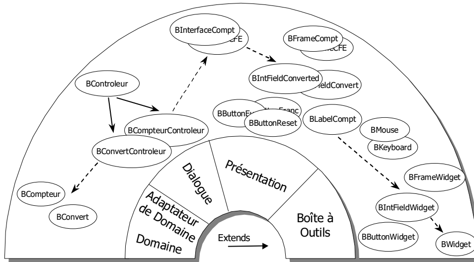
FIG. 2.5 – Composition modulaire ascendante des sous-systèmes convertisseur francs/euros compteur.
