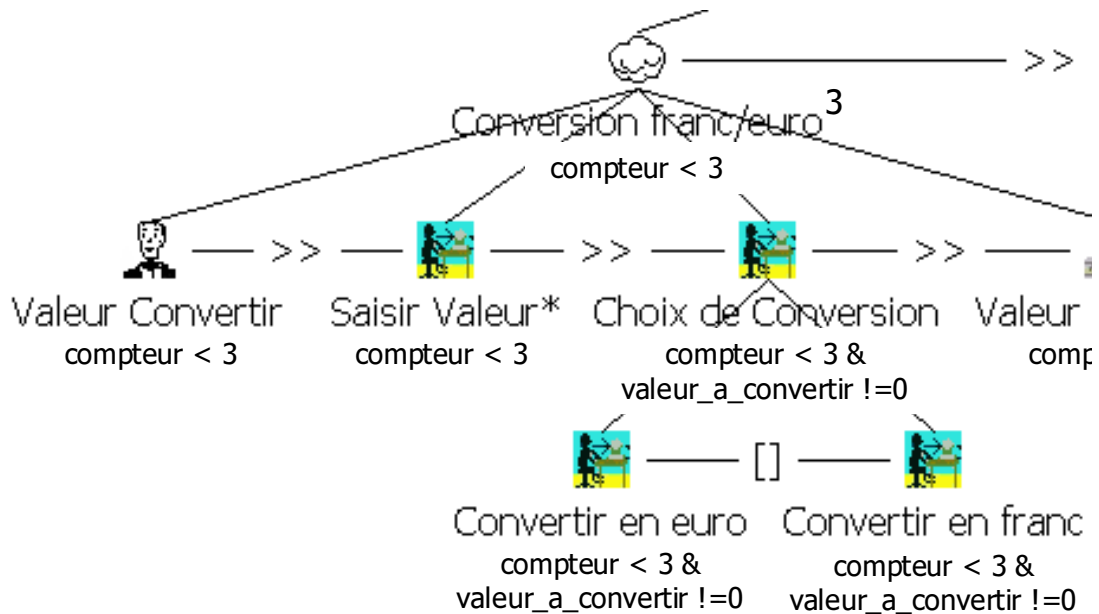
FIG. 3.10 – Exemple de préconditions (gardes) de tâches du modèle de tâches abstrait.
