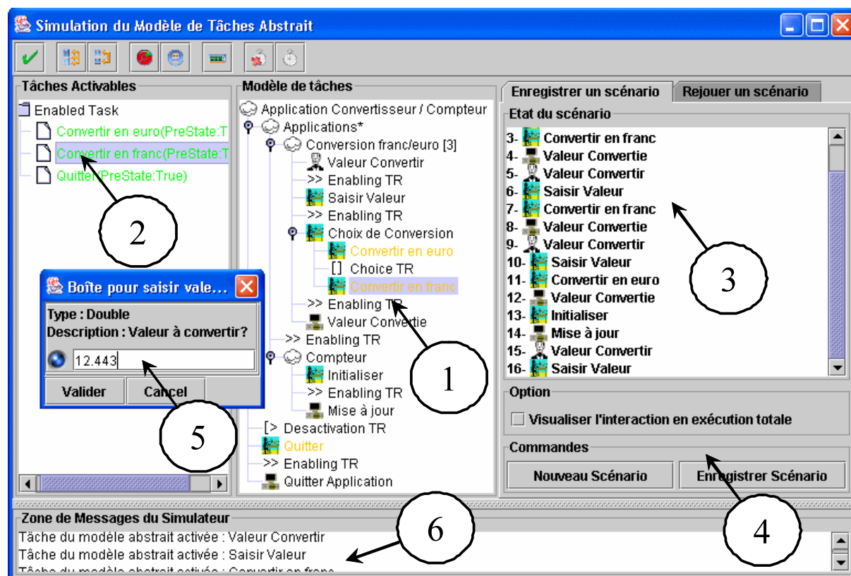
FIG. 3.17 – Capture d'écran de l'outil de simulation du modèle de tâches abstrait : Vue de l'enregistrement d'un scénario.
