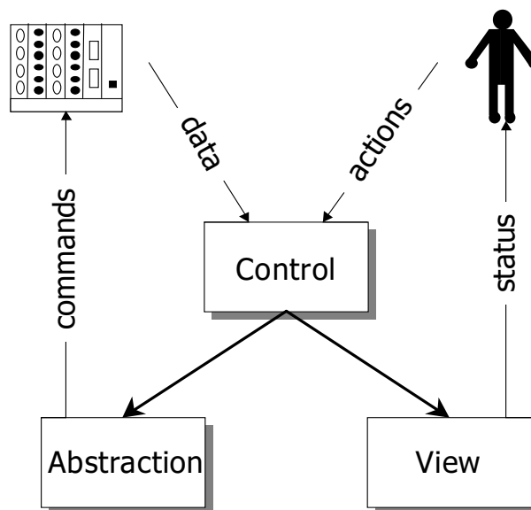
FIG. 1.21 – Le modèle d'architecture CAV Control-Abstraction-View .
