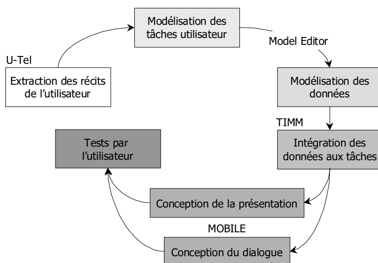
FIG. 1.26 – Cycle de développement dans MOBI-D.
