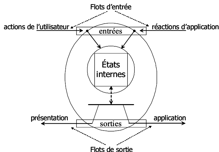
FIG. 1.19 – Interacteur à flots de données .
