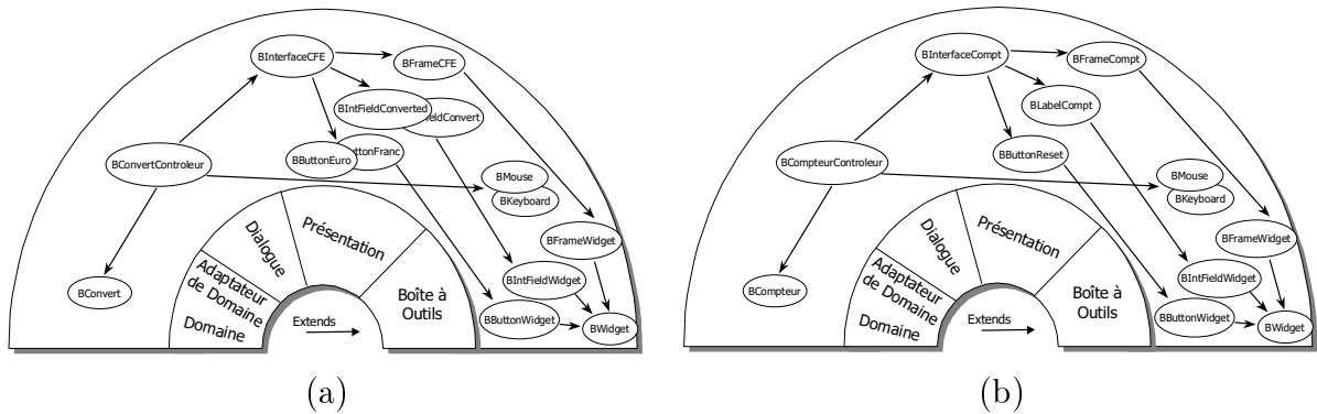
FIG. 2.4 – Relations entre machines abstraites B de la modélisation du convertisseur francs/euros (a) et du compteur (b).
