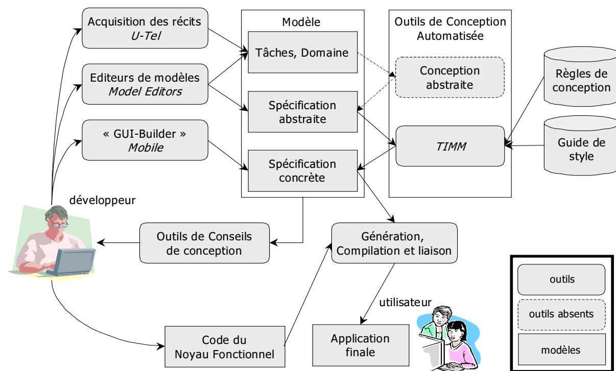
FIG. 1.27 – Architecture générique de l'environnement MOBI-D.
