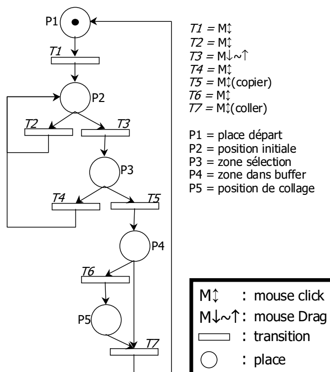
FIG. 1.13 – Copier/Coller une zone de texte, un exemple d'un réseau de Petri.
