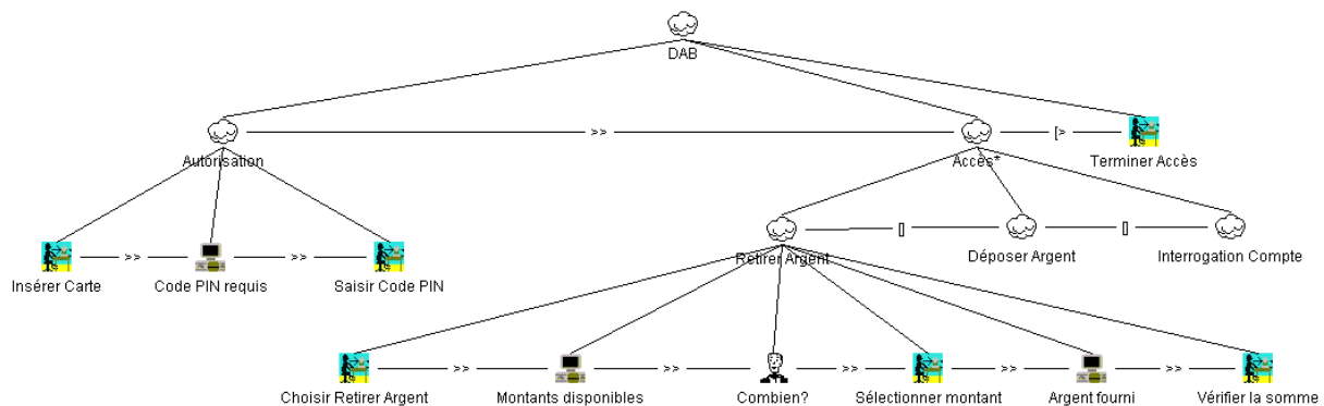
FIG. 1.7 – Distributeur automatique de billets , un exemple en notation CTT.
