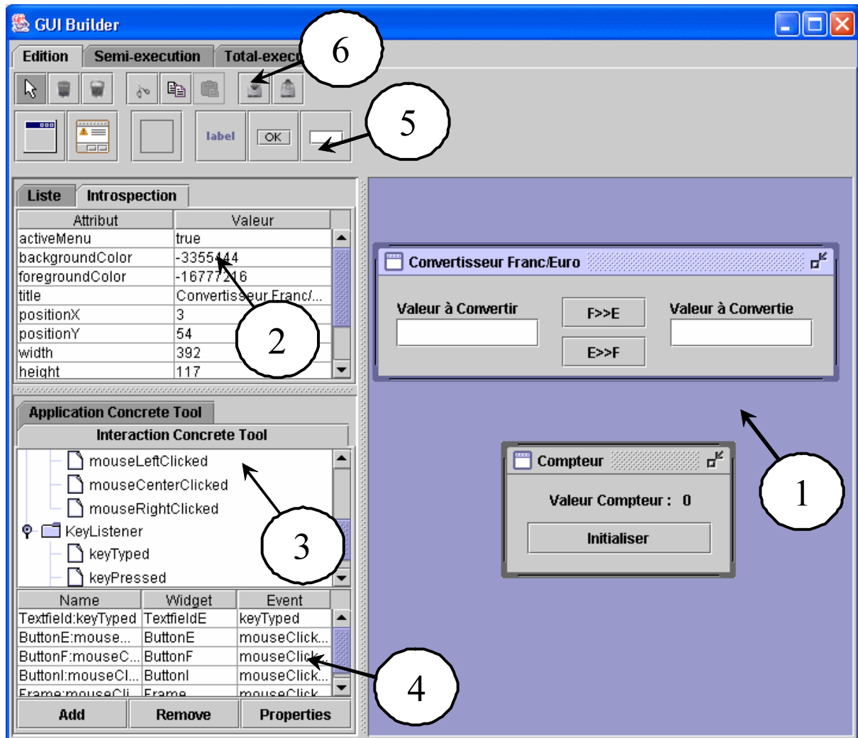
FIG. 3.22 – Capture d'écran de l'outil de construction d'interfaces utilisateur.
