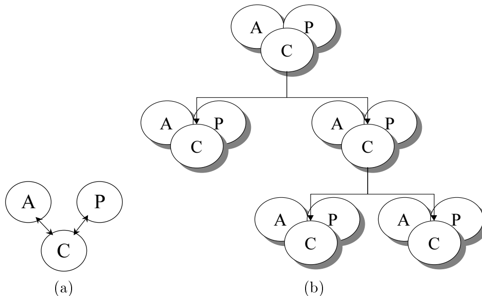
FIG. 1.11 – Agent PAC (a) et hiérarchie d'agent PAC (b).
