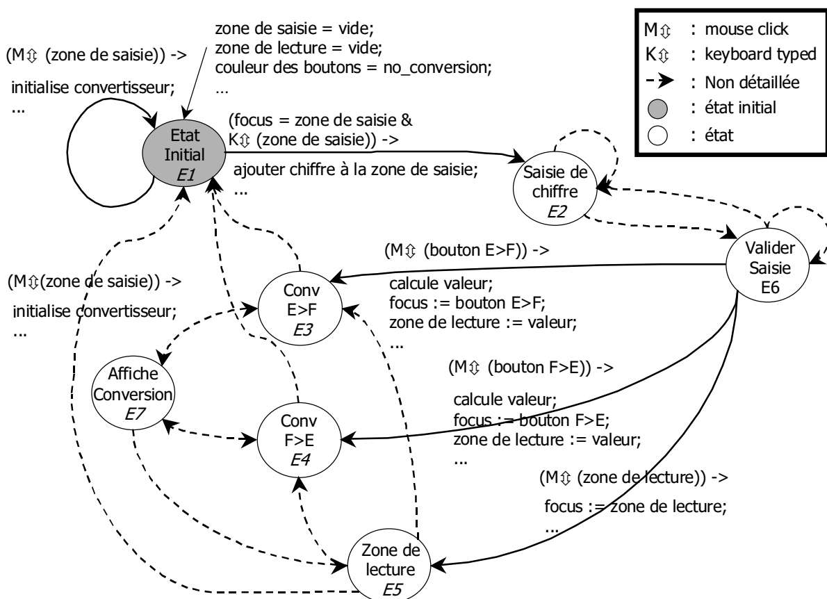
FIG. 2.10 – Système de transitions étiquetées du convertisseur francs/euros.
