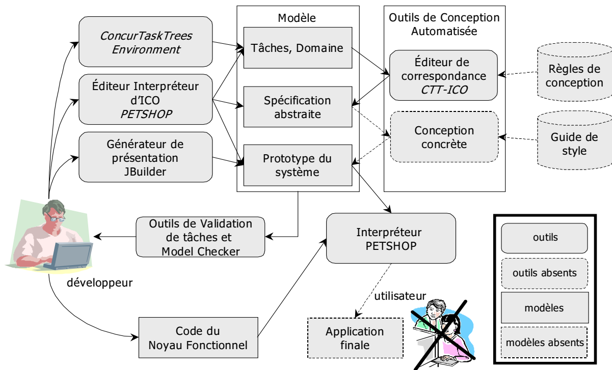
FIG. 1.32 – Architecture générique de l'environnement PETHOP.
