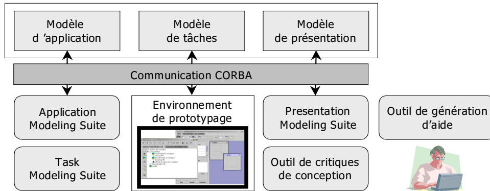
FIG. 1.28 – Rôle de la communication CORBA dans l’environnement MASTERMIND.
