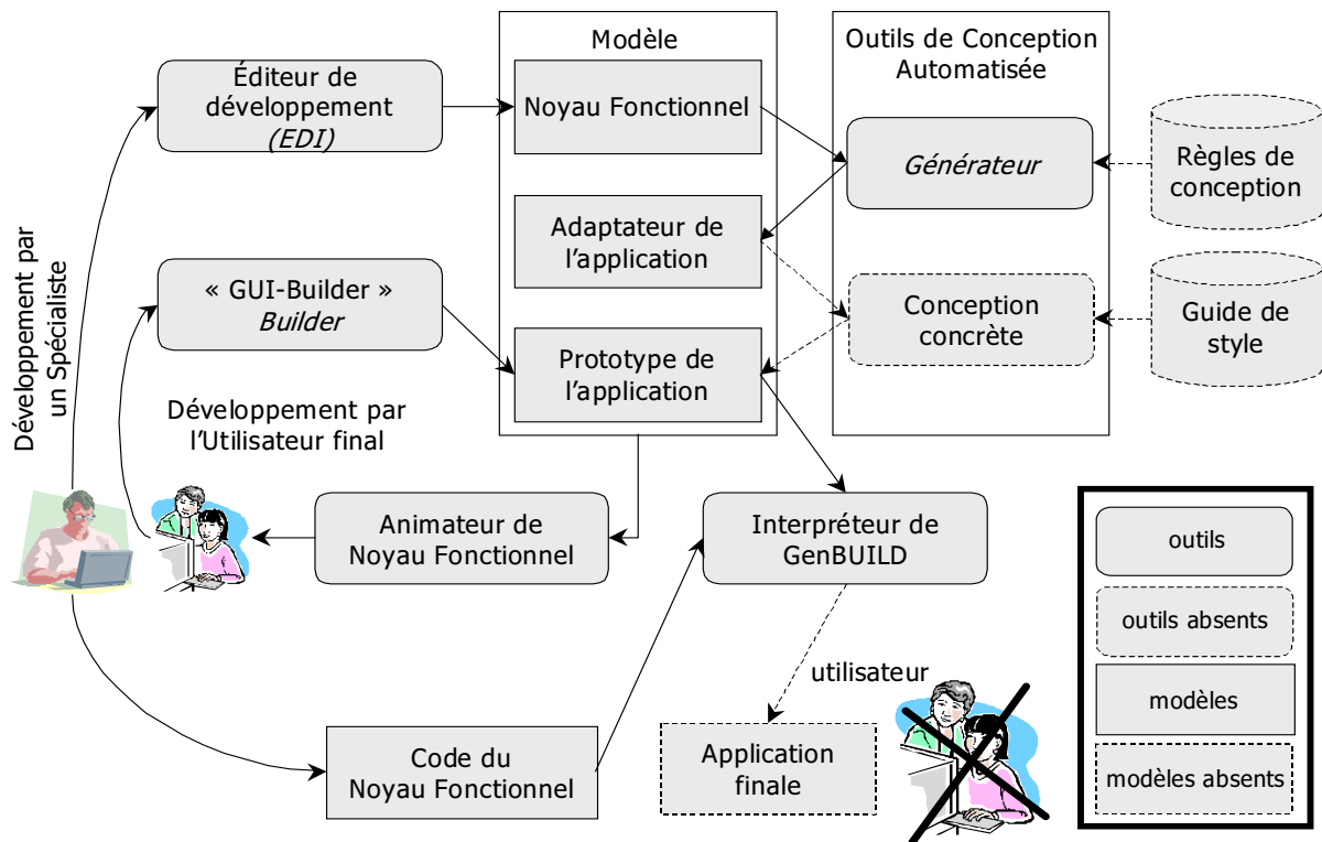
FIG. 3.2 – Architecture générique de l'environnement GenBUILD.
