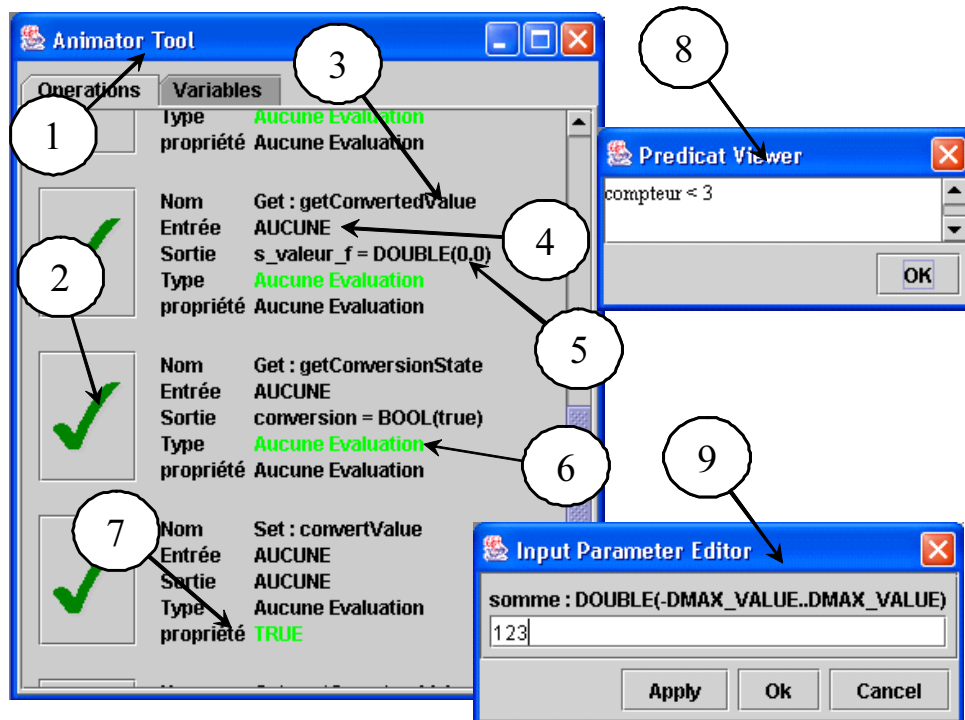
FIG. 3.7 – Capture d'écran de l'outil Animateur de noyau fonctionnel formel.
