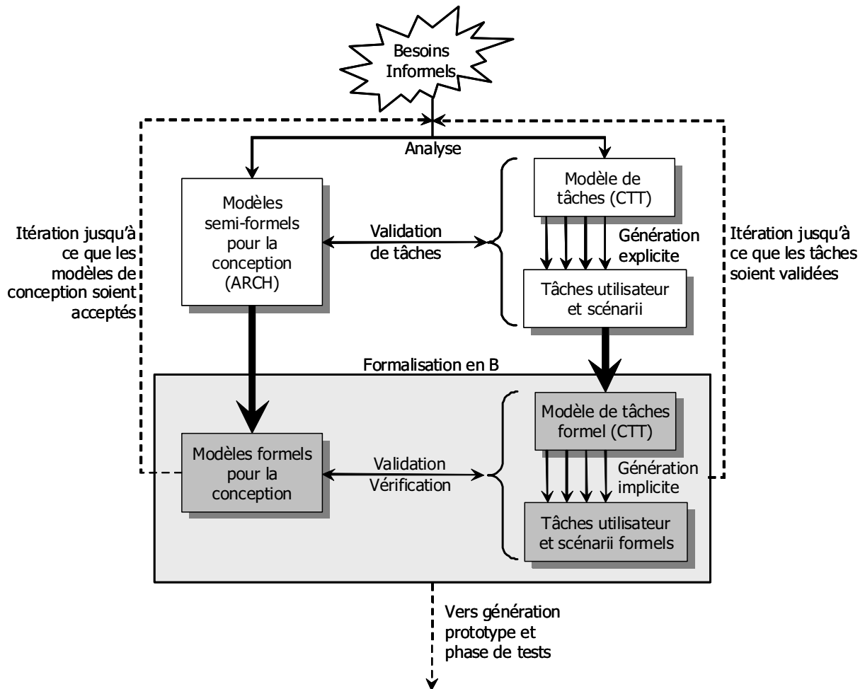
FIG. 2.15 – Description de l'approche implicite.
