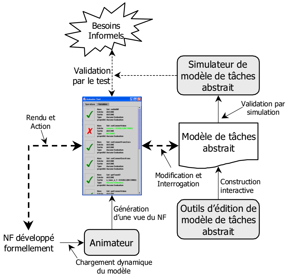
FIG. 3.8 – Démarche pour la modélisation du modèle de tâches abstrait.
