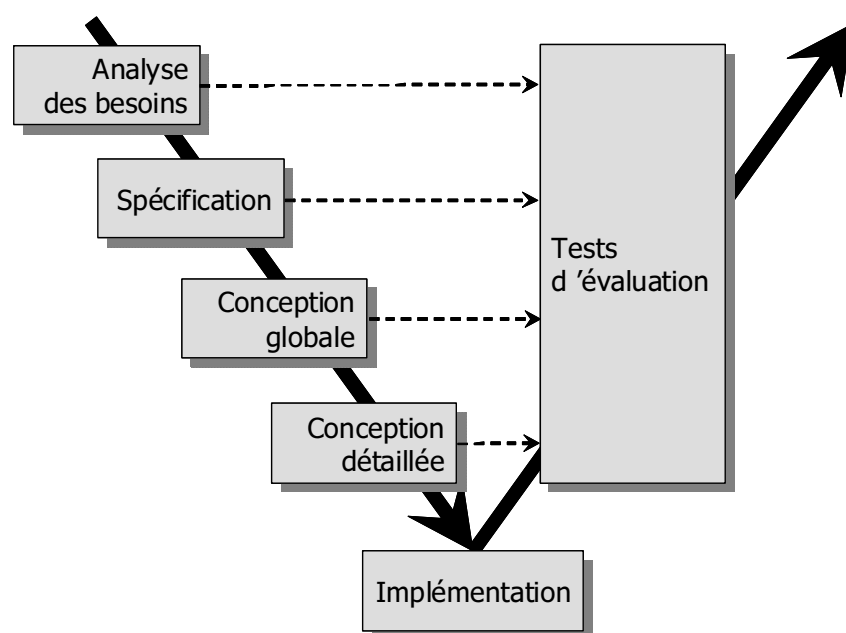
FIG. 1.3 – Modèle de développement en V pour les systèmes interactifs.
