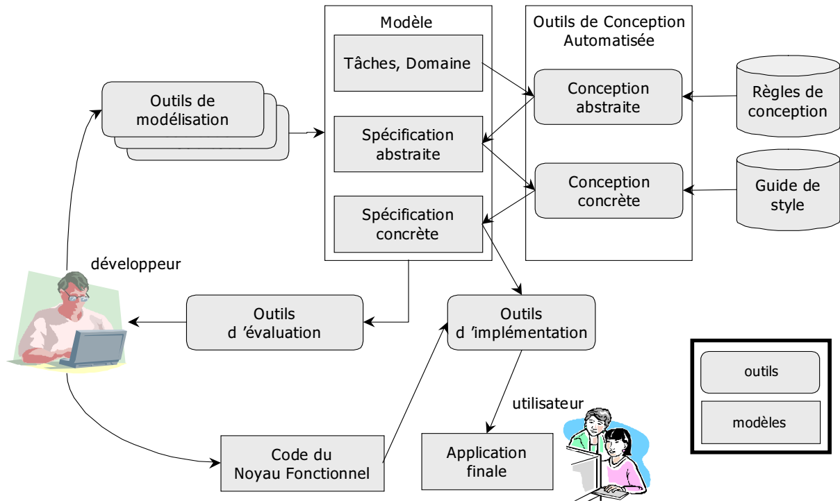
FIG. 1.25 – Environnement de développement d’interfaces à base de modèles, adapté de [Sze96].
