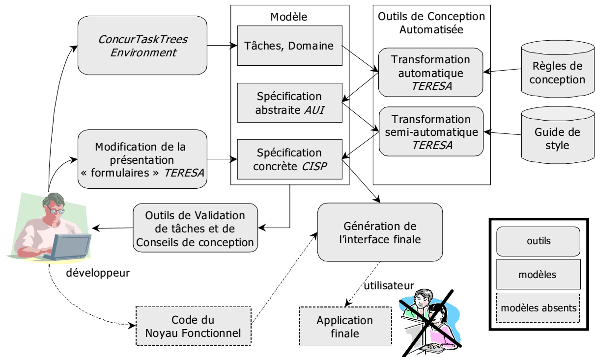
FIG. 1.30 – Architecture générique de l'environnement TERESA.
