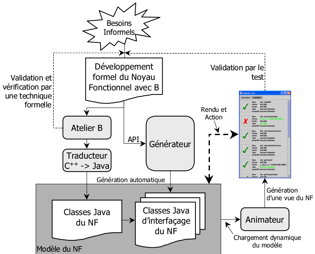
FIG. 3.4 – Démarche pour la prise en compte d'un noyau fonctionnel développé formellement
