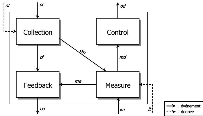
FIG. 1.15 – Boîte blanche de l'interacteur de CNUCE, adapté de [PF92].
