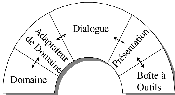
FIG. 1.9 – Le modèle ARCH.
