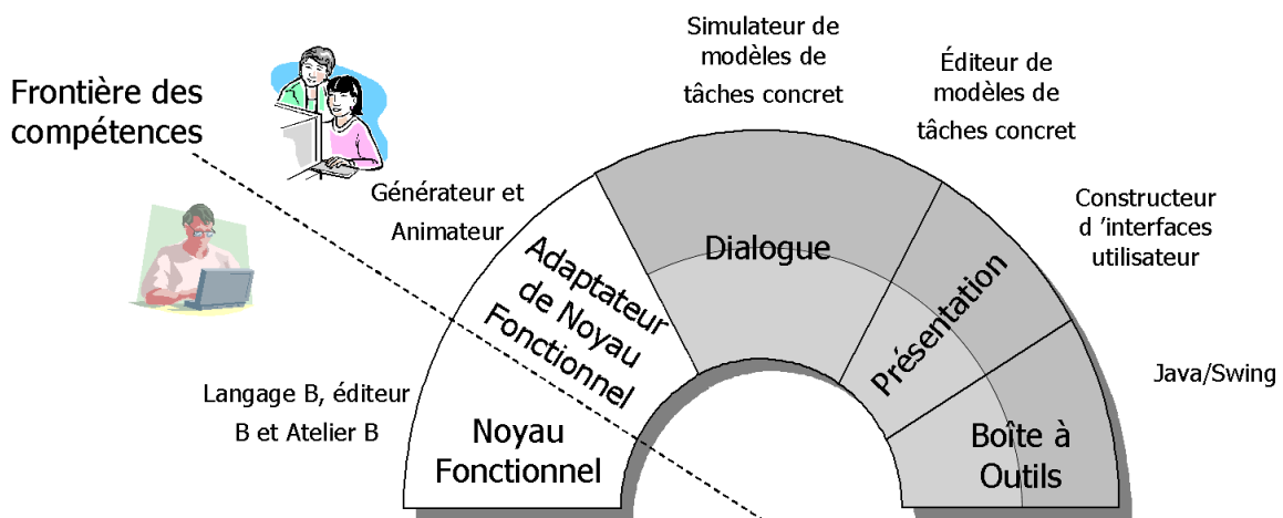
FIG. 3.20 – Concrétisation du module Dialogue, Présentation et Boîte à outils de l'architecture ARCH.
