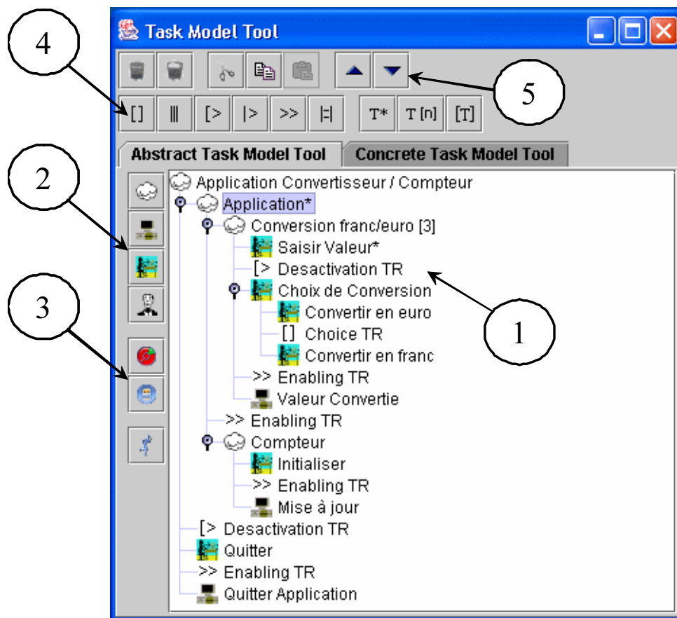
FIG. 3.12 – Capture d'écran de l'éditeur de modèle de tâches abstrait.
