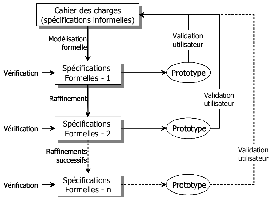
FIG. 1.14 – Processus de développement formel.
