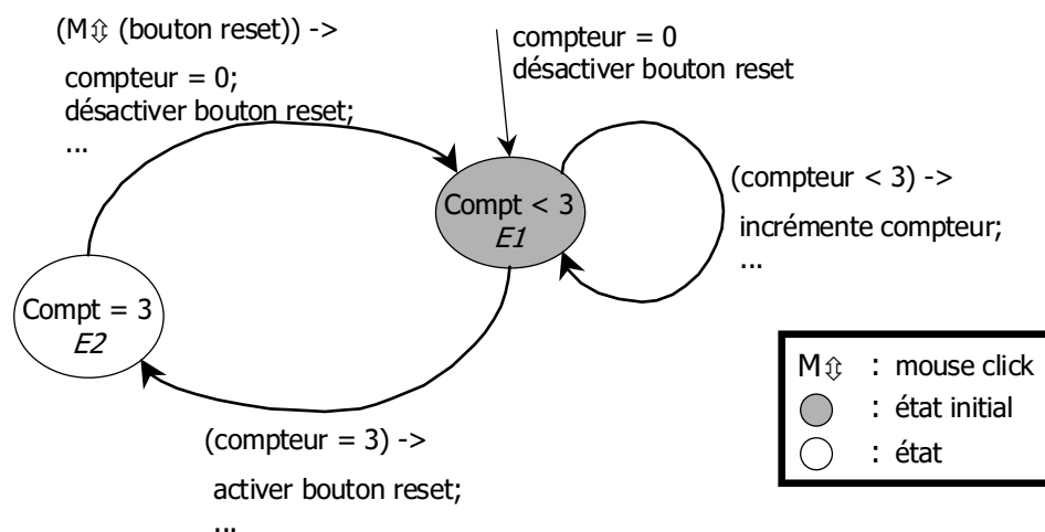
FIG. 2.11 – Système de transitions étiqueté du compteur.
