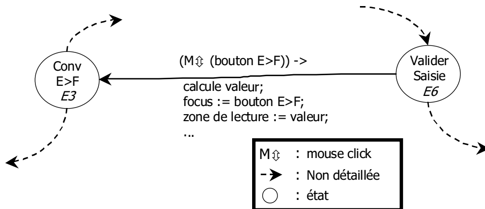
FIG. 2.12 – Transition de l'état E6 à E3 de l'automate du convertisseur francs/euros.
