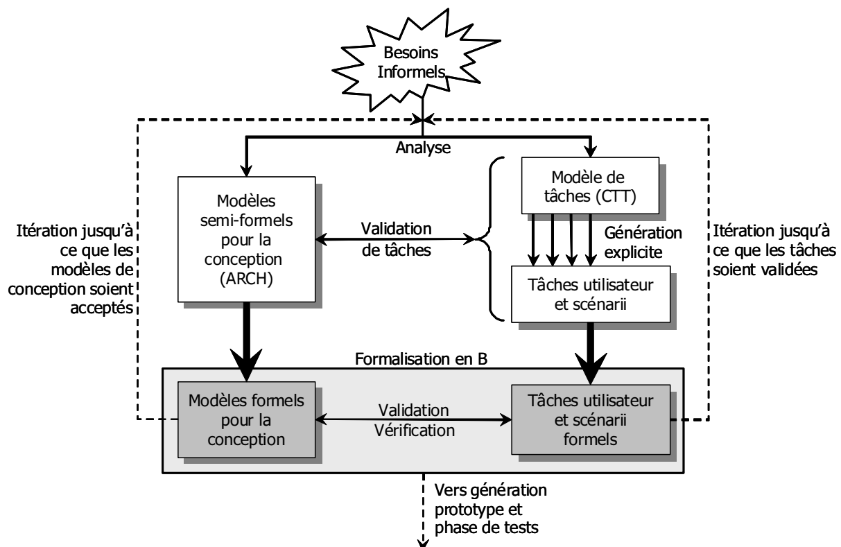
FIG. 2.6 – Description de l'approche explicite.
