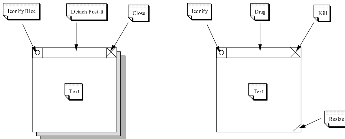
FIG. 2.2 – Interface de l'application Post-It Notes ® modélisée au moyen de la méthode B.
