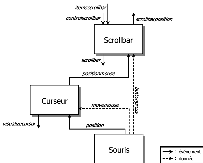
FIG. 1.16 – Modélisation d'un scrollbar, un exemple avec les interacteurs en boîte noire de CNUCE, adapté de [PF92].
