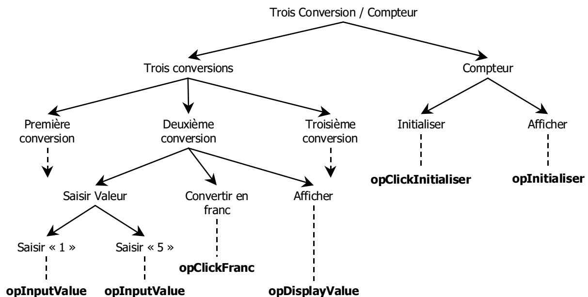
FIG. 2.8 – Décomposition en sous-tâches de la tâche Trois conversions / Compteur .
