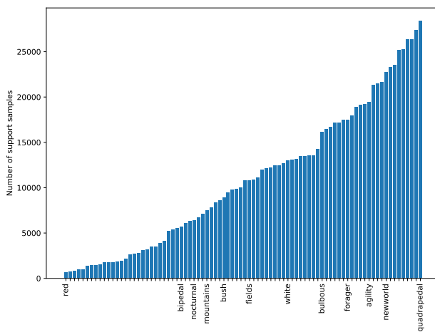
b) AwA2
