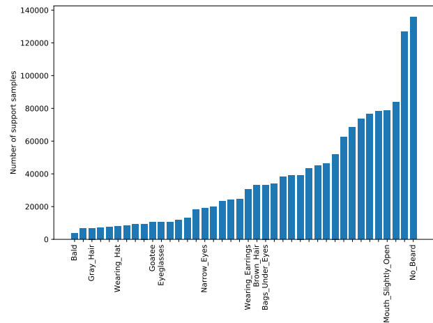
c) CelebA
