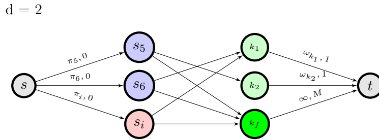
FIGURE 4.2 – Graphes de planification du service i pour les jours 1 et 2
