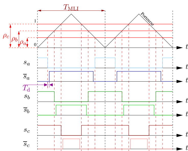
FIGURE 3.3 – PWM centrée avec temps mort T_d .
