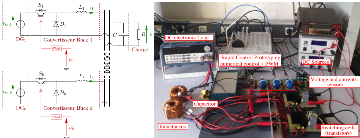
FIGURE 1.6 – Convertisseurs parallèles.
