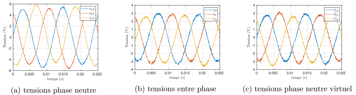
FIGURE A.5 – Représentation des mesure de FEMs du moteur BLDC faible coût.
