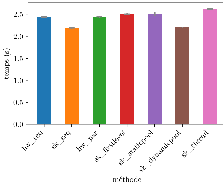
FIGURE 5.31 – Temps d’exécution séquentielle d’un \text{GRASP} \times \text{ELS} pour une instance de TSP de 38 sommets
