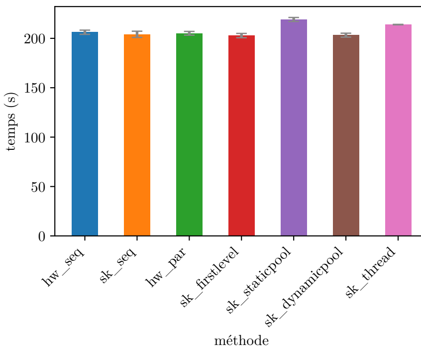
FIGURE 5.32 – Temps d’exécution séquentielle d’un \text{GRASP} \times \text{ELS} pour une instance de TSP de 194 sommets
