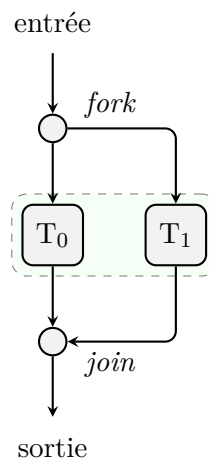
FIGURE 5.1 – Patron d'exécution parallèle fork-join
