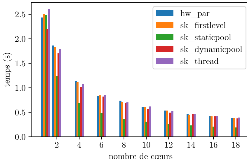
FIGURE 5.33 – Temps d'exécution parallèle d'un \text{GRASP} \times \text{ELS} pour une instance de \text{TSP} de 38 sommets
