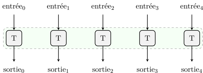
FIGURE 5.2 – Patron d'exécution parallèle map
