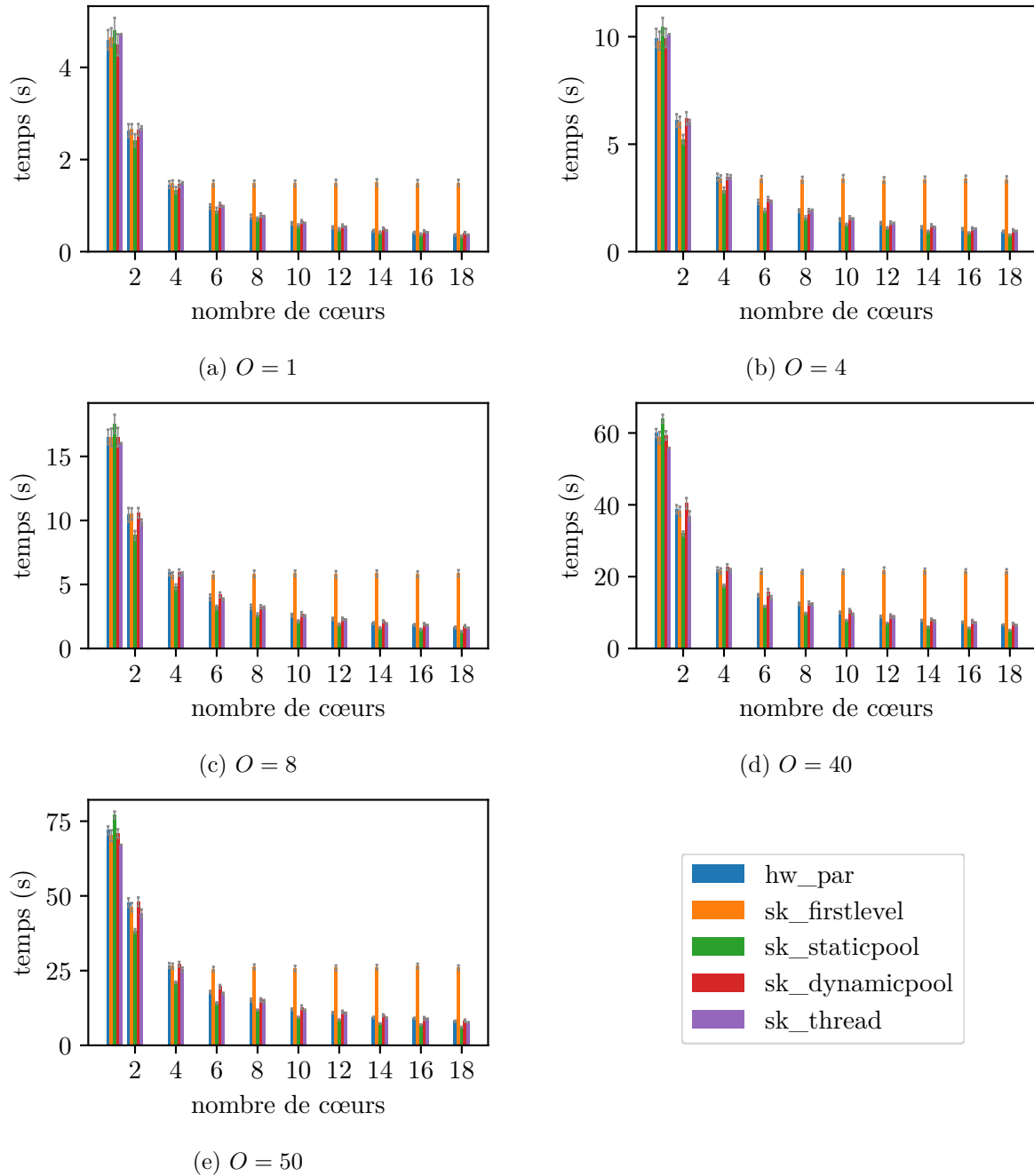
FIGURE 5.36 – Temps d'exécution parallèle d'un GRASP×ELS pour une instance de TSP de 194 sommets selon le nombre d'itérations non parallélisables de l'ELS
