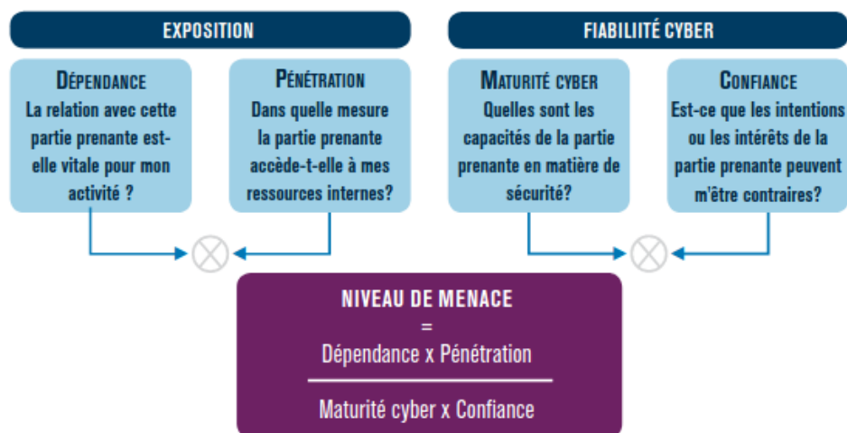
FIGURE II.11: Calcul du niveau de menace associé à une partie prenante [ANS19], sous licence Etalab
