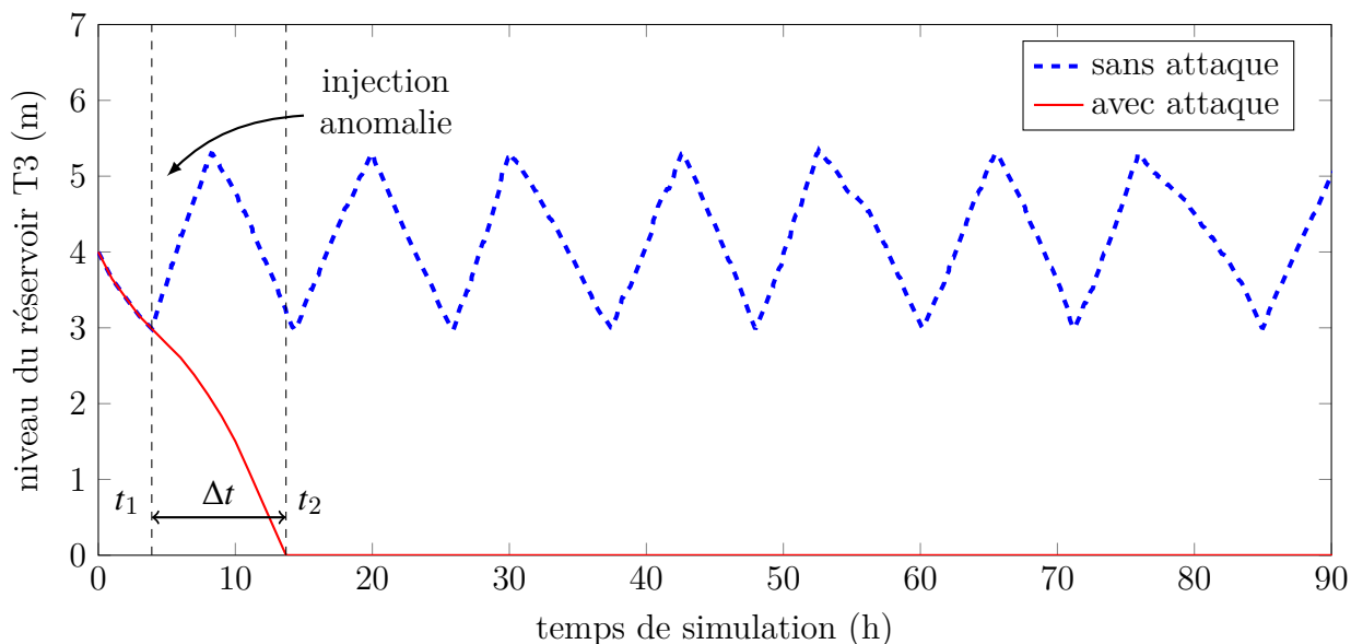
FIGURE III.19: Scénario 3, niveau du réservoir T3
