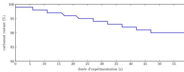
(c) Niveau l_{f_t} de carburant
