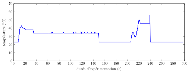
(a) Température t_m du moteur
