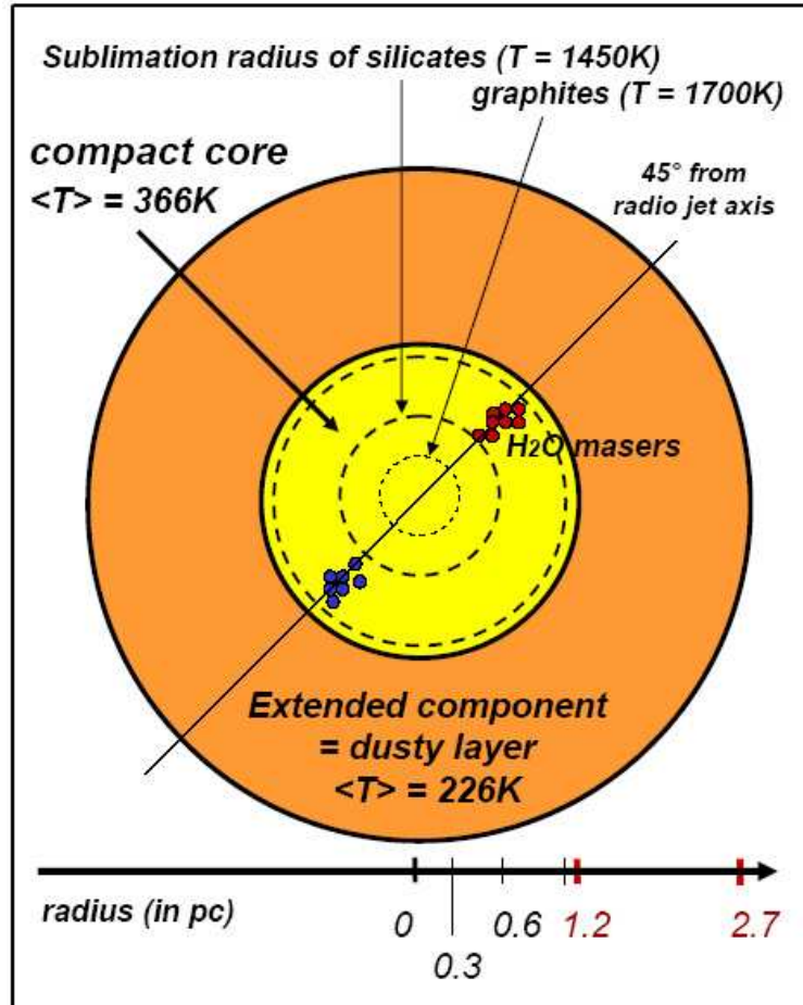
FIG. 5.3 – Schéma récapitulatif de la disposition des différentes composantes dans le coeur de NGC 1068. On y voit la couche de silicates déduite de la présente analyse des données MIDI ; la couche située juste à l’intérieur, potentiellement composée de graphites déduite des observations de Weigelt et al. (2004) et Gratadour et al. (2006) et constituant un environnement favorable à l’émission des masers H 2 O observées par Greenhill et al. (1996) et Greenhill et Gwinn (1997) ; les rayons de sublimations sont également représentés.
