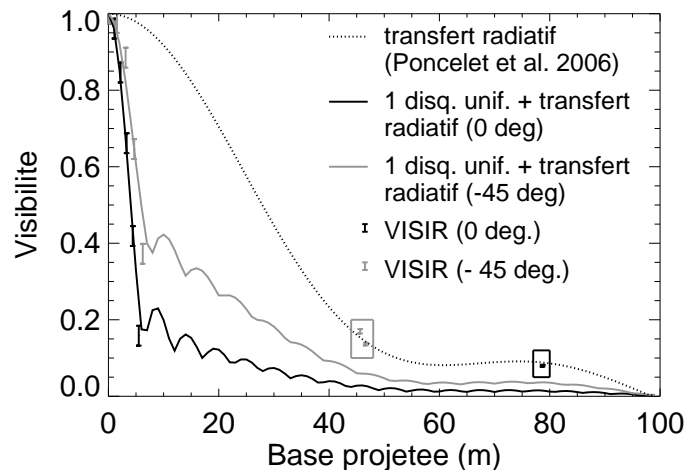
FIG. 8.2 – Comparaison entre les points de visibilité MIDI à 12,8 \mu\text{m} (ceux à 45 m sont repérés par le carré gris et celui à 78 m est repéré par le carré noir ) et les visibilités à faibles fréquences spatiales déduites des images mode BURST de VISIR (points entre 0 et 8 m ; en considérant le masque de MIDI et en traitant les images comme dans les conditions d'acquisition des données MIDI). Le modèle à deux disques uniformes ( courbes noire et grise ) doit être comparé au modèle de transfert radiatif appliqué aux données MIDI ( courbe en pointillés ; voir la Partie II de cette thèse). Pour tenter de rendre compte de la chute importante de la visibilité à faible fréquence spatiale, nous avons ajouté une composante étendue autour du tore de poussière. La figure montre qu'il n'est toutefois pas possible de reproduire ainsi simultanément les deux jeux de données. Un modèle plus complexe sera nécessaire pour y parvenir. Les tailles de la composante étendue sont \sim 600 mas et \sim 300 mas suivant les directions à \text{PA} = 0^\circ et \text{PA} = -45^\circ respectivement.
