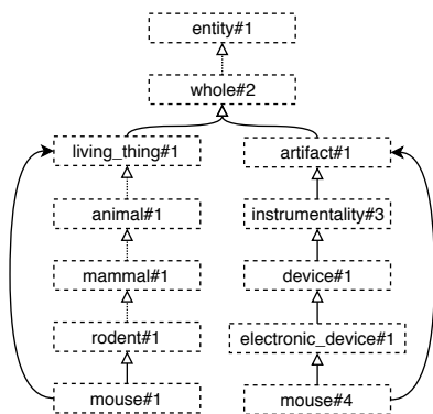
FIGURE 5.5 – Compression de vocabulaire utilisant la hiérarchie d’hyponymie, appliquée au premier et quatrième sens du mot ‘mouse’. Les lignes en pointillés indiquent que des nœuds ont été omis pour la clarté (issue de (Vial et al., 2019b)).
