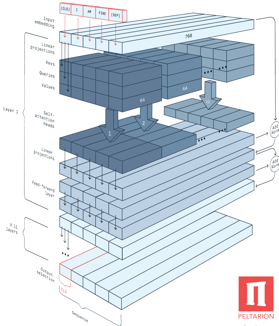
FIGURE 4.8 – Vue simplifiée de l'architecture de BERT BASE . La figure ne présente qu'une des 12 couches identiques. Les vecteurs sont de taille 768, il y a 12 têtes d'attention soit un total de 110 millions de paramètres – image issue de https://peltarion.com/knowledge-center/documentation/modeling-view/build-an-ai-model/blocks/english-bert .
