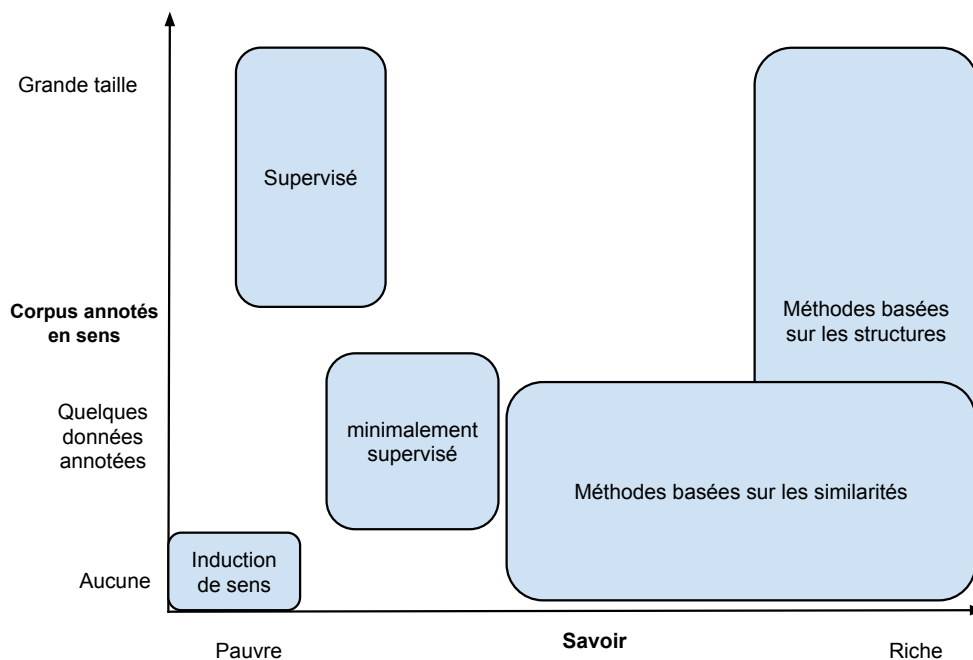
FIGURE 5.2 – Les différentes méthodes de désambiguïisation lexicale
