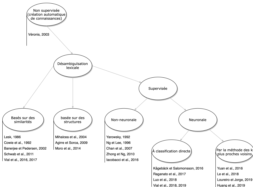
FIGURE 5.3 – Quelques-unes des différentes approches de la désambiguïation lexicale. Nous nous restreignons ici à celles que nous avons plus particulièrement étudiées au cours de nos recherches. Les approches non supervisées sont situées un peu au dessus, car la plupart des méthodes de désambiguïation lexicale sont utilisables une fois la ressource générique constituée.
